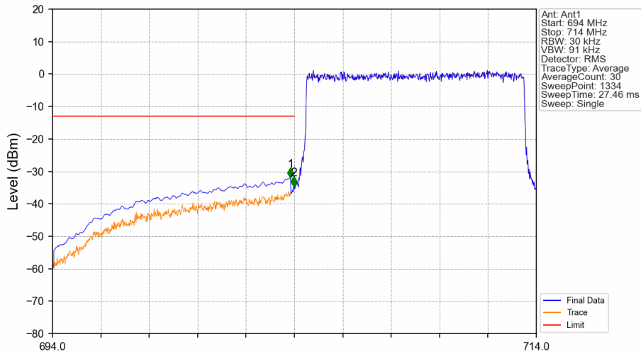
Band17_10MHz_QPSK_LCH_709MHz_RB_50_0_NTNV
