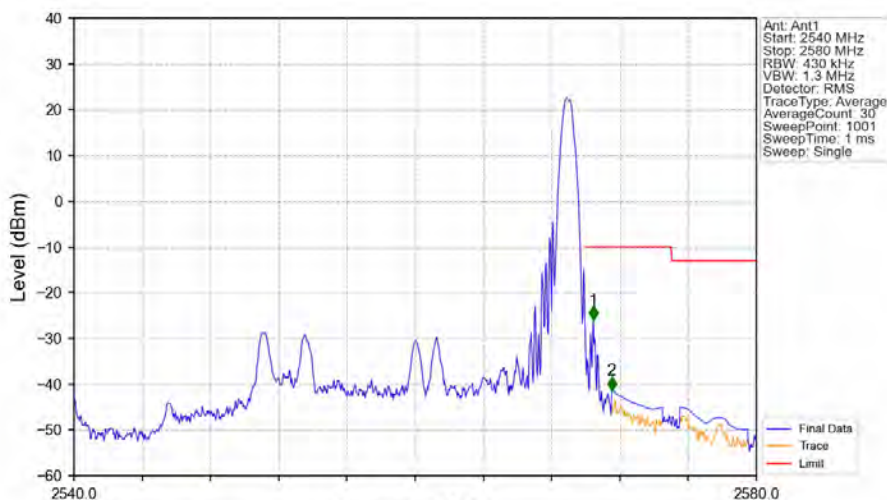
Band7_20MHz_QPSK_HCH_2560MHz_RB_1_99_NTNV
