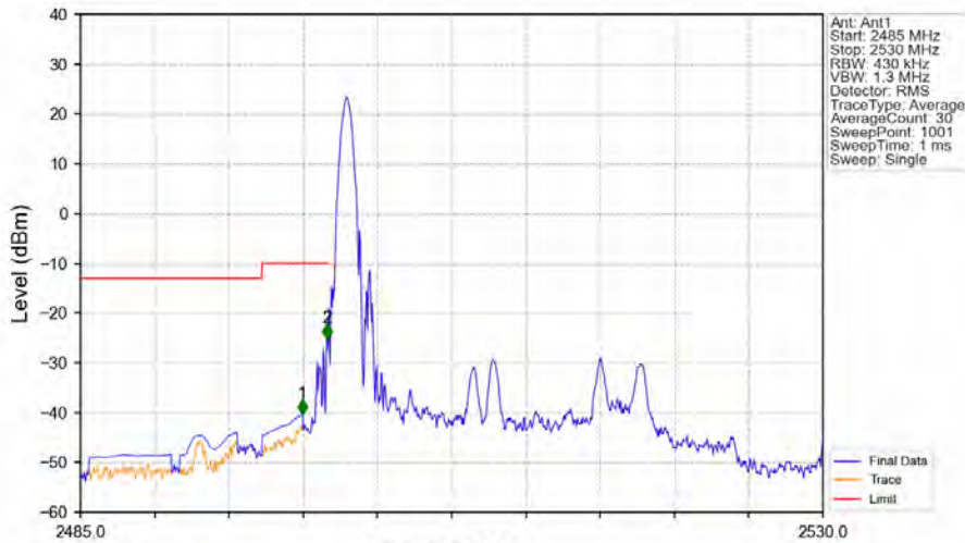
Band7_20MHz_16QAM_LCH_2510MHz_RB_1_0_NTNV
