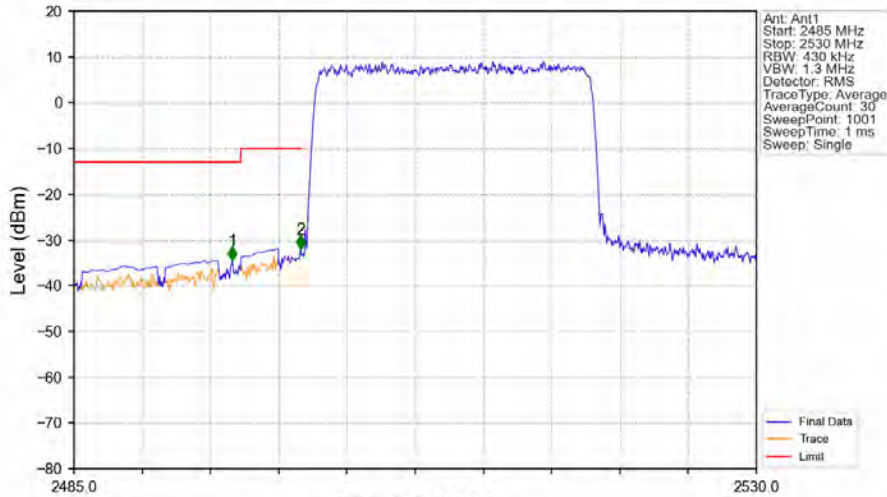
Band7_20MHz_QPSK_LCH_2510MHz_RB_100_0_NTNV
