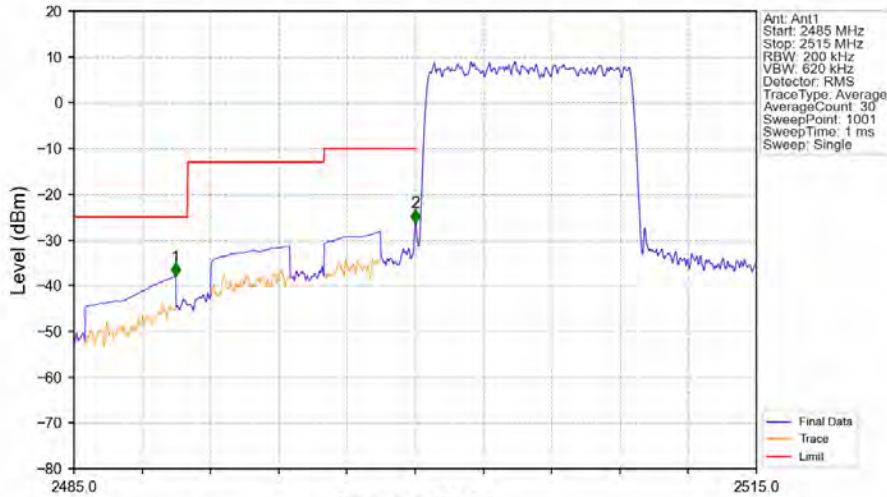
Band7_10MHz_QPSK_LCH_2505MHz_RB_50_0_NTNV
