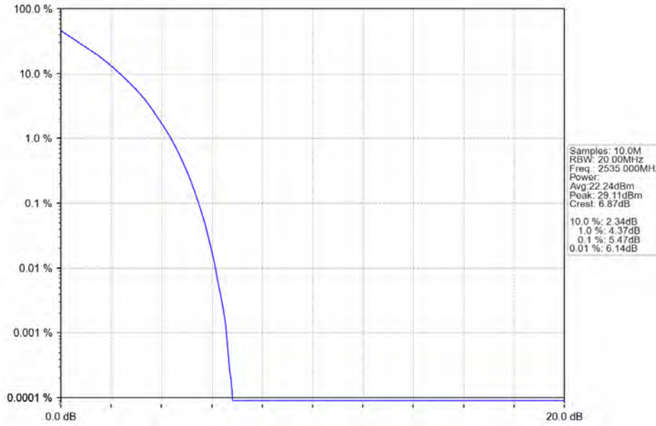
Band7_20MHz_QPSK_MCH_2535MHz_RB_100_0_NTNV
