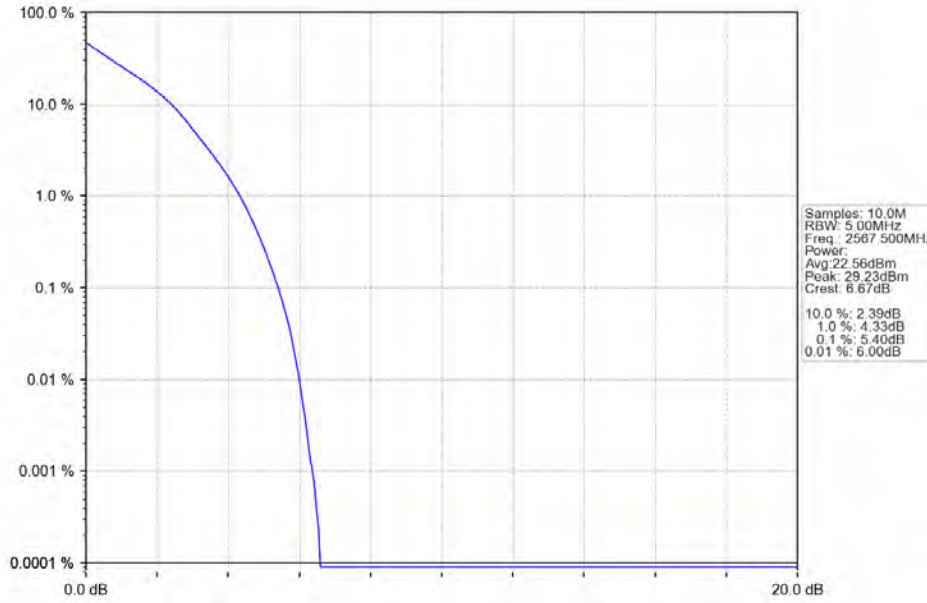
Band7_5MHz_QPSK_HCH_2567.5MHz_RB_25_0_NTNV
