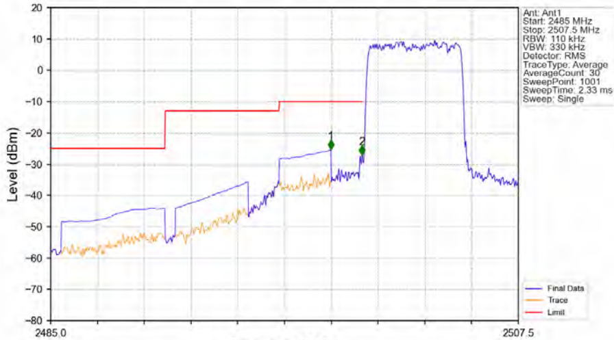
Band7_5MHz_QPSK_LCH_2502.5MHz_RB_25_0_NTNV
