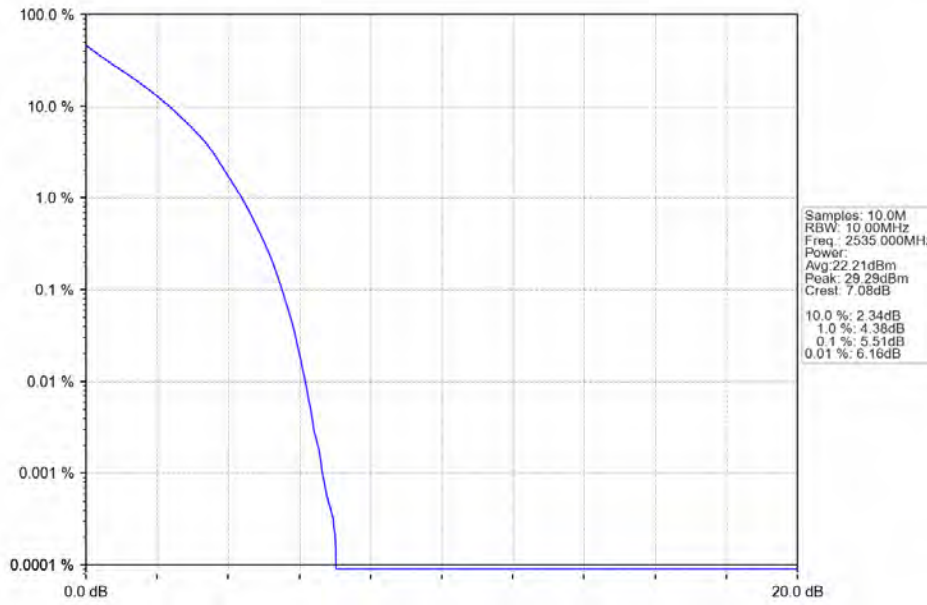
Band7_10MHz_QPSK_MCH_2535MHz_RB_50_0_NTNV
