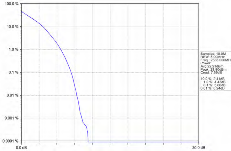
Band7_5MHz_QPSK_MCH_2535MHz_RB_25_0_NTNV
