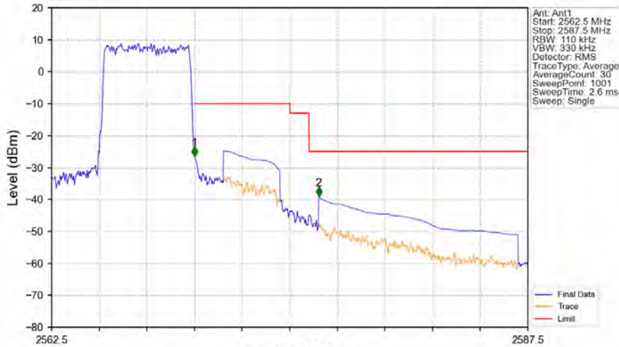
Band7_5MHz_QPSK_HCH_2567.5MHz_RB_25_0_NTNV
