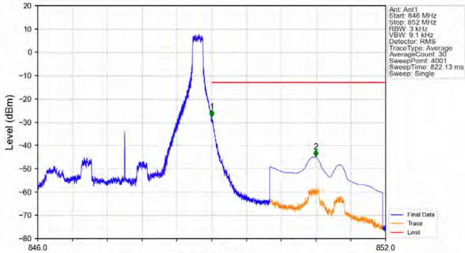
Band5_3MHz_QPSK_HCH_847.5MHz_RB_1_14_NTNV
