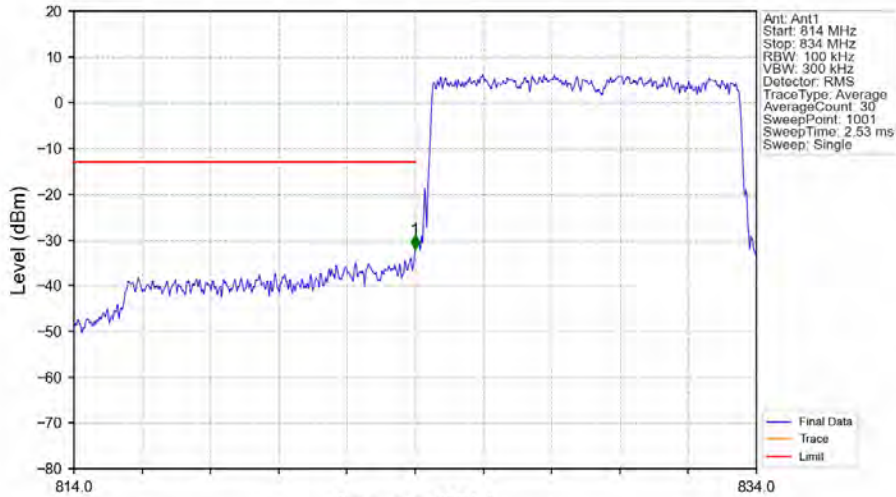
Band5_10MHz_QPSK_LCH_829MHz_RB_50_0_NTNV
