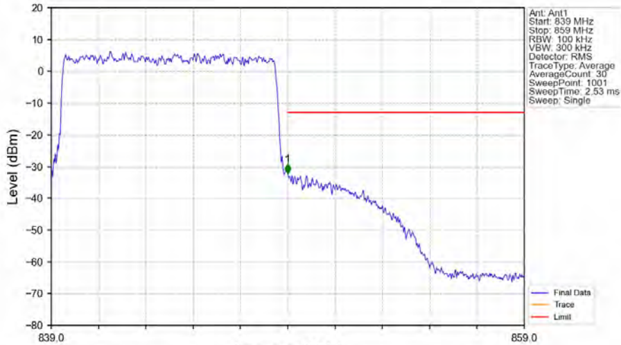
Band5_10MHz_QPSK_HCH_844MHz_RB_50_0_NTNV
