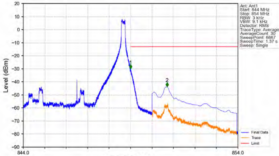
Band5_5MHz_QPSK_HCH_846.5MHz_RB_1_24_NTNV
