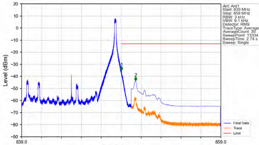
Band5_10MHz_QPSK_HCH_844MHz_RB_1_49_NTNV
