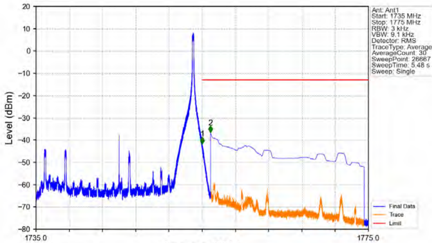
Band4_20MHz_QPSK_HCH_1745MHz_RB_1_99_NTNV
