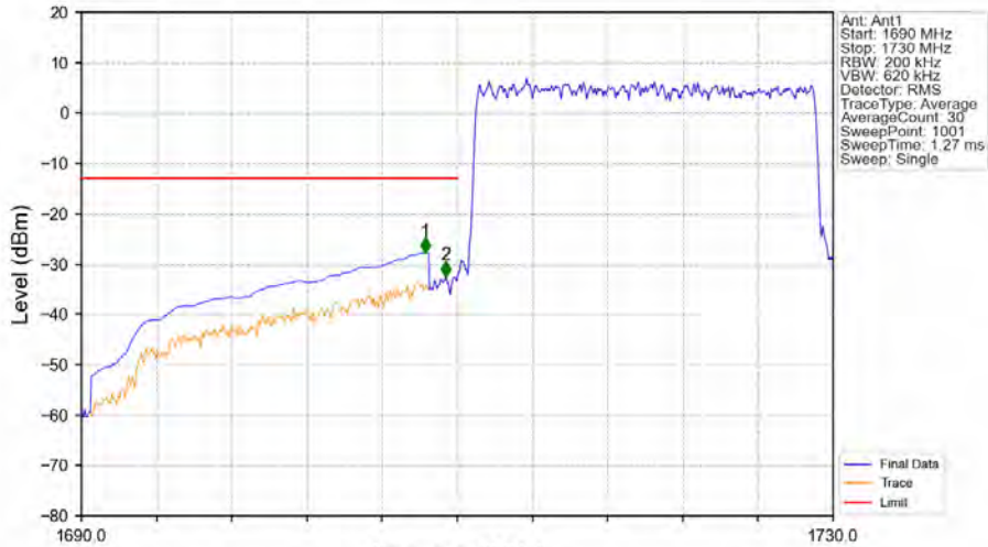
Band4_20MHz_QPSK_LCH_1720MHz_RB_100_0_NTNV
