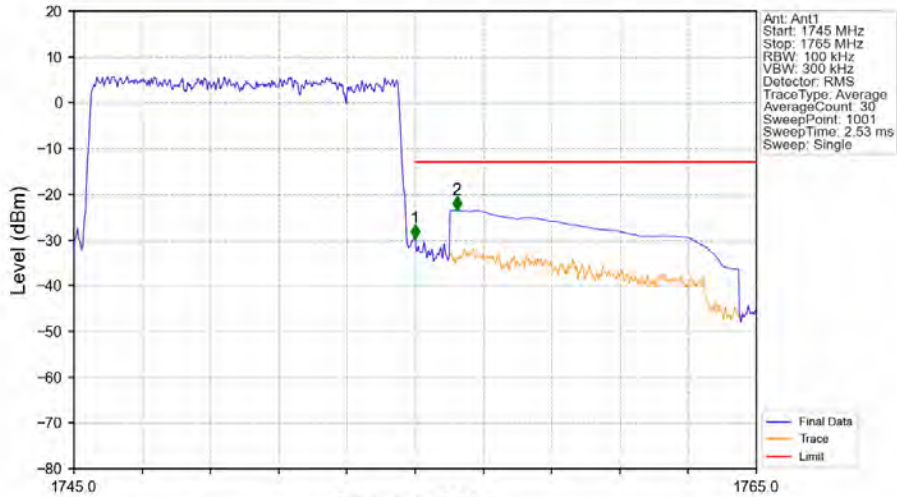
Band4_10MHz_QPSK_HCH_1750MHz_RB_50_0_NTNV
