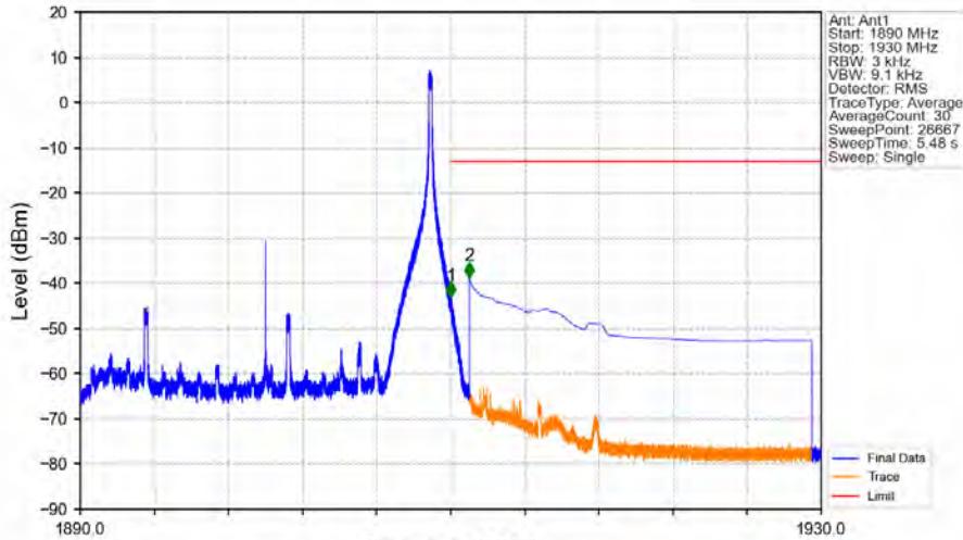
Band2_20MHz_16QAM_HCH_1900MHz_RB_1_99_NTNV
