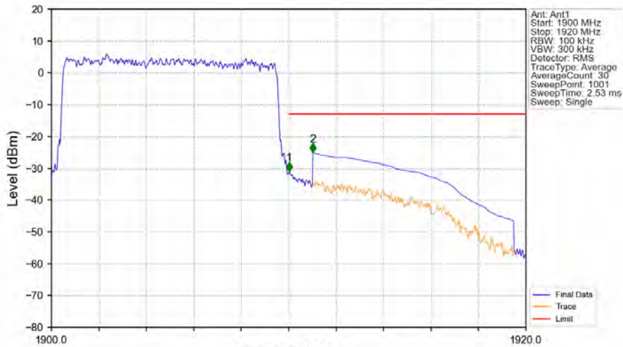
Band2_10MHz_QPSK_HCH_1905MHz_RB_50_0_NTNV
