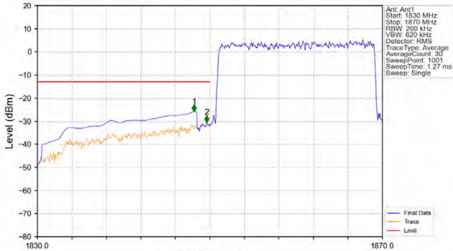
Band2_20MHz_QPSK_LCH_1860MHz_RB_100_0_NTNV
