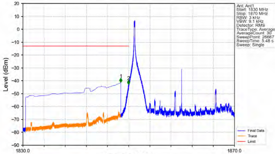
Band2_20MHz_64QAM_LCH_1860MHz_RB_1_0_NTNV
