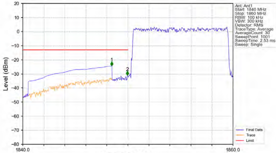
Band2_10MHz_64QAM_LCH_1855MHz_RB_50_0_NTNV
