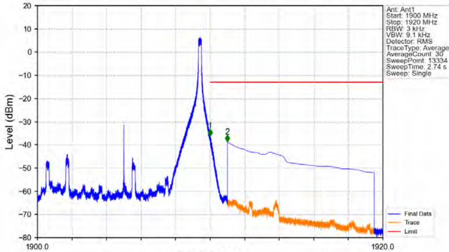
Band2_10MHz_16QAM_HCH_1905MHz_RB_1_49_NTNV
