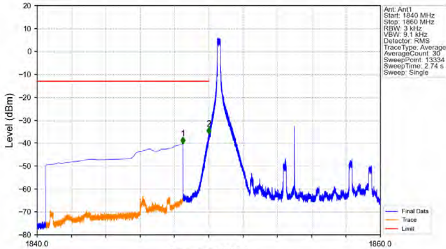
Band2_10MHz_64QAM_LCH_1855MHz_RB_1_0_NTNV
