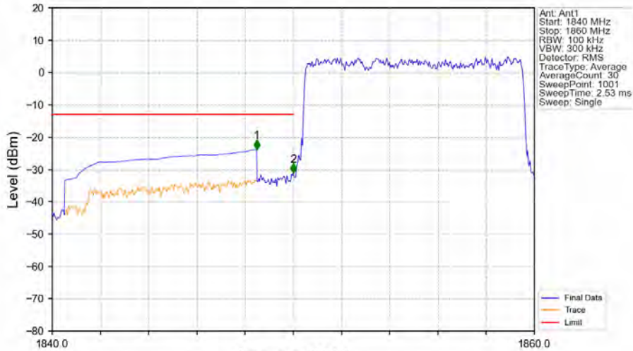
Band2_10MHz_QPSK_LCH_1855MHz_RB_50_0_NTNV
