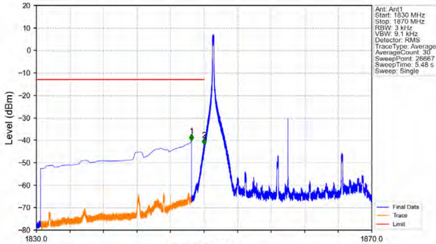
Band2_20MHz_16QAM_LCH_1860MHz_RB_1_0_NTNV
