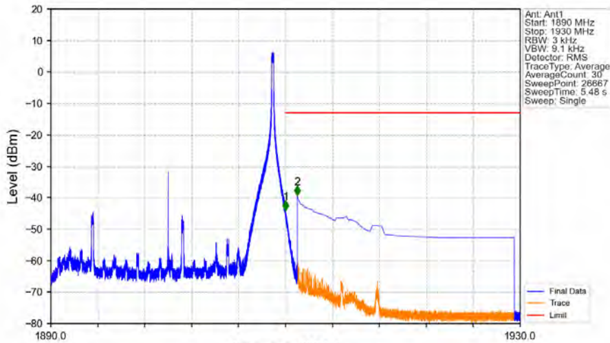
Band2_20MHz_QPSK_HCH_1900MHz_RB_1_99_NTNV
