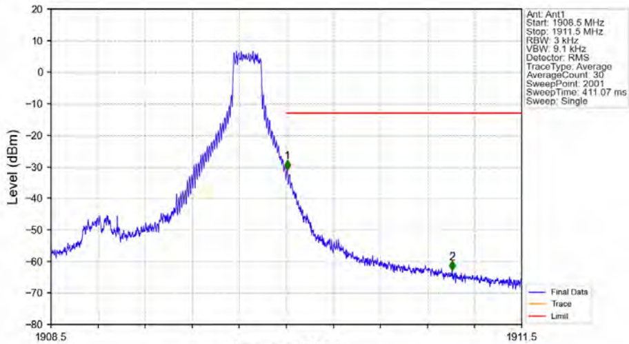
Band2_1.4MHz_QPSK_HCH_1909.3MHz_RB_1_5_NTV
