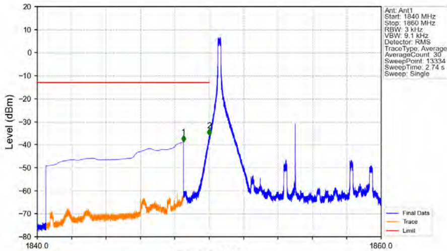
Band2_10MHz_16QAM_LCH_1855MHz_RB_1_0_NTNV
