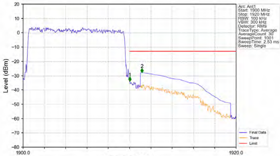
Band2_10MHz_16QAM_HCH_1905MHz_RB_50_0_NTNV
