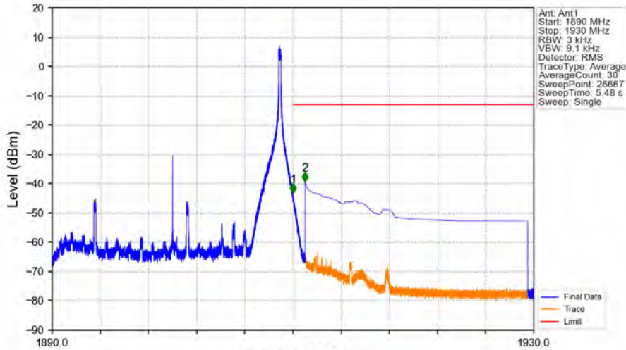
Band2_20MHz_64QAM_HCH_1900MHz_RB_1_99_NTNV
