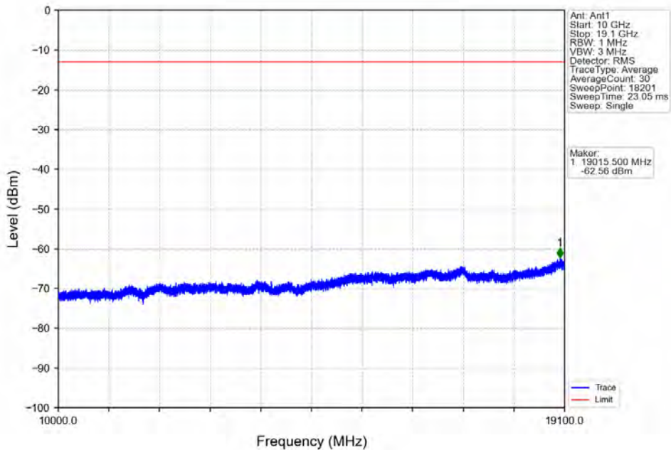
Band2_3MHz_QPSK_MCH_1880MHz_RB_1_0_NTNV
