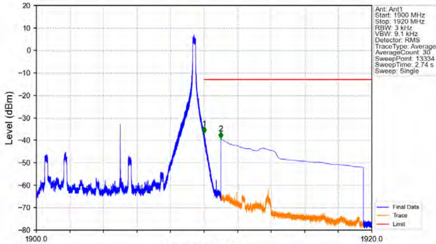
Band2_10MHz_QPSK_HCH_1905MHz_RB_1_49_NTNV
