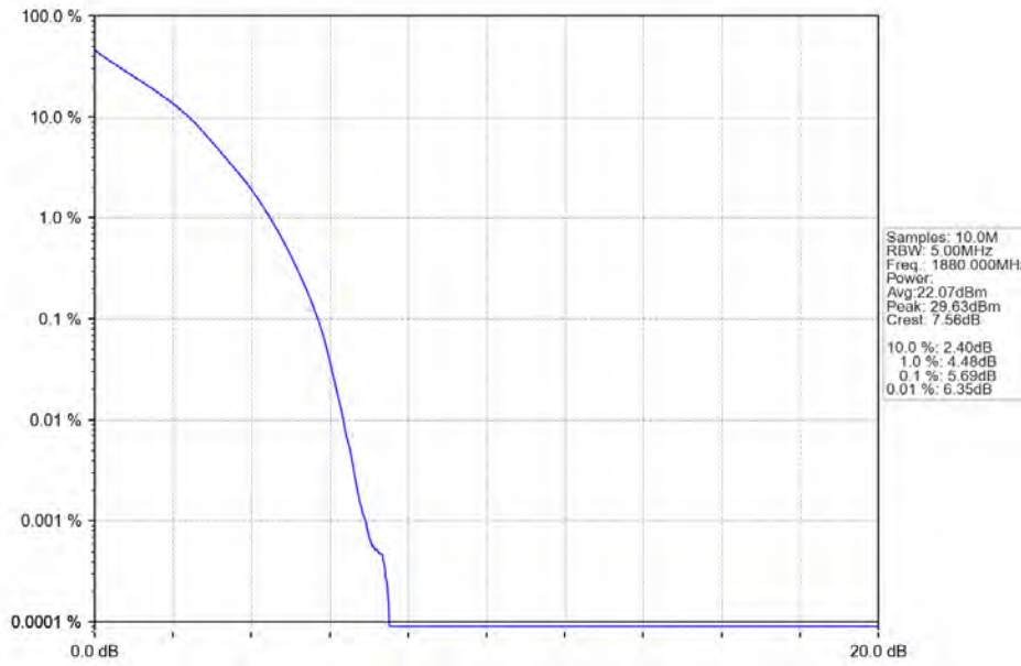
Band2_5MHz_QPSK_MCH_1880MHz_RB_25_0_NTNV
