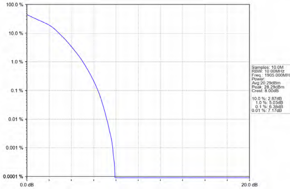
Band2_10MHz_16QAM_HCH_1905MHz_RB_50_0_NTNV
