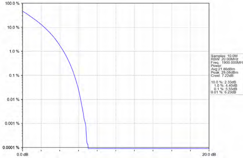
Band2_20MHz_QPSK_HCH_1900MHz_RB_100_0_NTNV
