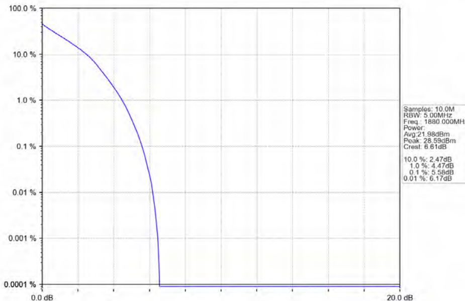
Band2_3MHz_QPSK_MCH_1880MHz_RB_15_0_NTNV
