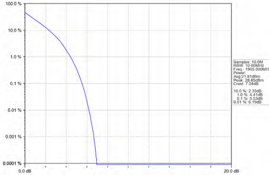
Band2_10MHz_QPSK_HCH_1905MHz_RB_50_0_NTNV
