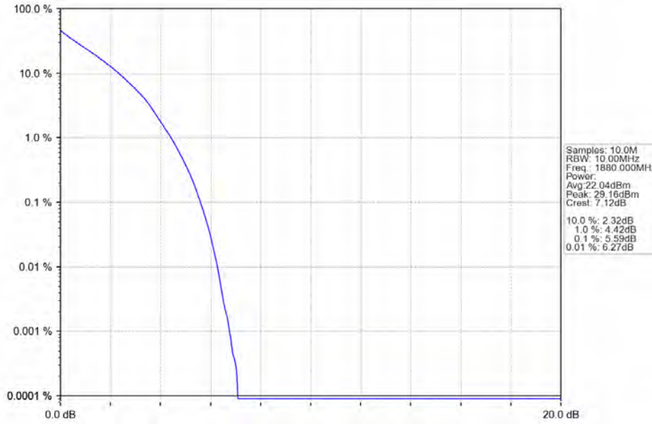
Band2_10MHz_QPSK_MCH_1880MHz_RB_50_0_NTNV
