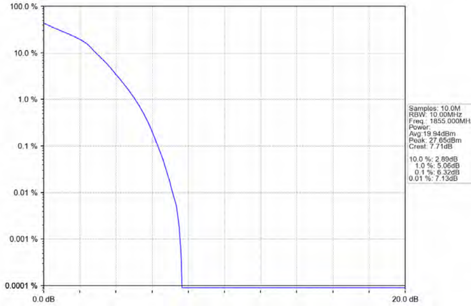
Band2_10MHz_16QAM_LCH_1855MHz_RB_50_0_NTNV
