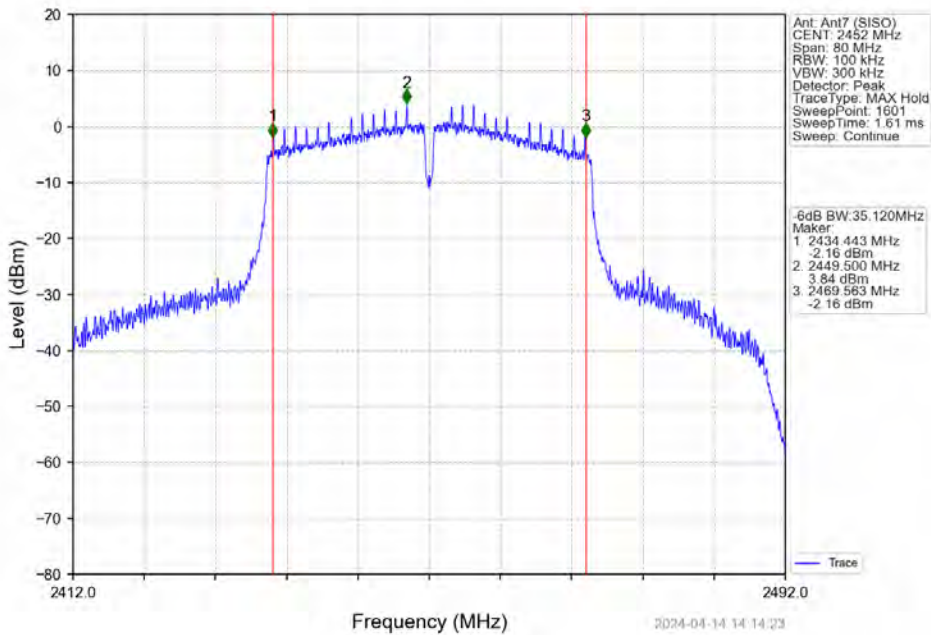
802.11(VHT40) HCH_2452MHz_Ant7 (SISO) NTN
