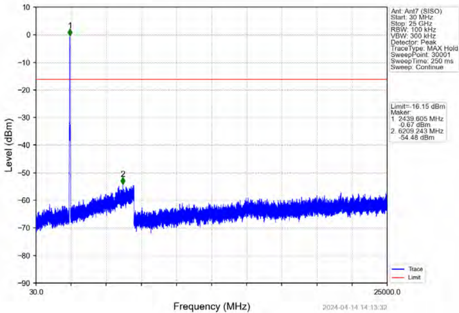
802.11(VHT40)_MCH_2437MHz_Ant7 (SISO)_NTNV
