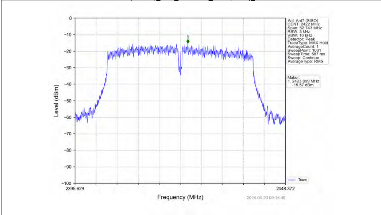
802.11(VHT40)_LCH_2422MHz_Ant7 (SISO)_NTNV
