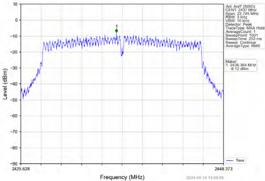
802.11(VHT20)_MCH_2437MHz_Ant7 (SISO)_NTNV
