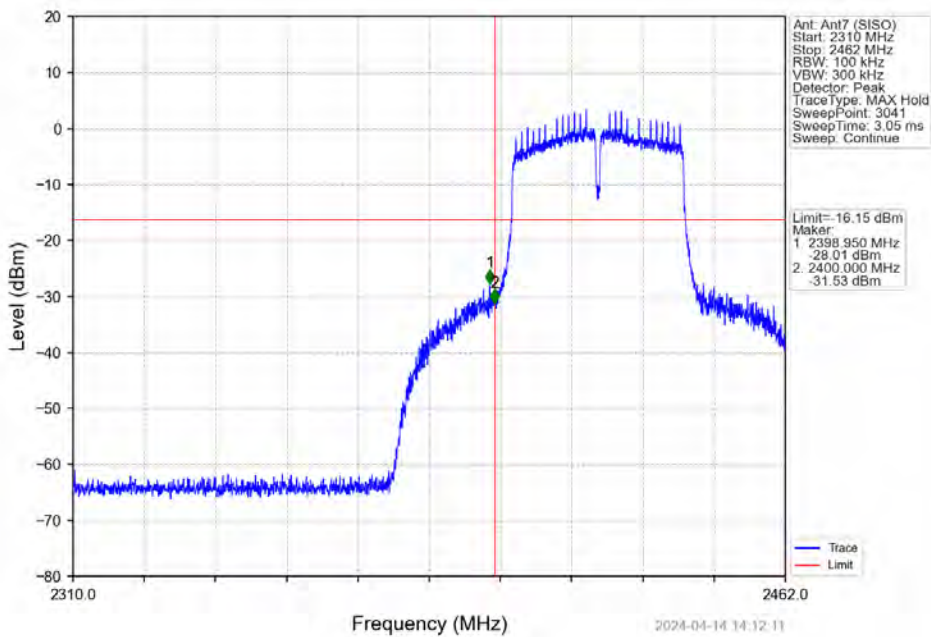
802.11(VHT40)_LCH_2422MHz_Ant7 (SISO)_NTNV
