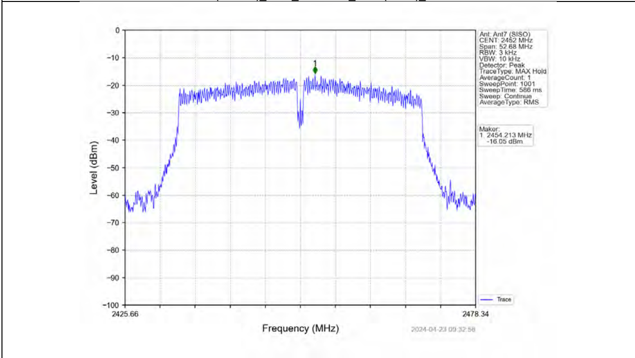
802.11(VHT40) HCH_2452MHz_Ant7 (SISO) NTN
