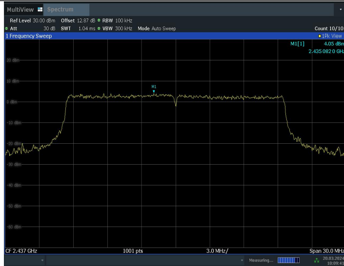
11AX20MIMO_Ant9_2437_0~Reference
