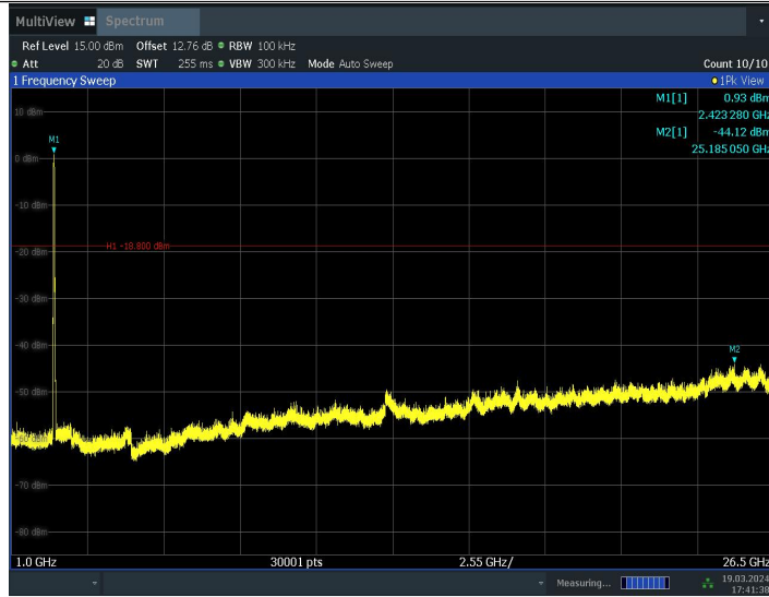
11N40MIMO_Ant9_2422_0~Reference
