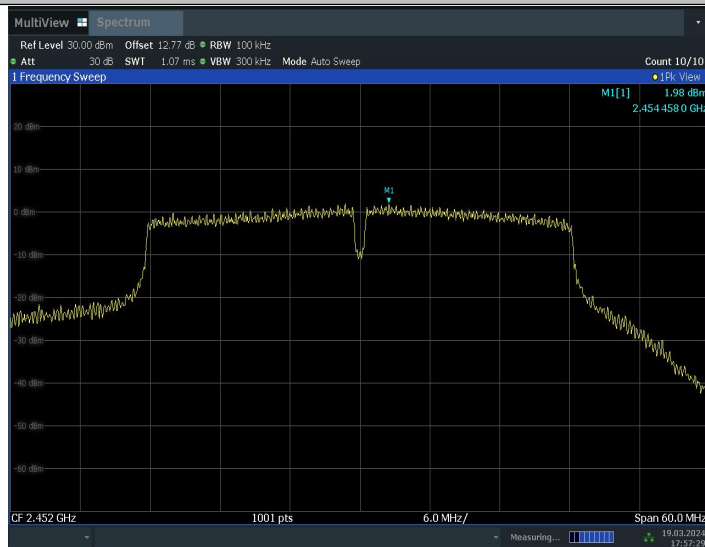
11N40MIMO_Ant9_2452_0~Reference
