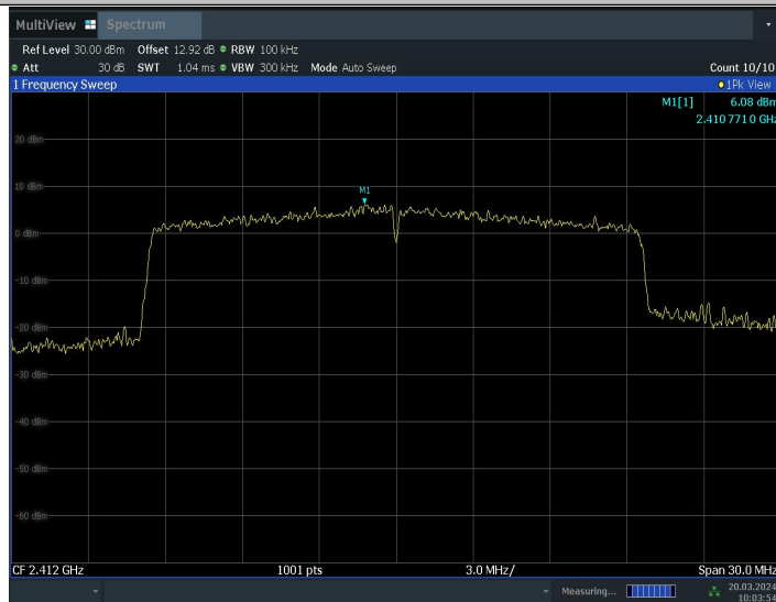
11AX20MIMO_Ant9_2412_0~Reference
