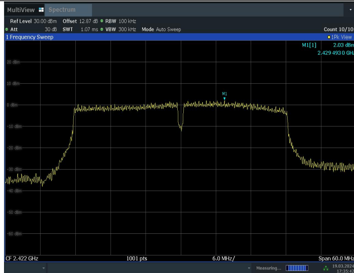
11N40MIMO_Ant9_2422_0~Reference
