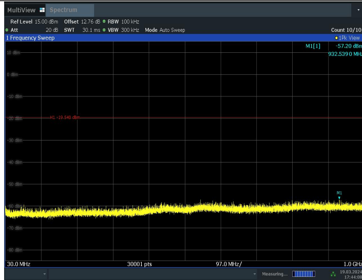
11N40MIMO_Ant8_2437_30~1000
