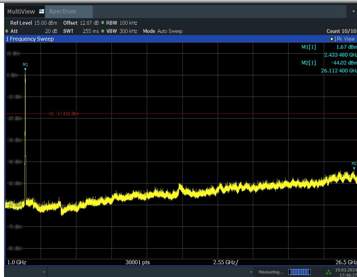
11N40MIMO_Ant9_2437_1000~26500
