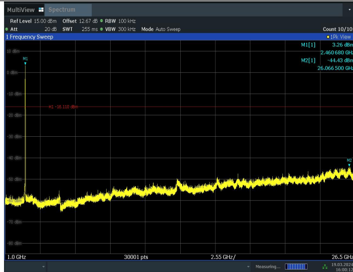
11N20MIMO_Ant9_2462_0~Reference
