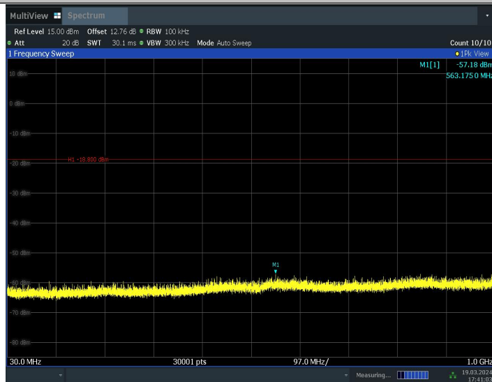
11N40MIMO_Ant8_2422_30~1000
