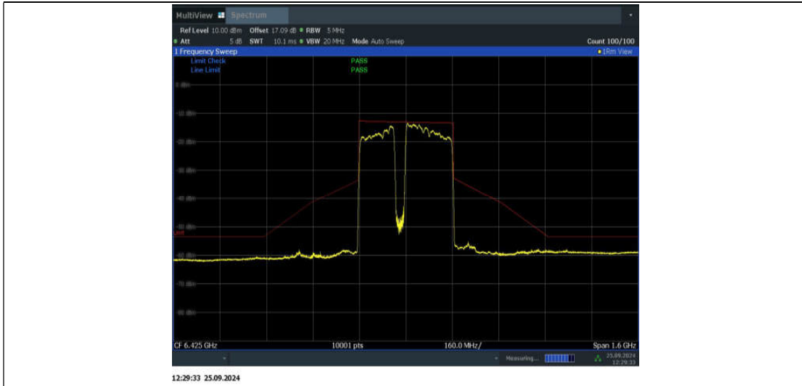
11BE320MIMO_Ant2_6425_3*996+484_Non-OFDMA_5
