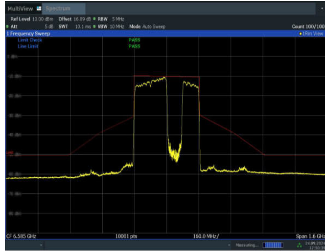
11BE320MIMO_Ant2_6585_3*996_Non-OFDMA_3
