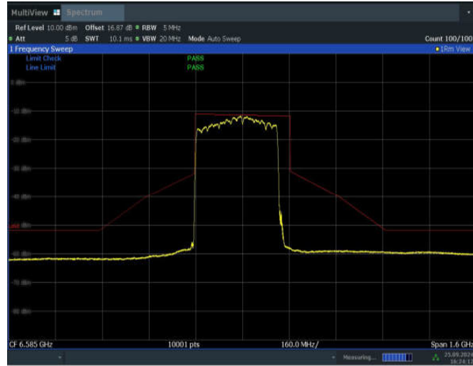
11BE320MIMO_Ant1_6585_3*996+484_Non-OFDMA_8
