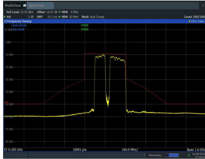
11BE320MIMO_Ant1_6585_2*996+484_Non-OFDMA_9
