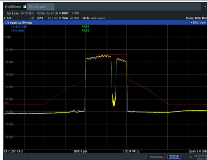
11BE320MIMO_Ant2_6265_3*996+484_Non-OFDMA_6
