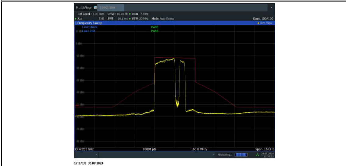
11BE320MIMO_Ant2_6265_2*996+484_Non-OFDMA_5
