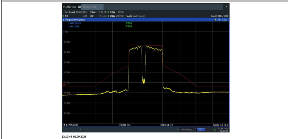
11BE320MIMO_Ant2_6265_3*996+484_Non-OFDMA_4
