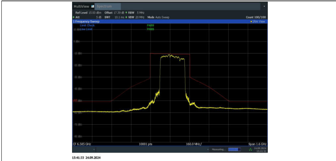
11BE320MIMO_Ant2_6585_3*996_Non-OFDMA_1
