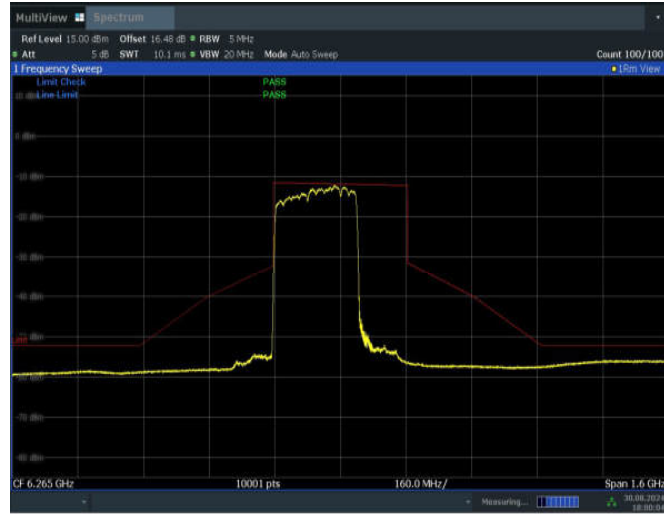
11BE320MIMO_Ant2_6265_2*996+484_Non-OFDMA_6
