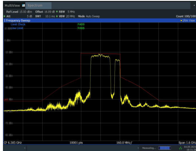
11BE320MIMO_Ant2_6585_2*996+484_Non-OFDMA_11
