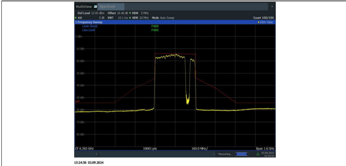
11BE320MIMO_Ant2_6265_3*996+484_Non-OFDMA_8
