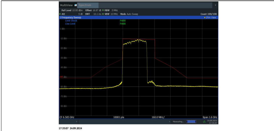
11BE320MIMO_Ant1_6585_3*996+484_Non-OFDMA_1
