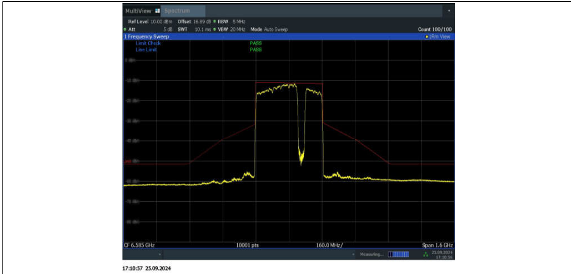
11BE320MIMO_Ant2_6585_3*996+484_Non-OFDMA_7
