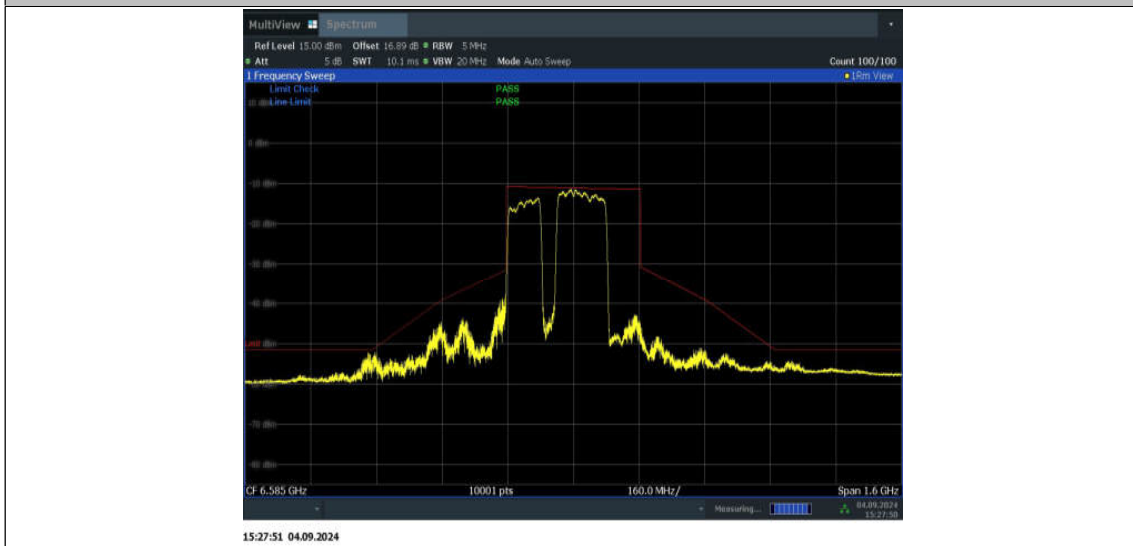
11BE320MIMO_Ant2_6585_2*996+484_Non-OFDMA_4
