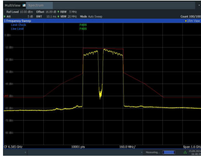
11BE320MIMO_Ant2_6585_3*996+484_Non-OFDMA_4
