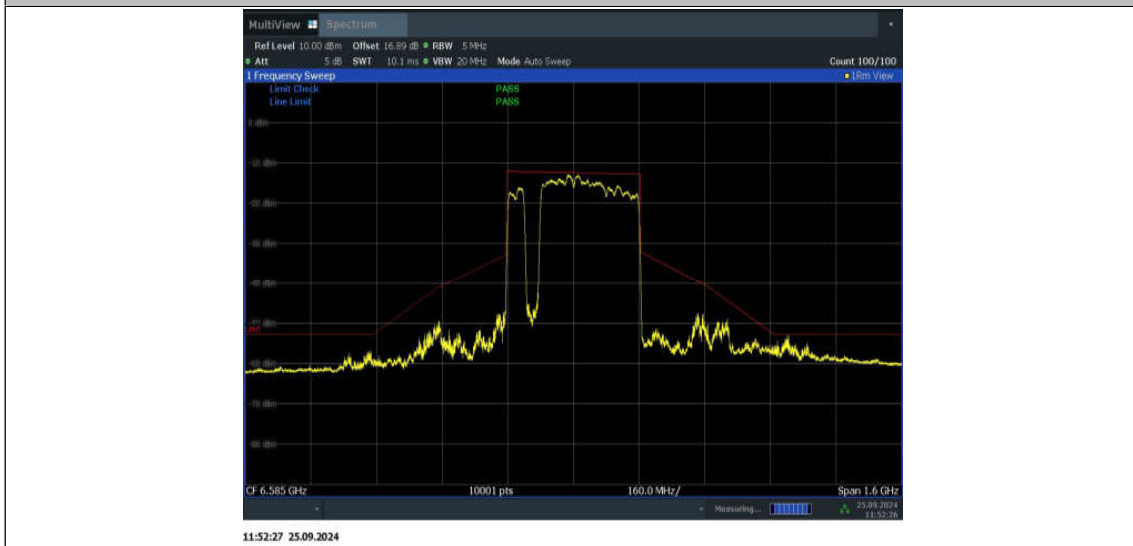
11BE320MIMO_Ant2_6585_3*996+484_Non-OFDMA_3
