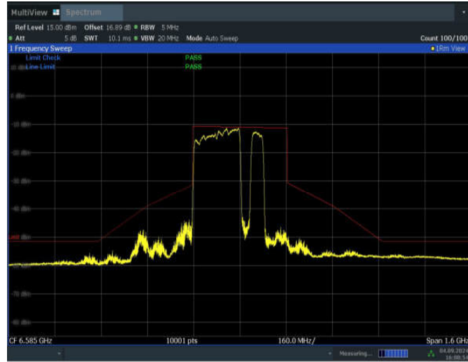
11BE320MIMO_Ant2_6585_2*996+484_Non-OFDMA_5
