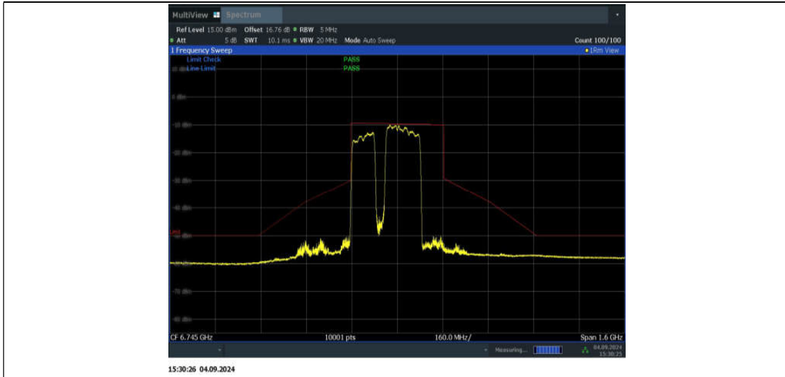
11BE320MIMO_Ant1_6745_2*996+484_Non-OFDMA_4
