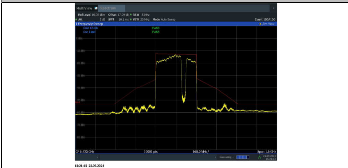
11BE320MIMO_Ant2_6425_3*996+484_Non-OFDMA_6
