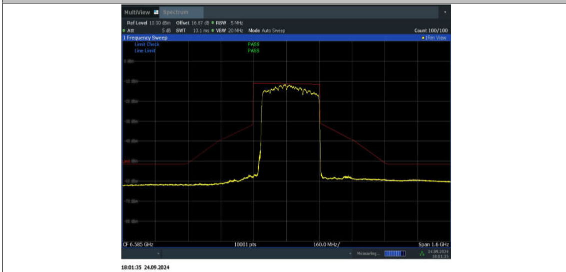
11BE320MIMO_Ant1_6585_3*996+484_Non-OFDMA_2
