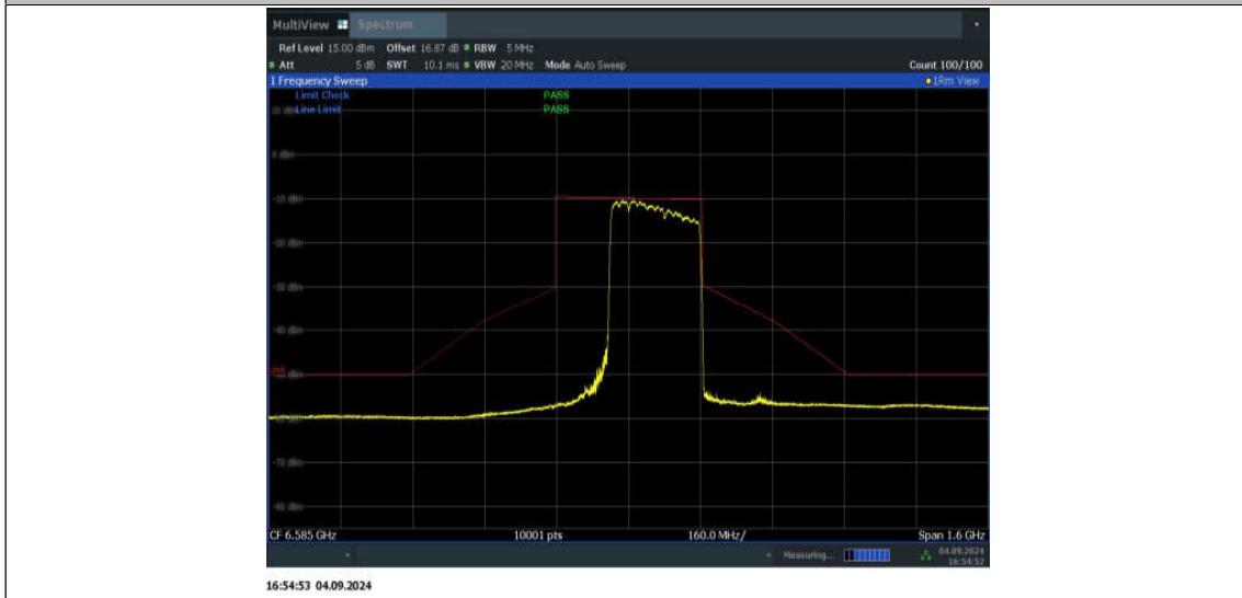
11BE320MIMO_Ant1_6585_2*996+484_Non-OFDMA_8
