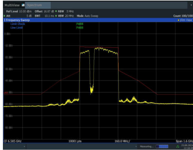
11BE320MIMO_Ant1_6585_3*996+484_Non-OFDMA_3
