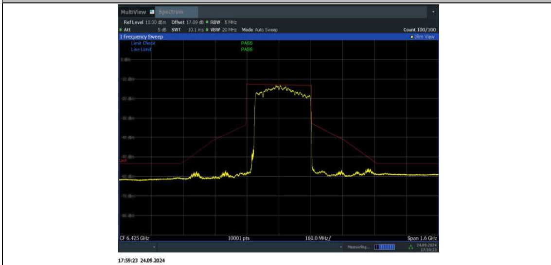
11BE320MIMO_Ant2_6425_3*996+484_Non-OFDMA_1
