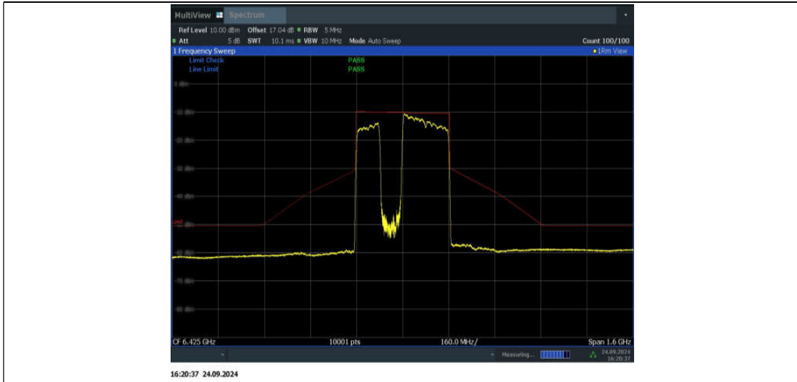
11BE320MIMO_Ant1_6425_3*996_Non-OFDMA_3
