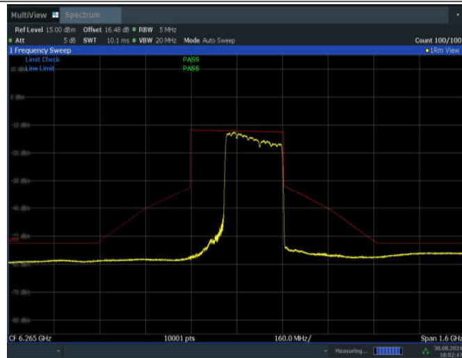
11BE320MIMO_Ant2_6265_2*996+484_Non-OFDMA_7
