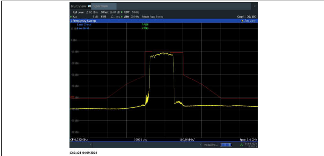
11BE320MIMO_Ant1_6585_2*996+484_Non-OFDMA_2
