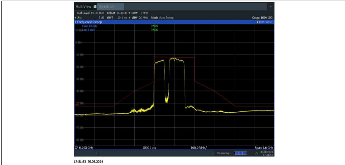
11BE320MIMO_Ant2_6265_2*996+484_Non-OFDMA_4
