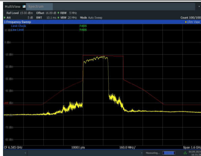
11BE320MIMO_Ant2_6585_2*996+484_Non-OFDMA_6
