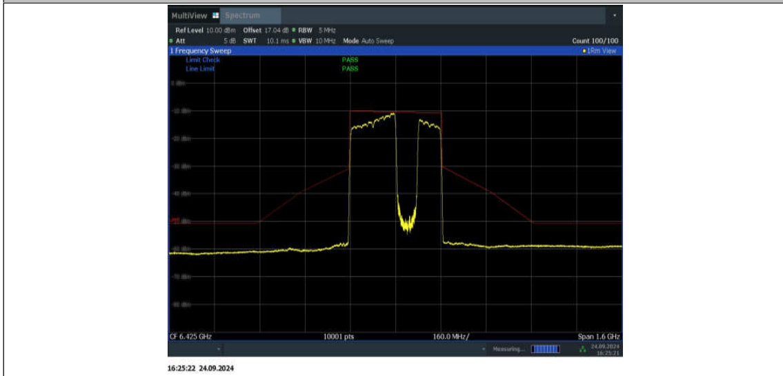
11BE320MIMO_Ant1_6425_3*996_Non-OFDMA_4
