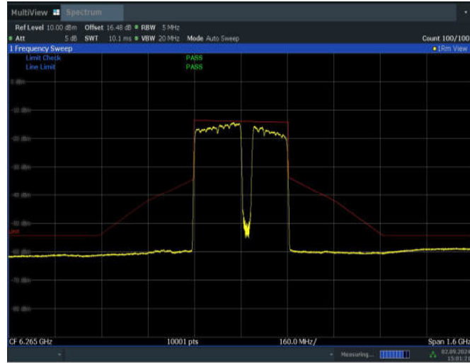
11BE320MIMO_Ant2_6265_3*996+484_Non-OFDMA_5
