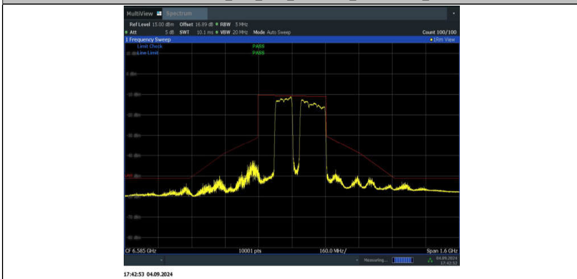
11BE320MIMO_Ant2_6585_2*996+484_Non-OFDMA_9
