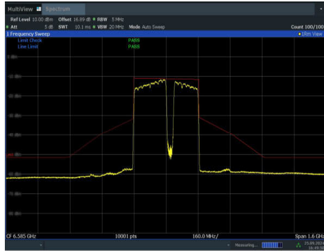
11BE320MIMO_Ant2_6585_3*996+484_Non-OFDMA_5
