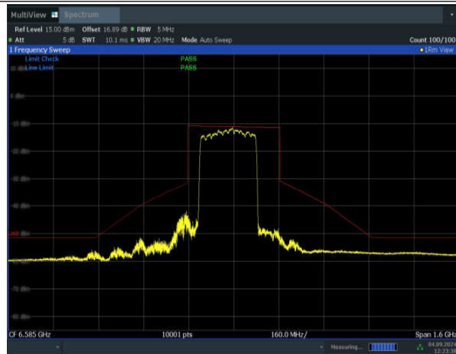
11BE320MIMO_Ant2_6585_2*996+484_Non-OFDMA_1
