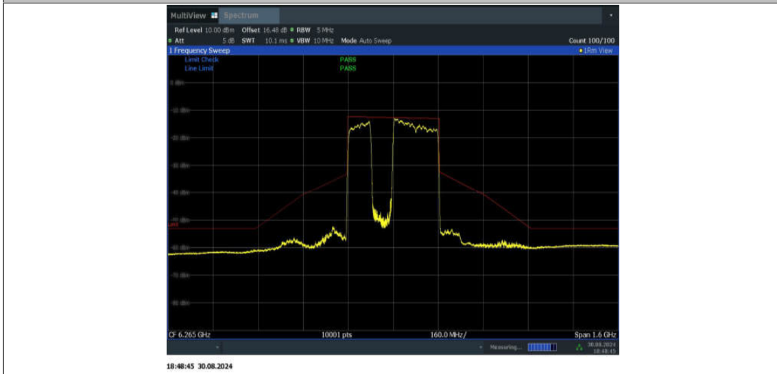
11BE320MIMO_Ant2_6265_3*996_Non-OFDMA_3
