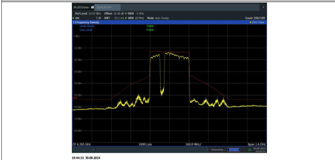
11BE320MIMO_Ant2_6265_3*996+484_Non-OFDMA_4
