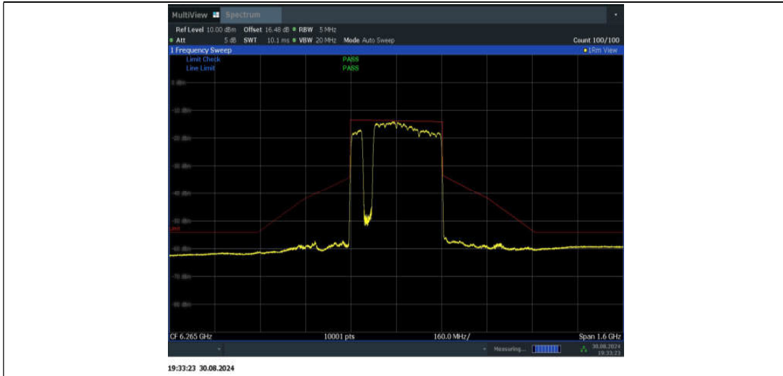
11BE320MIMO_Ant2_6265_3*996+484_Non-OFDMA_3
