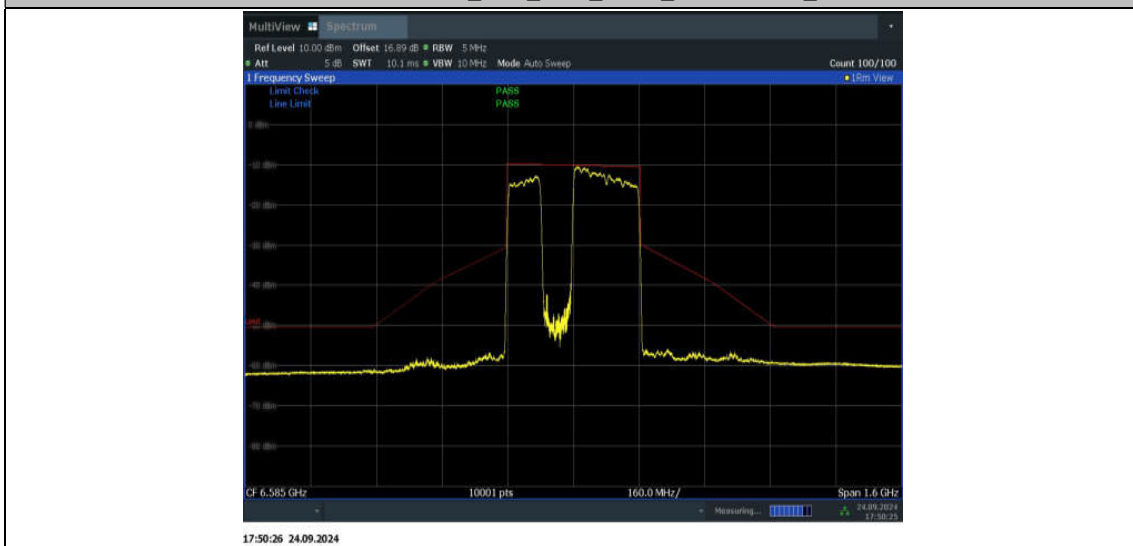
11BE320MIMO_Ant2_6585_3*996_Non-OFDMA_2
