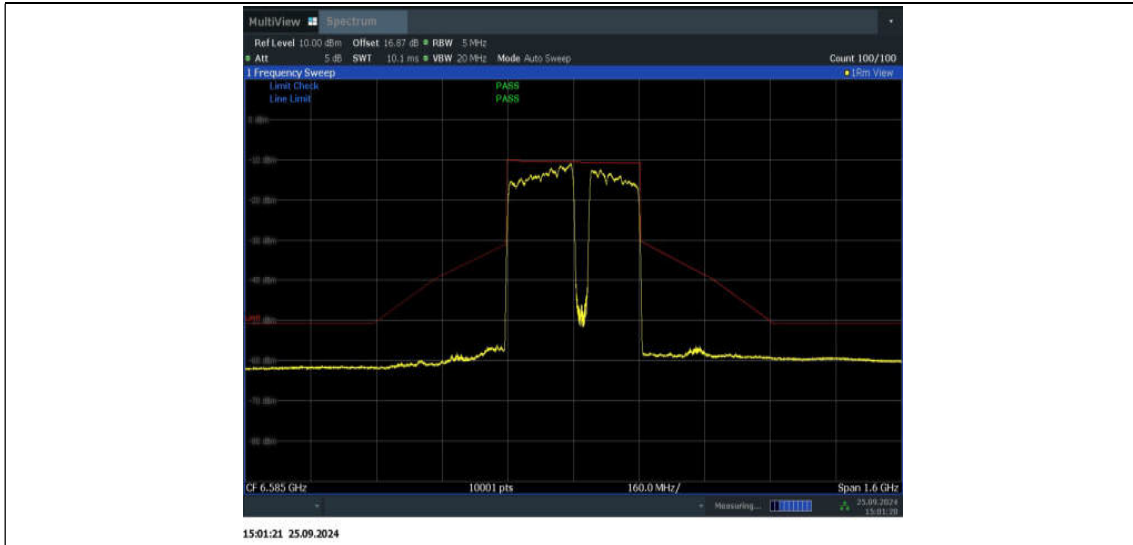
11BE320MIMO_Ant1_6585_3*996+484_Non-OFDMA_6
