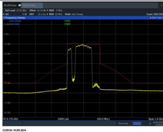
11BE320MIMO_Ant1_6745_2*996+484_Non-OFDMA_3
