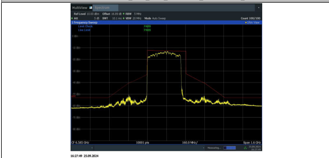
11BE320MIMO_Ant2_6585_3*996+484_Non-OFDMA_8
