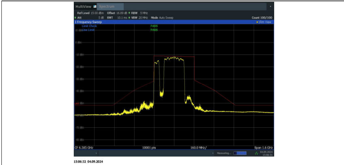
11BE320MIMO_Ant2_6585_2*996+484_Non-OFDMA_3
