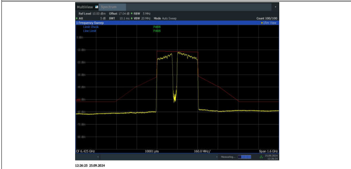
11BE320MIMO_Ant1_6425_3*996+484_Non-OFDMA_5
