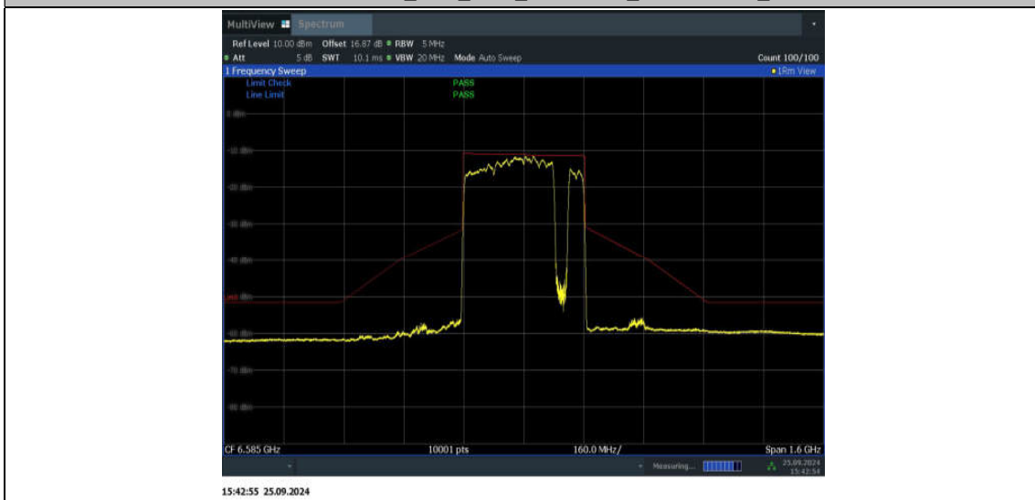
11BE320MIMO_Ant1_6585_3*996+484_Non-OFDMA_7
