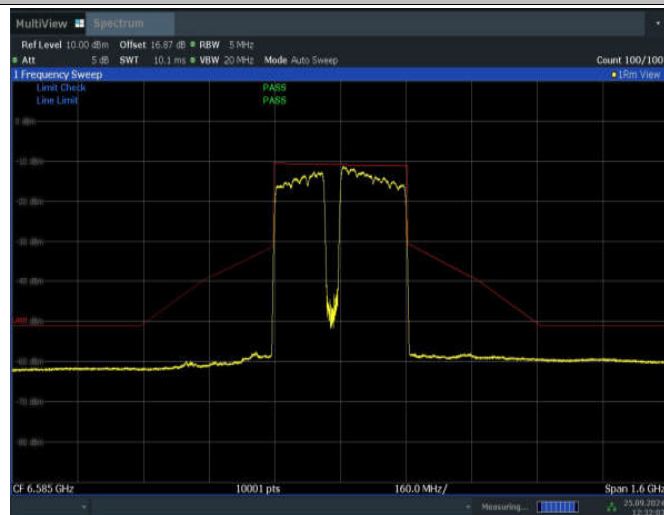
11BE320MIMO_Ant1_6585_3*996+484_Non-OFDMA_4
