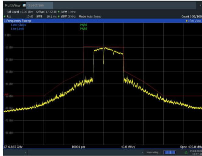
11BE80MIMO_Ant2_6865_484+242_Non-OFDMA_1
