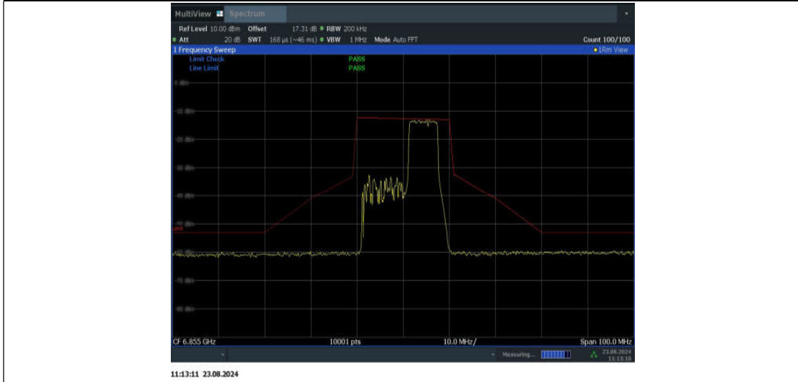
11BE20MIMO_Ant1_6855_106+26_OFDMA_2
