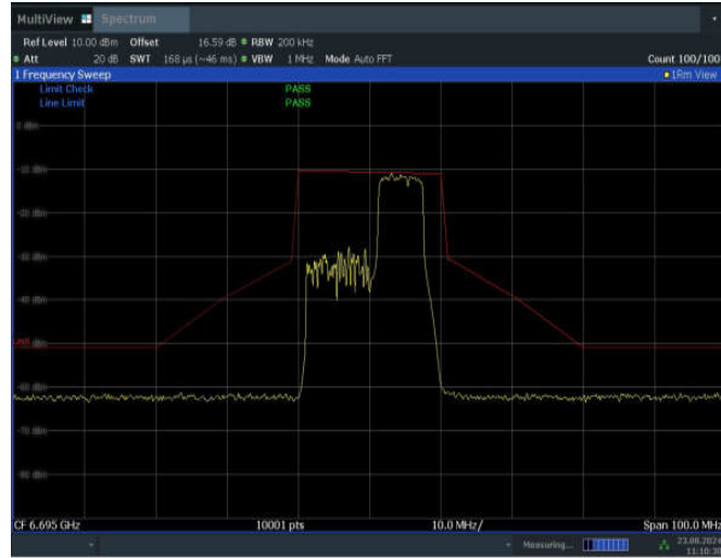
11BE20MIMO_Ant2_6695_52+26_OFDMA_3
