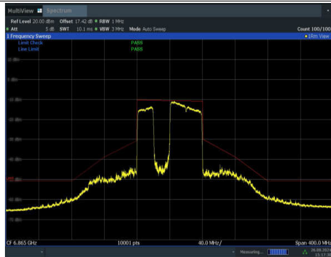
11BE80MIMO_Ant2_6865_484+242_Non-OFDMA_2
