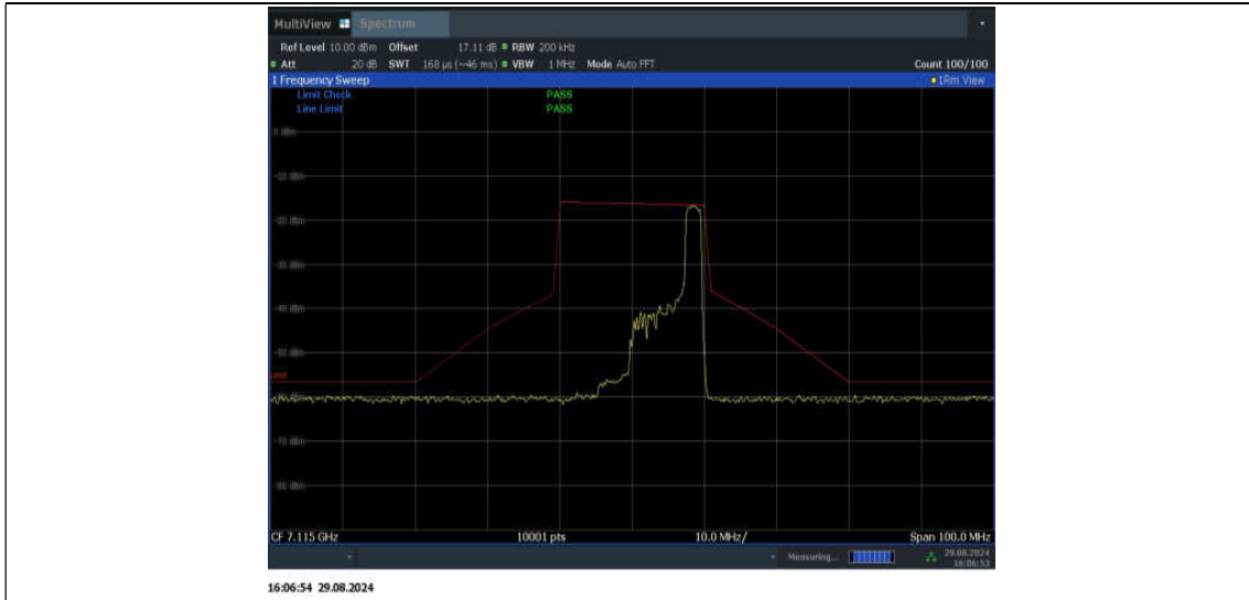
11BE20MIMO_Ant1_7115_52Tone_RU40
