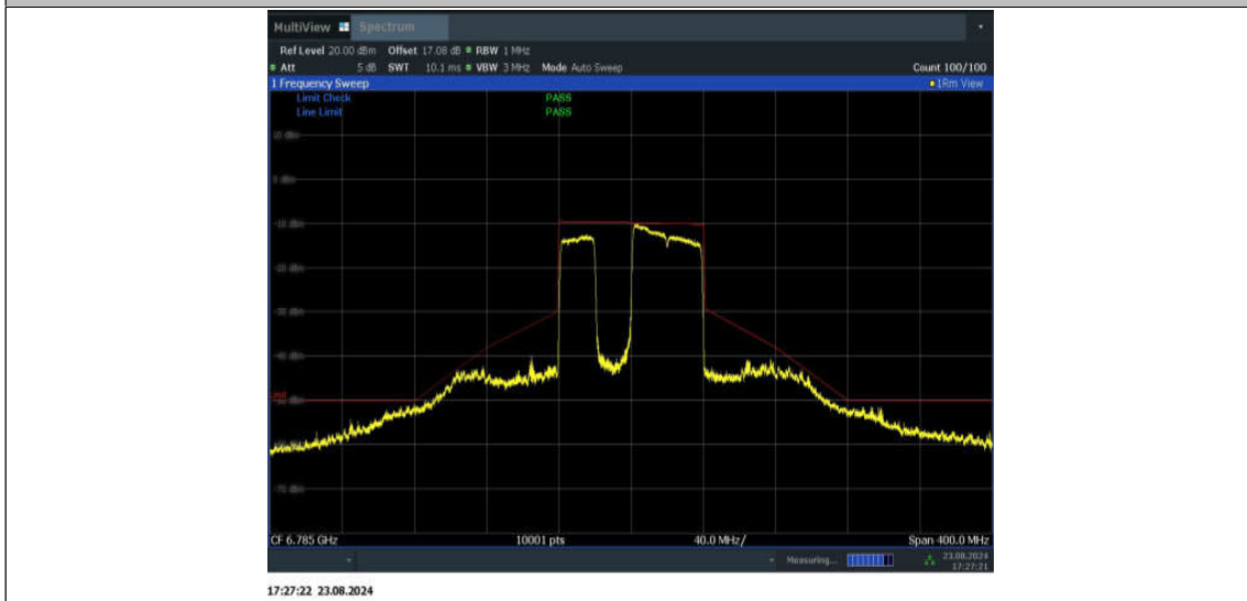
11BE80MIMO_Ant2_6785_484+242_Non-OFDMA_3
