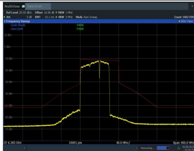
11BE80MIMO_Ant1_6385_484+242_Non-OFDMA_4
