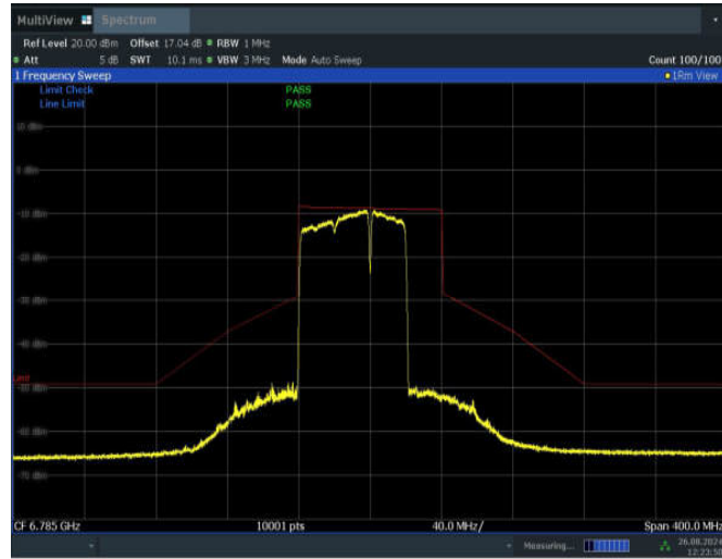
11BE80MIMO_Ant1_6785_484+242_Non-OFDMA_4
