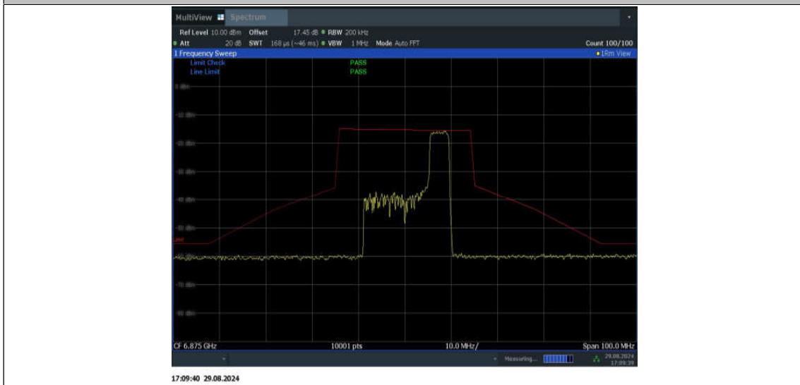
11BE20MIMO_Ant2_6875_106Tone_RU54
