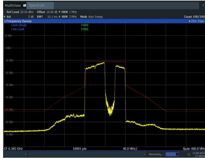
11BE80MIMO_Ant1_6385_484+242_Non-OFDMA_3
