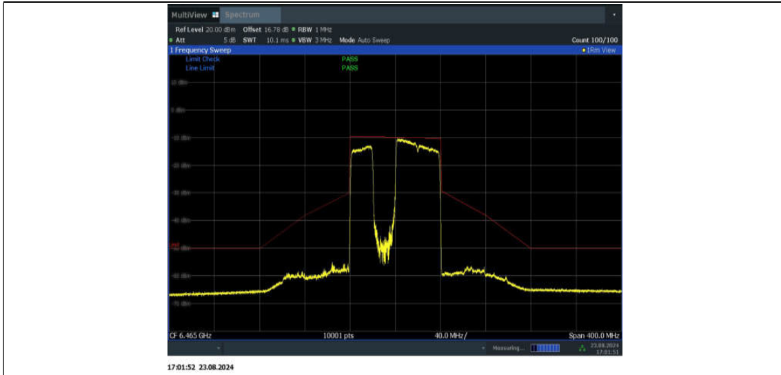
11BE80MIMO_Ant1_6465_484+242_Non-OFDMA_3
