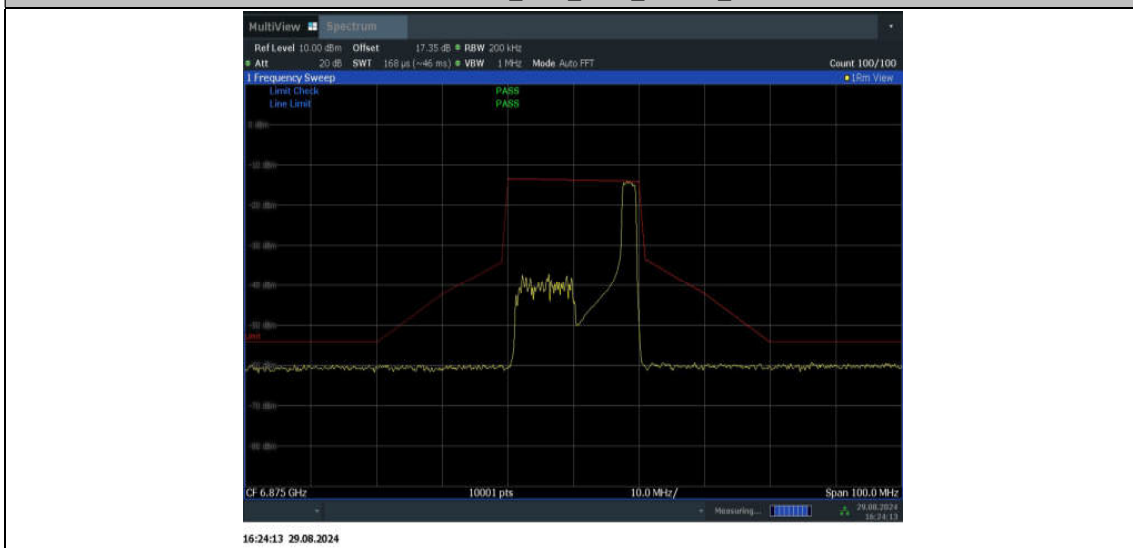
11BE20MIMO_Ant1_6875_26Tone_RU8
