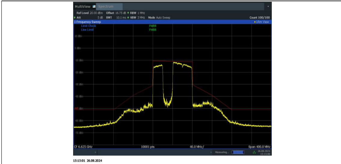
11BE80MIMO_Ant2_6625_484+242_Non-OFDMA_3
