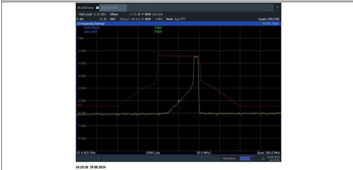
11BE20MIMO_Ant1_6855_52Tone_RU40
