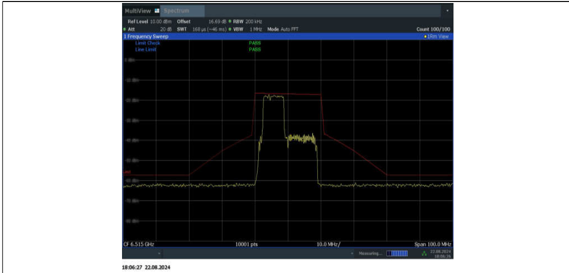
11BE20MIMO_Ant2_6515_106+26_OFDMA_1
