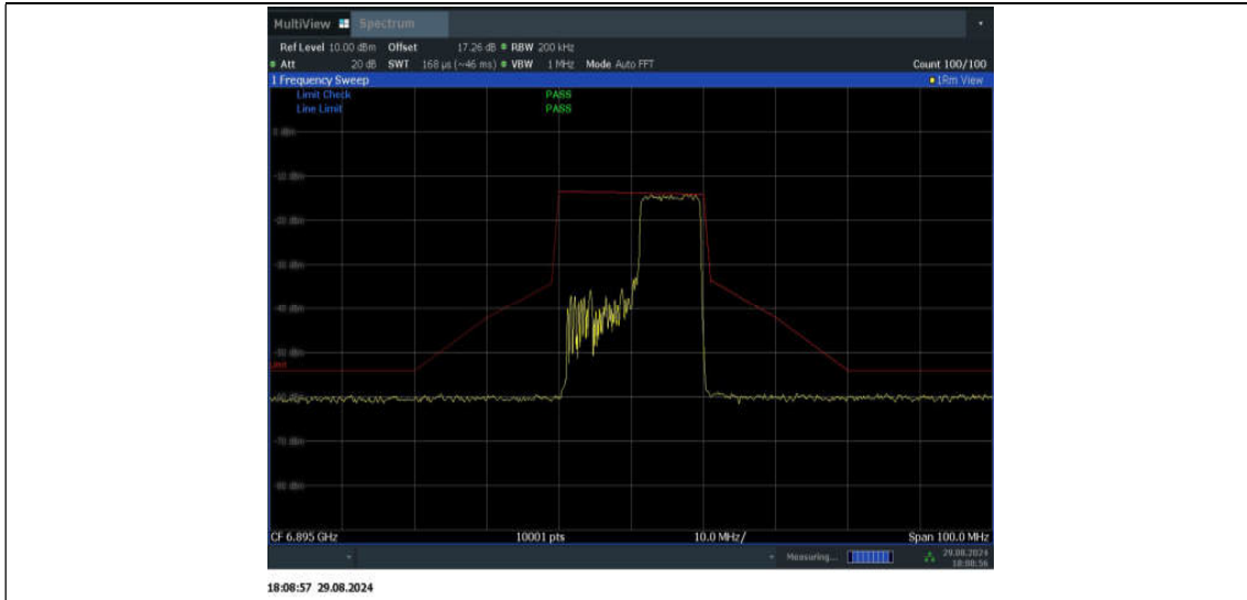
11BE20MIMO_Ant2_6895_26Tone_RU8
