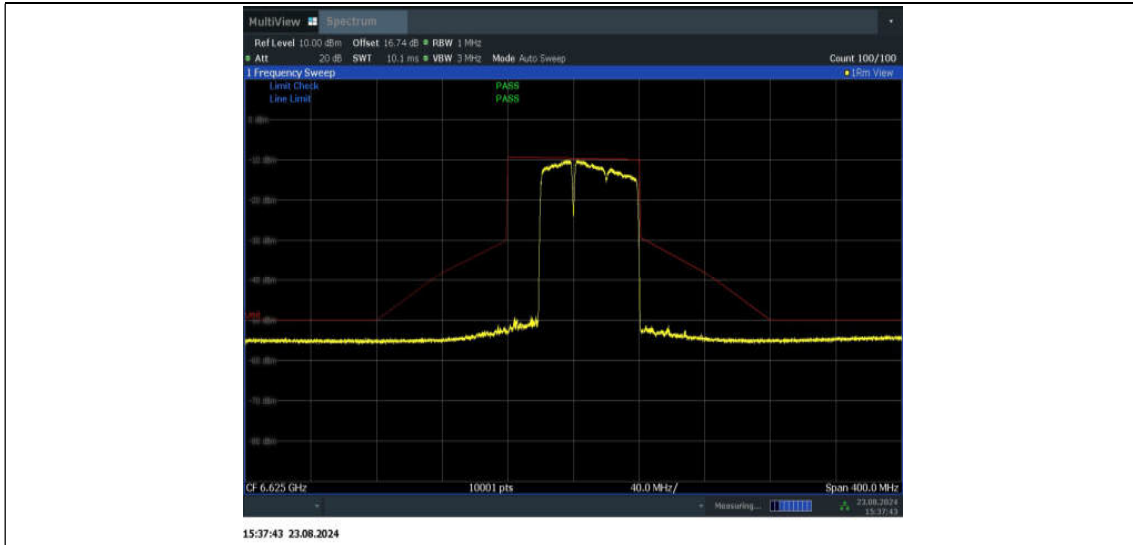
11BE80MIMO_Ant1_6625_484+242_Non-OFDMA_2
