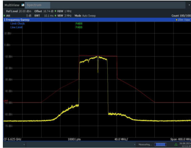
11BE80MIMO_Ant1_6625_484+242_Non-OFDMA_4
