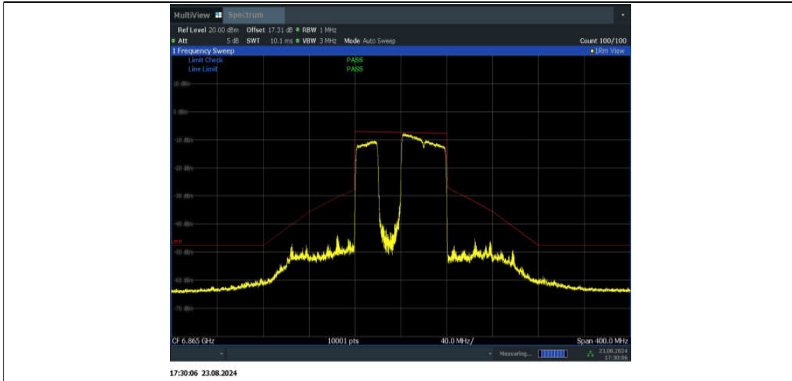
11BE80MIMO_Ant1_6865_484+242_Non-OFDMA_3
