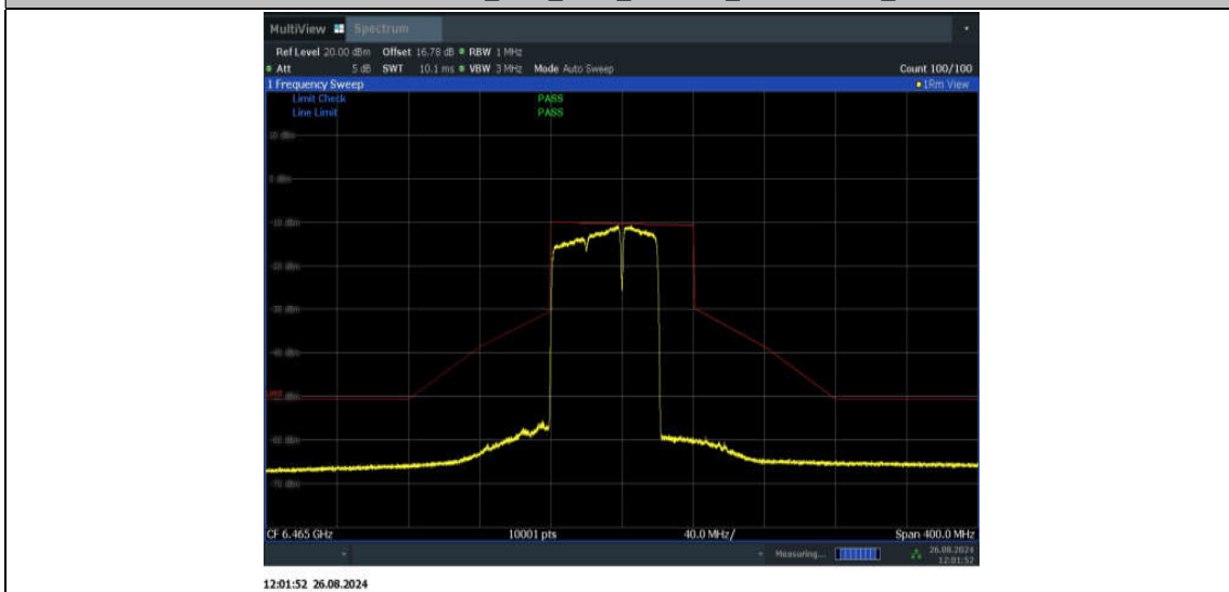
11BE80MIMO_Ant1_6465_484+242_Non-OFDMA_4
