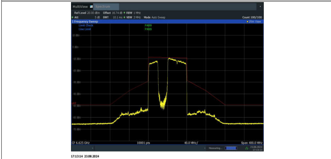
11BE80MIMO_Ant1_6625_484+242_Non-OFDMA_3
