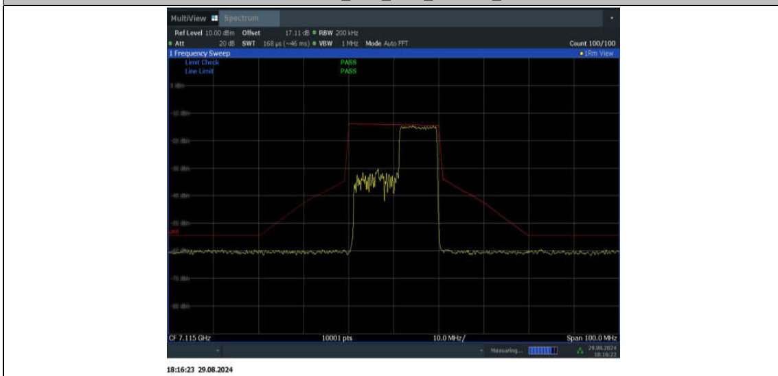
11BE20MIMO_Ant1_7115_106Tone_RU54
