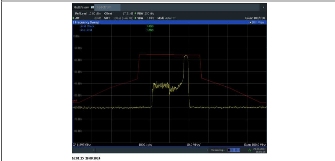
11BE20MIMO_Ant2_6895_52Tone_RU40
