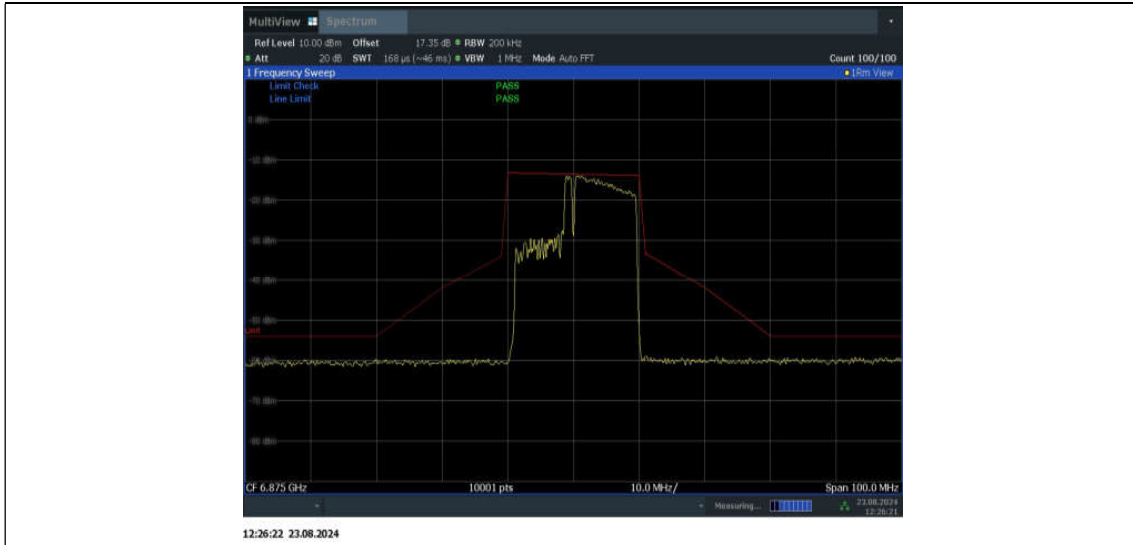
11BE20MIMO_Ant2_6875_52+26_OFDMA_3
