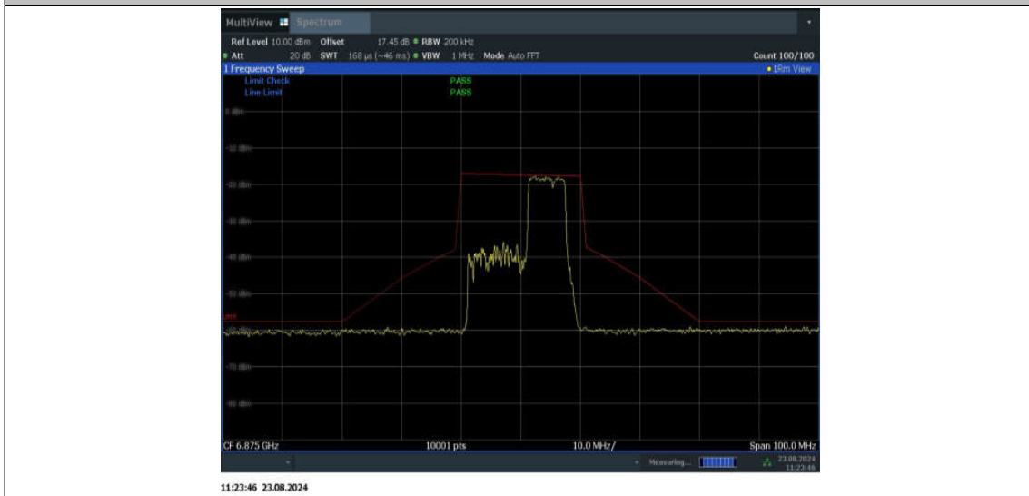
11BE20MIMO_Ant2_6875_106+26_OFDMA_2
