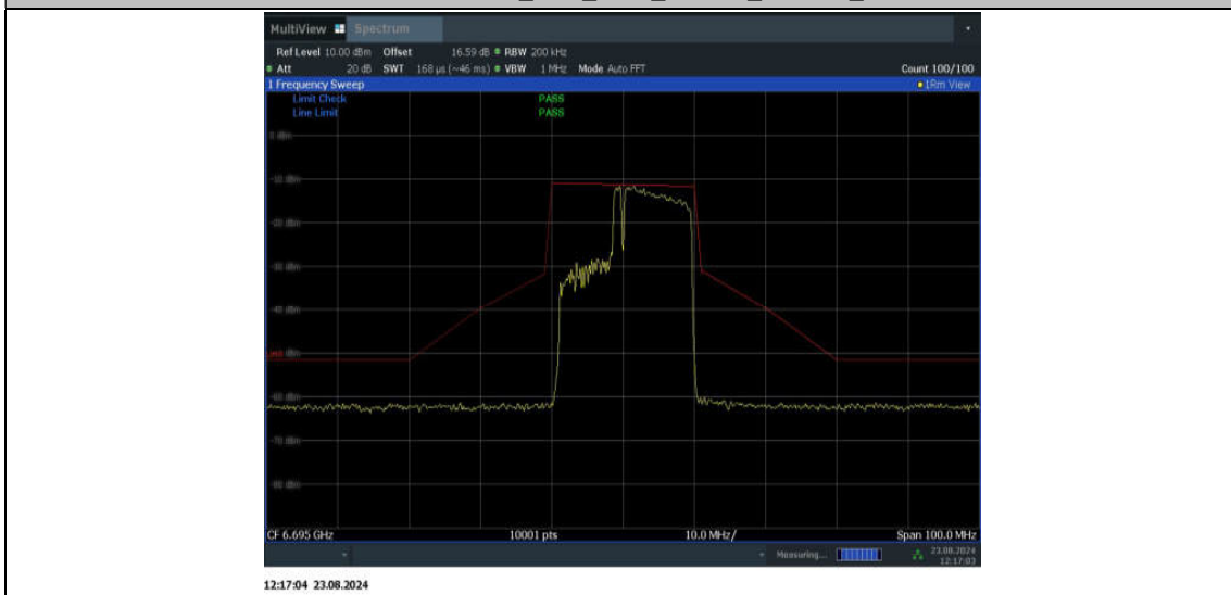
11BE20MIMO_Ant1_6695_106+26_OFDMA_2
