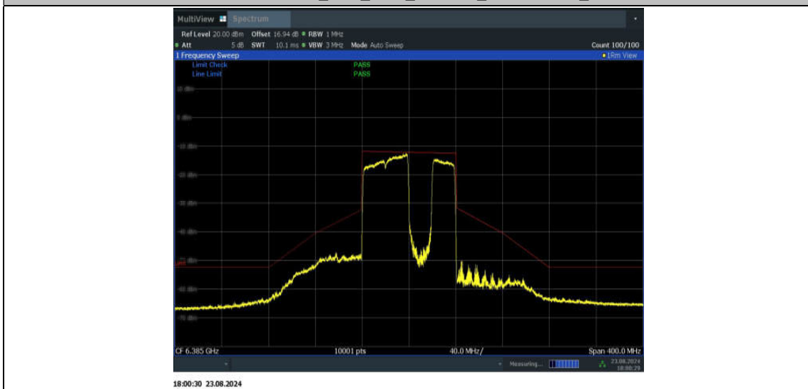
11BE80MIMO_Ant2_6385_484+242_Non-OFDMA_3
