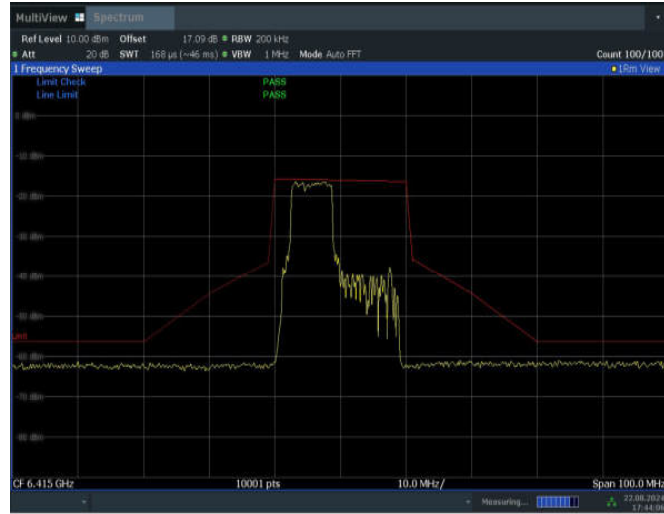
11BE20MIMO_Ant2_6415_52+26_OFDMA_1
