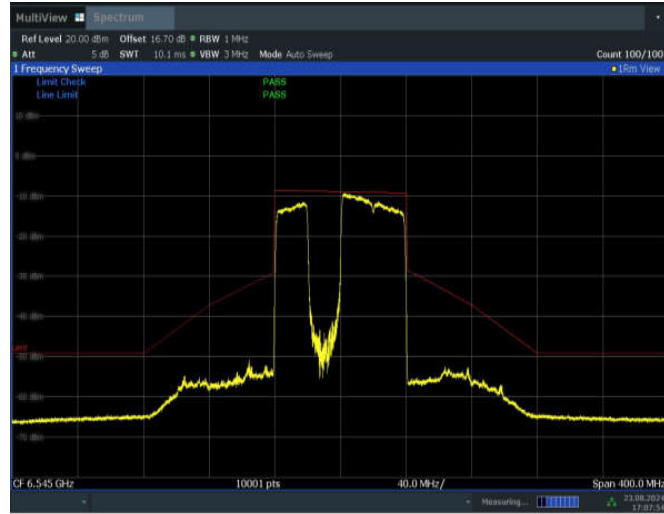
11BE80MIMO_Ant1_6545_484+242_Non-OFDMA_2
