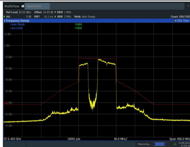
11BE80MIMO_Ant2_6465_484+242_Non-OFDMA_2
