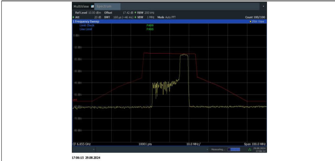
11BE20MIMO_Ant2_6855_106Tone_RU54
