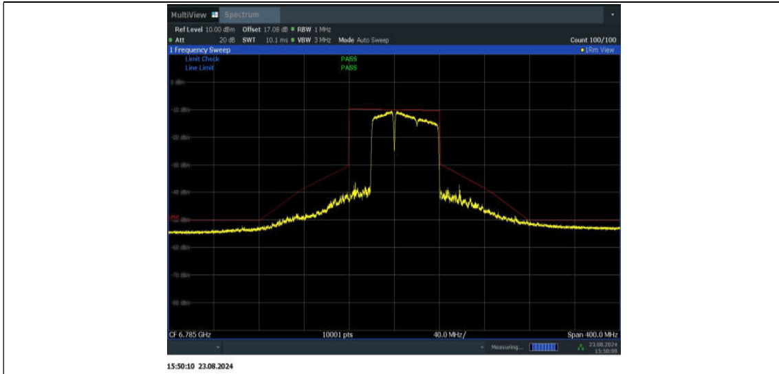
11BE80MIMO_Ant2_6785_484+242_Non-OFDMA_2
