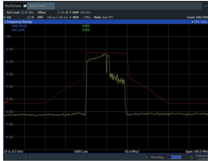
11BE20MIMO_Ant2_6415_106+26_OFDMA_1
