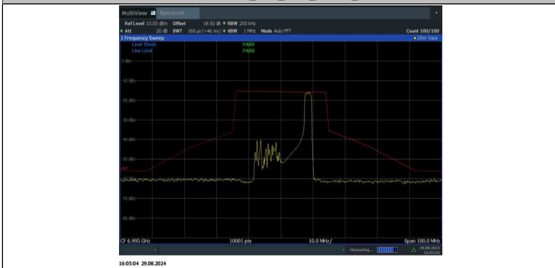
11BE20MIMO_Ant2_6995_26Tone_RU8
