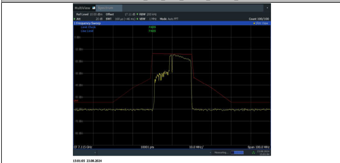
11BE20MIMO_Ant1_7115_106+26_OFDMA_2
