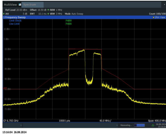
11BE80MIMO_Ant2_6705_484+242_Non-OFDMA_4
