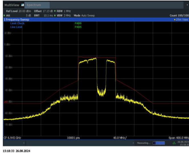
11BE80MIMO_Ant2_6945_484+242_Non-OFDMA_4
