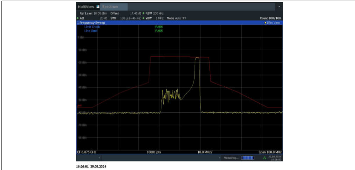
11BE20MIMO_Ant2_6875_52Tone_RU40
