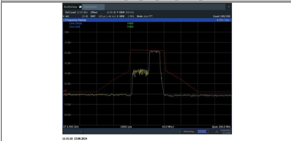
11BE20MIMO_Ant1_6995_52+26_OFDMA_3
