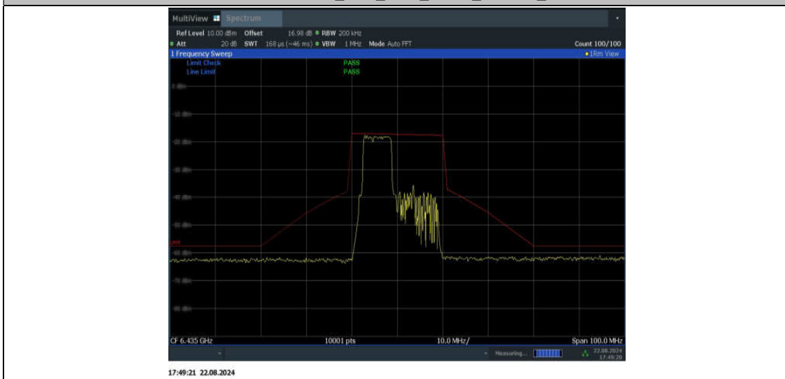
11BE20MIMO_Ant2_6435_52+26_OFDMA_1
