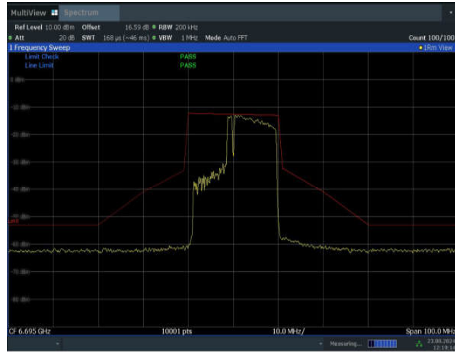
11BE20MIMO_Ant2_6695_106+26_OFDMA_2
