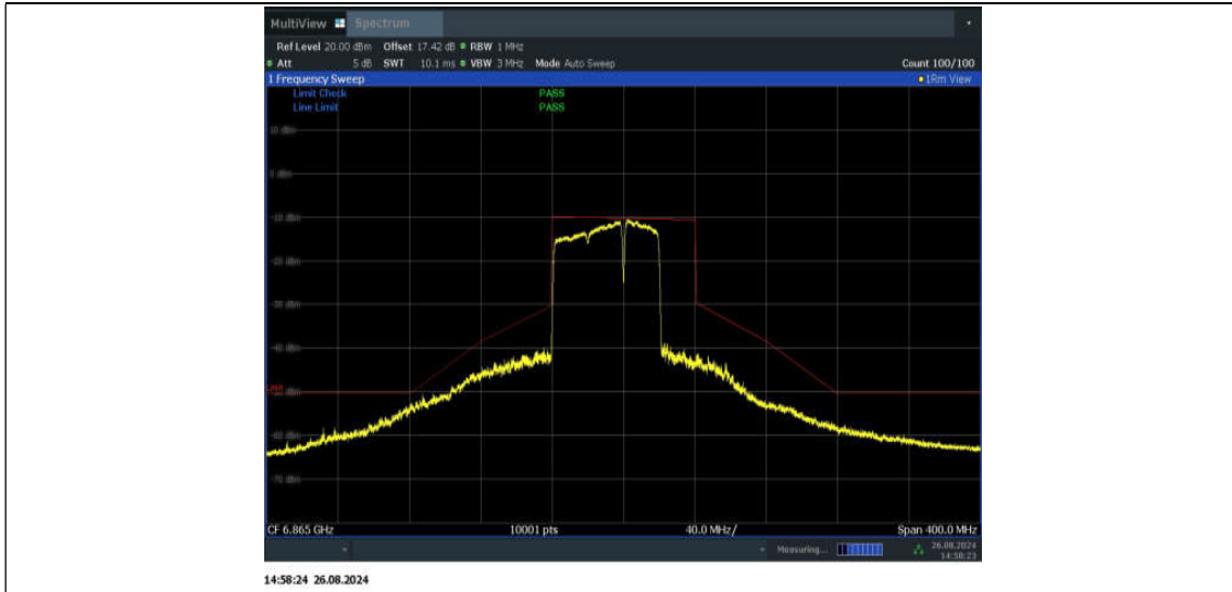
11BE80MIMO_Ant2_6865_484+242_Non-OFDMA_4
