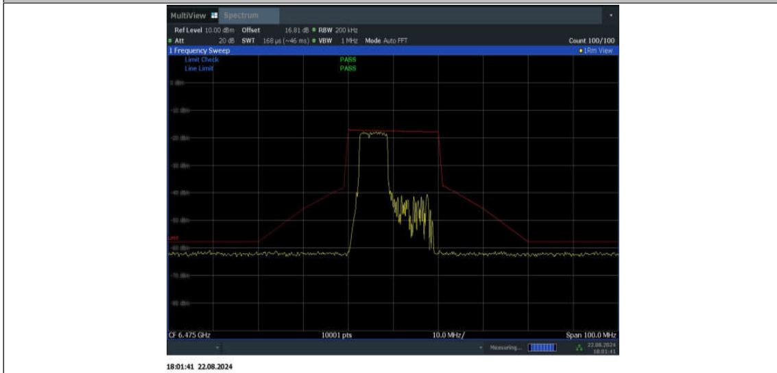
11BE20MIMO_Ant2_6475_106+26_OFDMA_1
