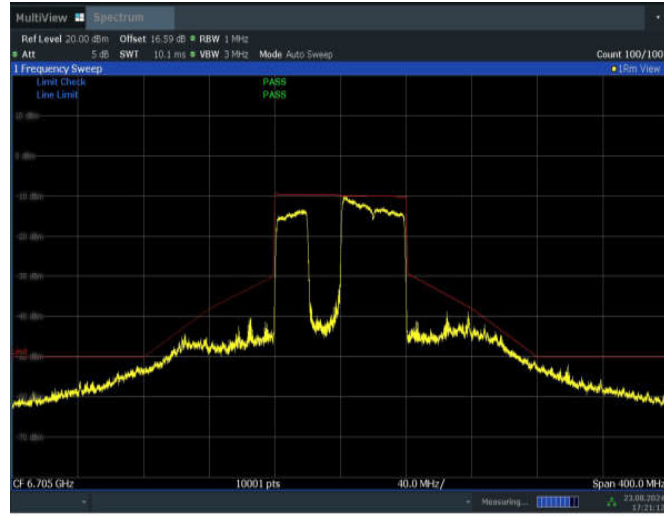
11BE80MIMO_Ant2_6705_484+242_Non-OFDMA_2
