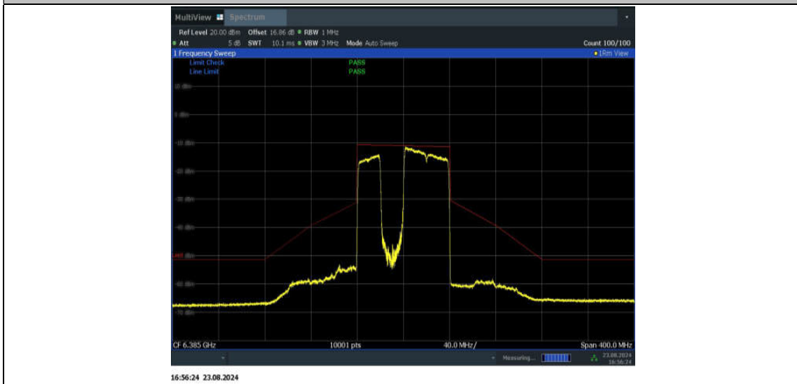
11BE80MIMO_Ant1_6385_484+242_Non-OFDMA_2
