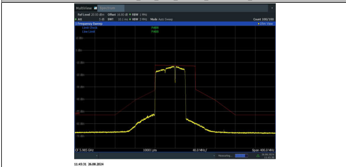
11BE80MIMO_Ant2_5985_484+242_Non-OFDMA_4
