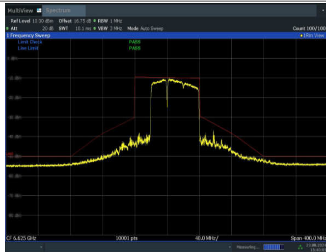
11BE80MIMO_Ant2_6625_484+242_Non-OFDMA_1
