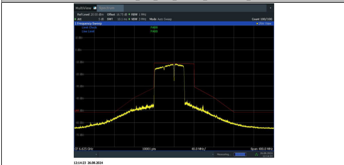
11BE80MIMO_Ant2_6625_484+242_Non-OFDMA_4
