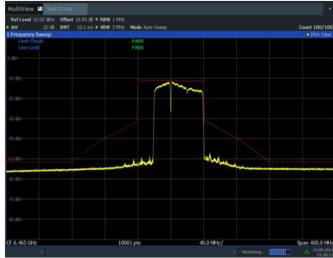
11BE80MIMO_Ant2_6465_484+242_Non-OFDMA_1
