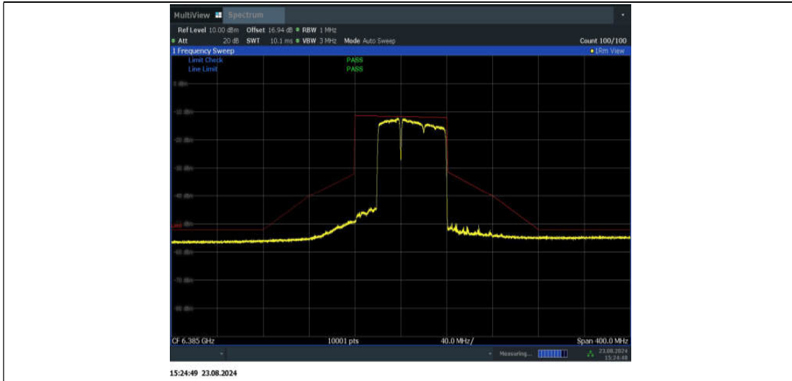
11BE80MIMO_Ant2_6385_484+242_Non-OFDMA_2
