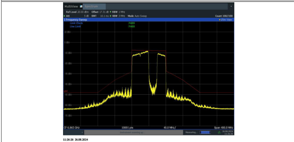
11BE80MIMO_Ant1_6865_484+242_Non-OFDMA_4
