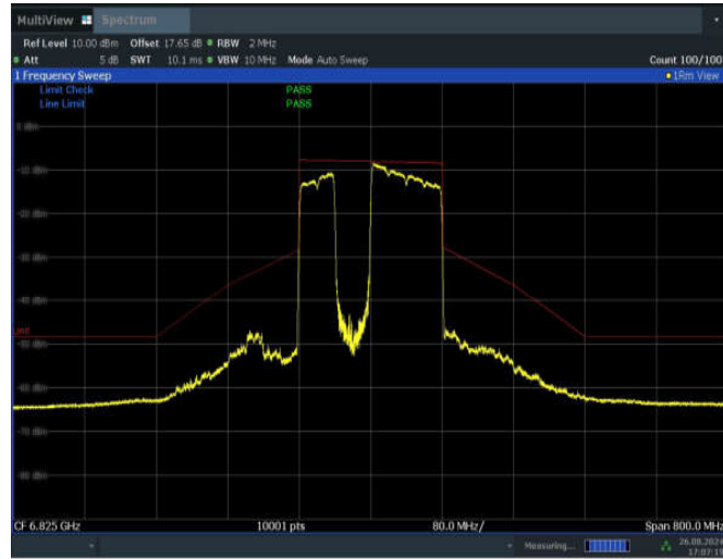
11BE160MIMO_Ant1_6825_996+484_Non-OFDMA_2
