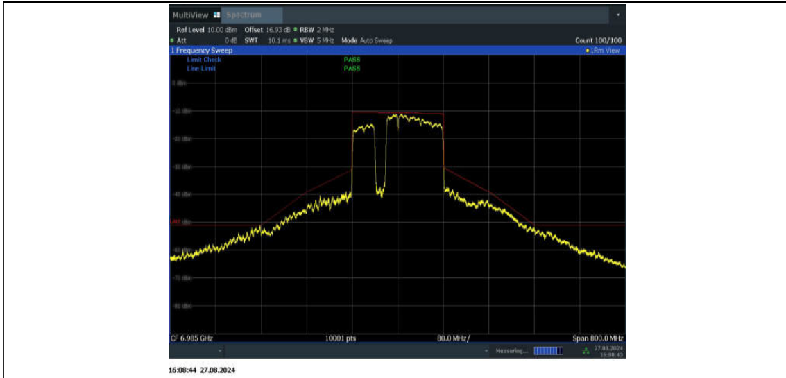
11BE160MIMO_Ant2_6985_996+484+242_Non-OFDMA_4
