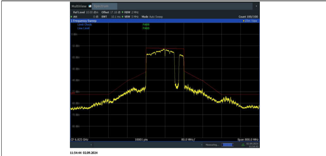
11BE160MIMO_Ant2_6825_996+484+242_Non-OFDMA_8
