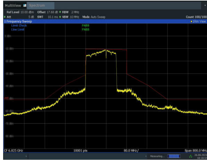
11BE160MIMO_Ant2_6825_996+484_Non-OFDMA_4
