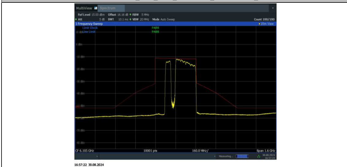
11BE320MIMO_Ant2_6105_2*996+484_Non-OFDMA_8
