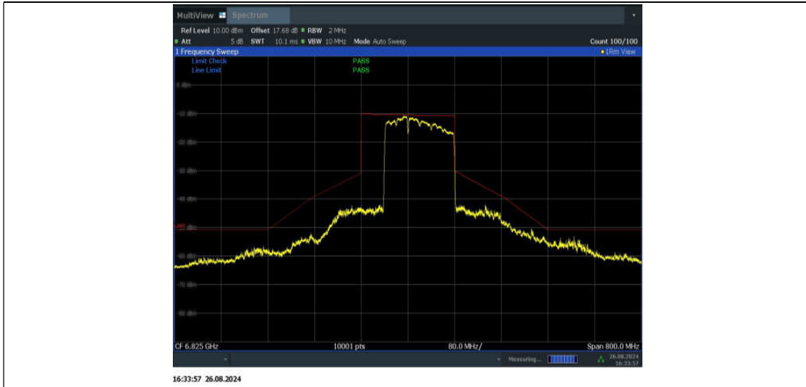
11BE160MIMO_Ant2_6825_996+484_Non-OFDMA_2
