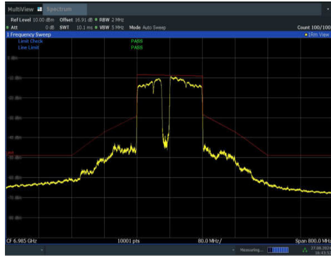
11BE160MIMO_Ant1_6985_996+484+242_Non-OFDMA_4
