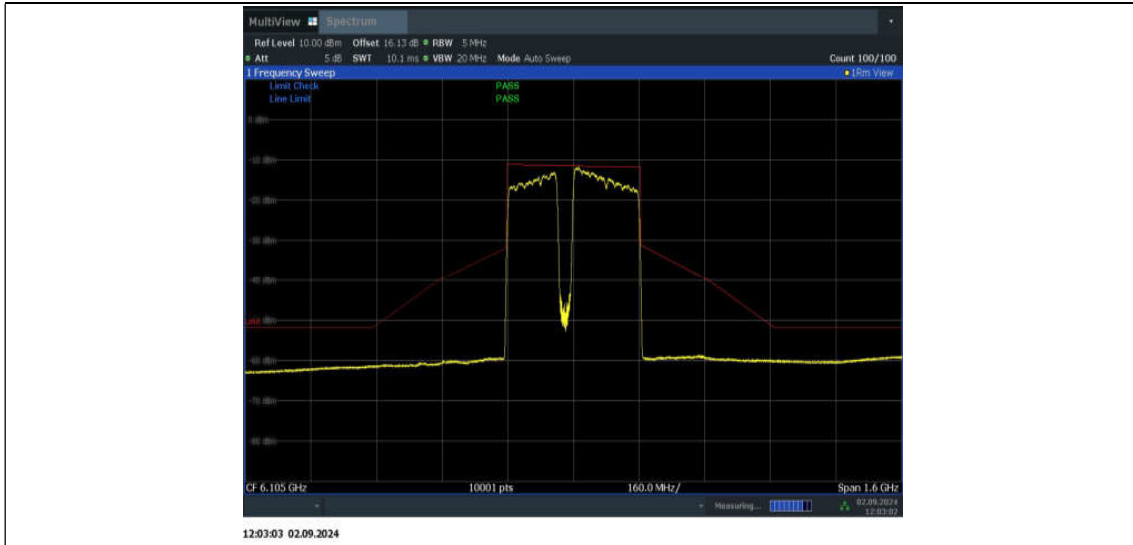
11BE320MIMO_Ant1_6105_3*996+484_Non-OFDMA_5
