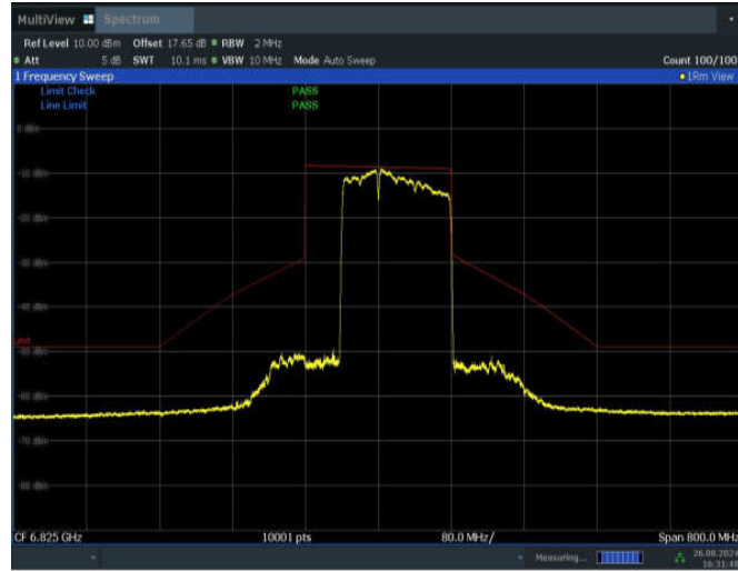
11BE160MIMO_Ant1_6825_996+484_Non-OFDMA_1
