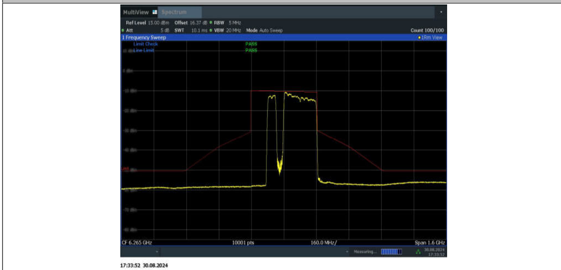
11BE320MIMO_Ant1_6265_2*996+484_Non-OFDMA_9
