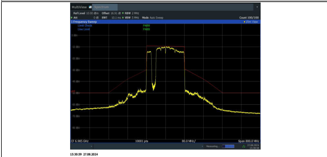
11BE160MIMO_Ant1_6985_996+484+242_Non-OFDMA_2
