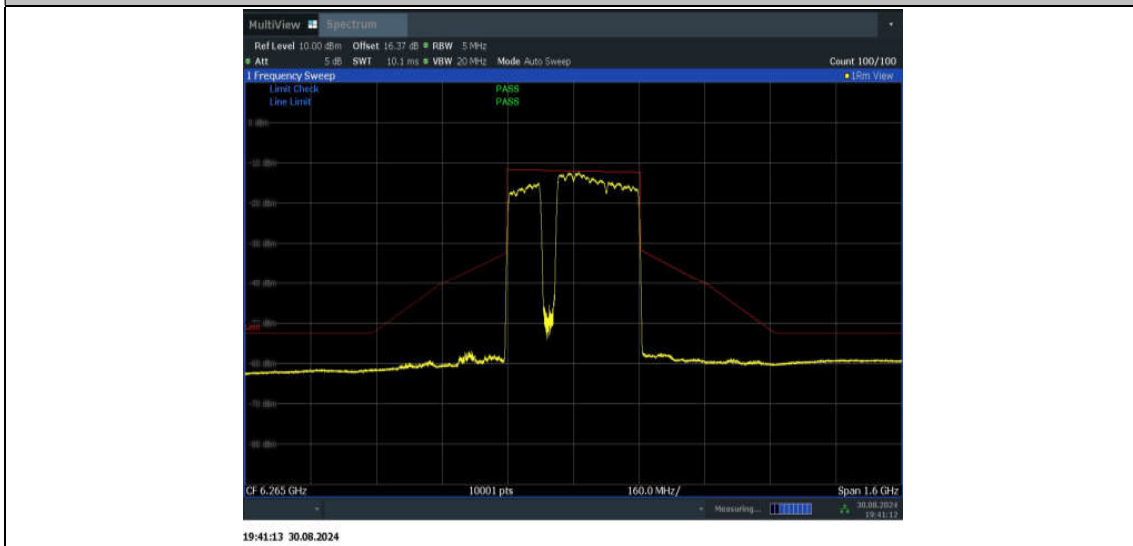
11BE320MIMO_Ant1_6265_3*996+484_Non-OFDMA_3
