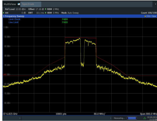
11BE160MIMO_Ant2_6825_996+484+242_Non-OFDMA_5
