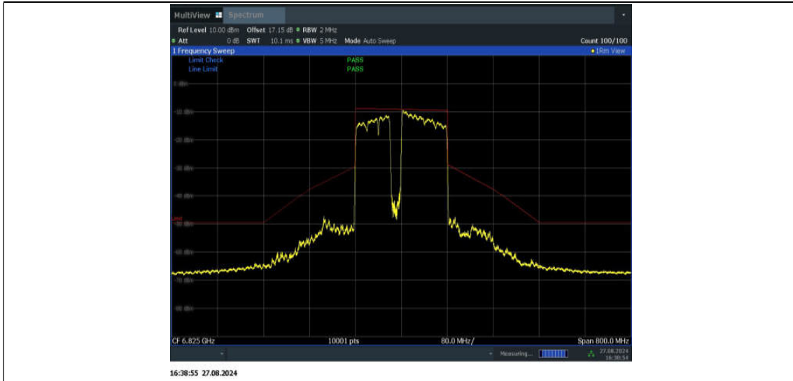
11BE160MIMO_Ant1_6825_996+484+242_Non-OFDMA_5
