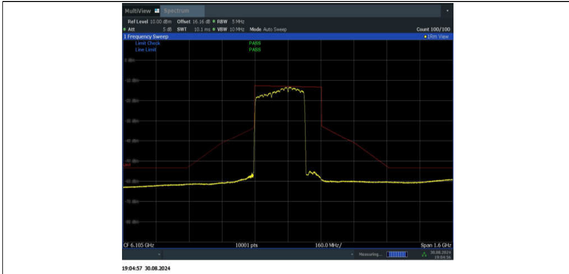
11BE320MIMO_Ant2_6105_3*996+484_Non-OFDMA_1
