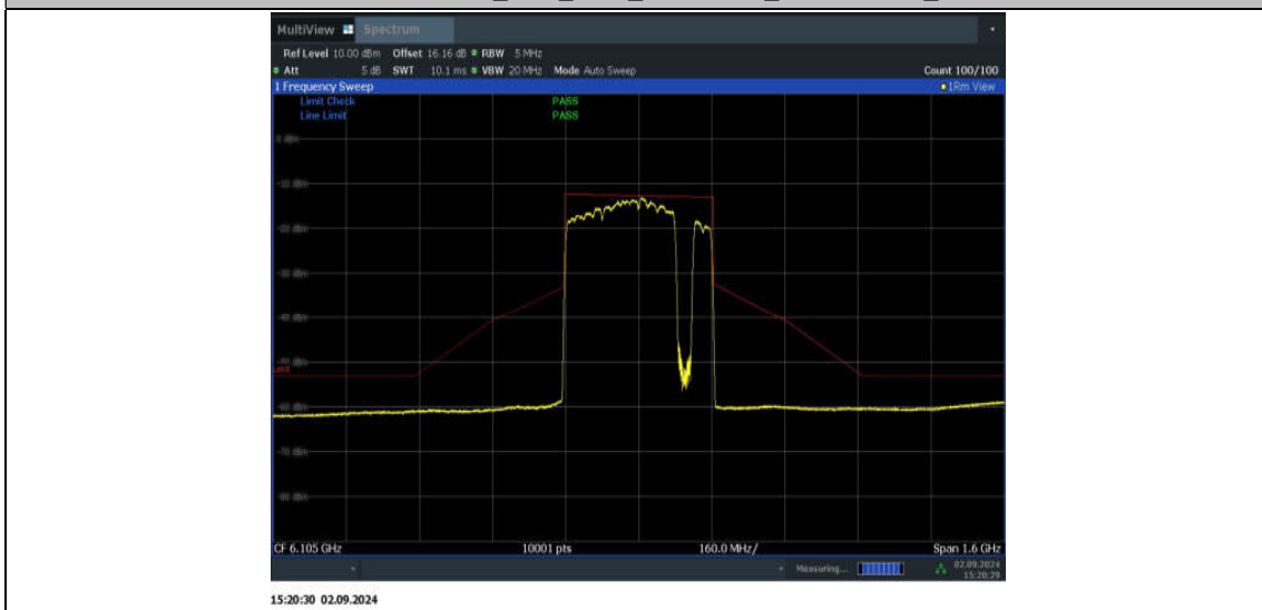
11BE320MIMO_Ant2_6105_3*996+484_Non-OFDMA_7
