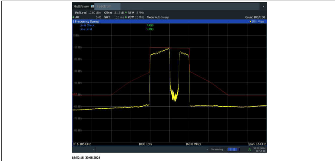
11BE320MIMO_Ant1_6105_3*996_Non-OFDMA_4
