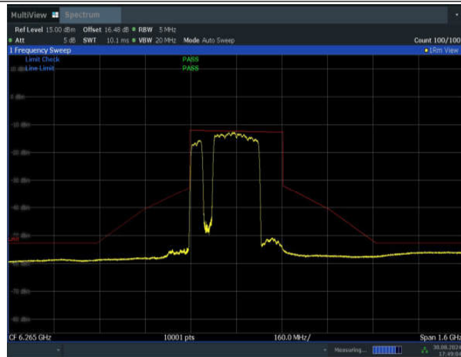
11BE320MIMO_Ant2_6265_2*996+484_Non-OFDMA_2
