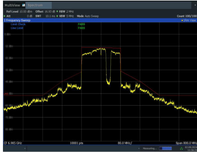
11BE160MIMO_Ant2_6985_996+484+242_Non-OFDMA_6
