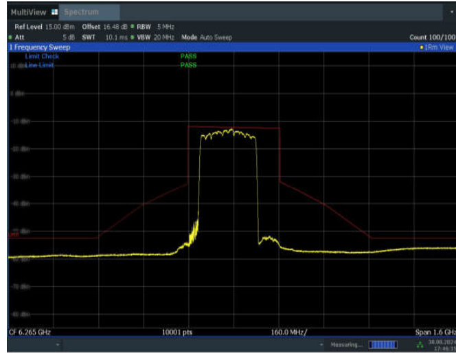
11BE320MIMO_Ant2_6265_2*996+484_Non-OFDMA_1
