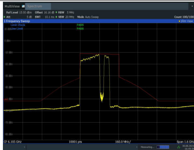
11BE320MIMO_Ant2_6105_2*996+484_Non-OFDMA_5
