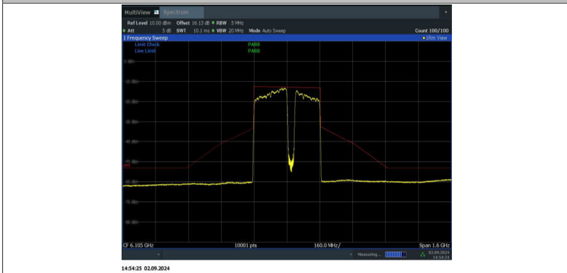
11BE320MIMO_Ant1_6105_3*996+484_Non-OFDMA_6
