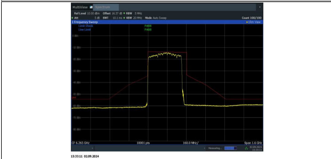
11BE320MIMO_Ant1_6265_3*996+484_Non-OFDMA_8
