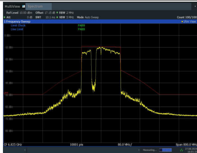
11BE160MIMO_Ant1_6825_996+484+242_Non-OFDMA_3
