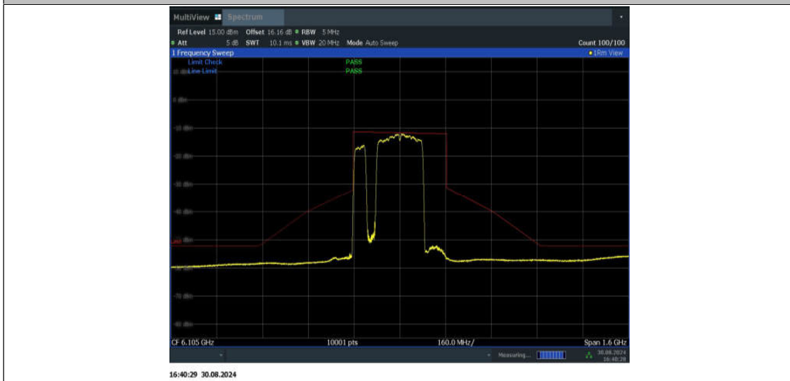
11BE320MIMO_Ant2_6105_2*996+484_Non-OFDMA_3
