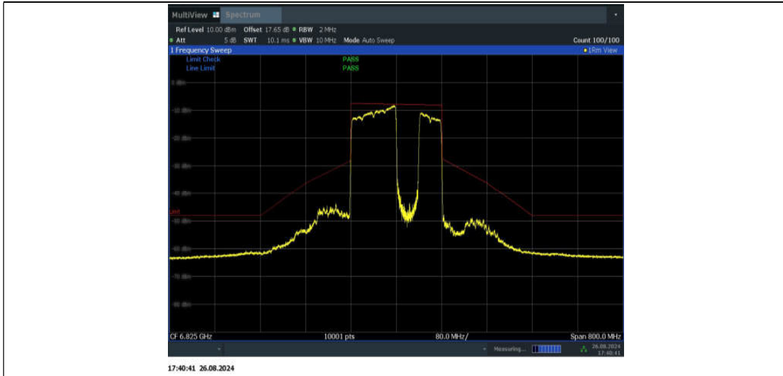
11BE160MIMO_Ant1_6825_996+484_Non-OFDMA_4
