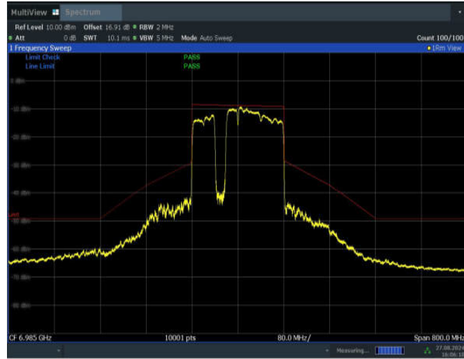
11BE160MIMO_Ant1_6985_996+484+242_Non-OFDMA_3
