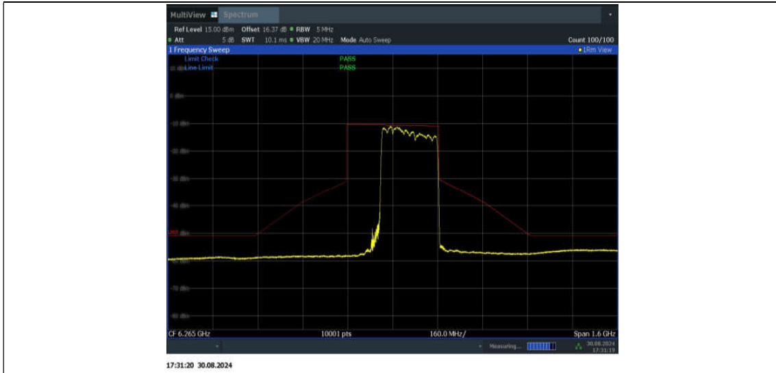
11BE320MIMO_Ant1_6265_2*996+484_Non-OFDMA_8
