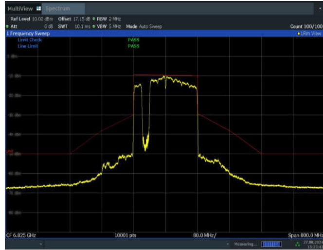
11BE160MIMO_Ant1_6825_996+484+242_Non-OFDMA_2
