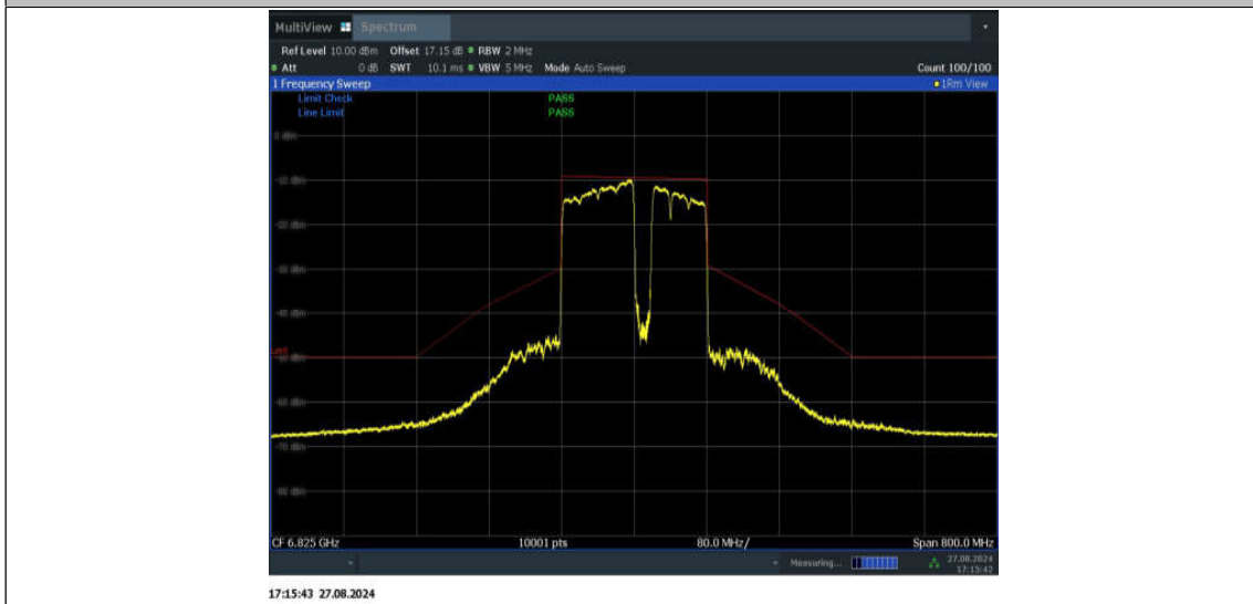
11BE160MIMO_Ant1_6825_996+484+242_Non-OFDMA_6
