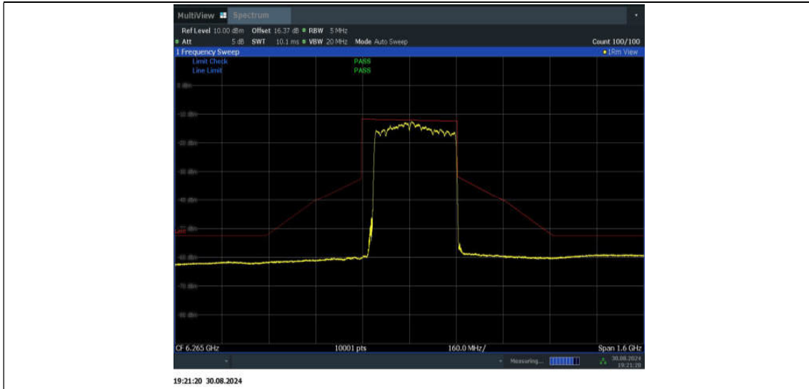
11BE320MIMO_Ant1_6265_3*996+484_Non-OFDMA_2
