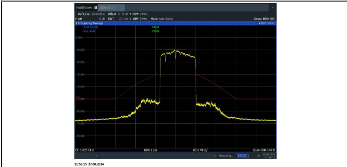
11BE160MIMO_Ant1_6825_996+484+242_Non-OFDMA_1
