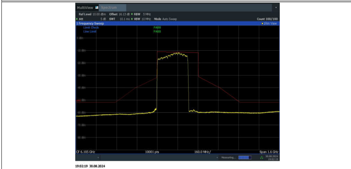
11BE320MIMO_Ant1_6105_3*996+484_Non-OFDMA_1
