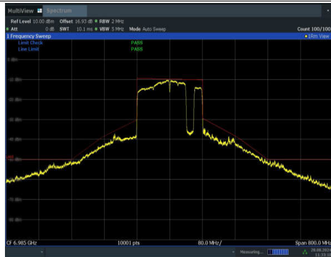
11BE160MIMO_Ant2_6985_996+484+242_Non-OFDMA_7
