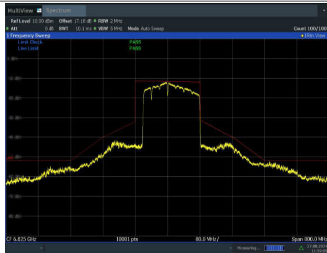
11BE160MIMO_Ant2_6825_996+484+242_Non-OFDMA_1
