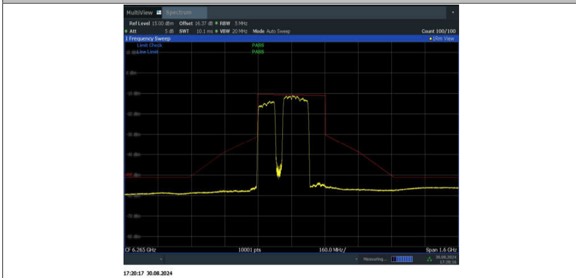
11BE320MIMO_Ant1_6265_2*996+484_Non-OFDMA_4
