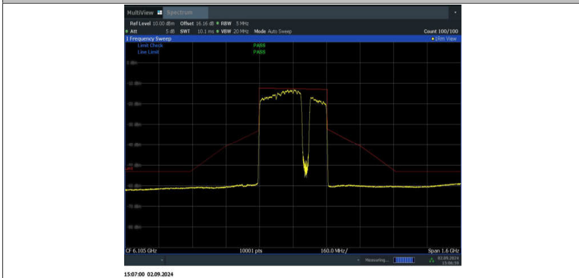
11BE320MIMO_Ant2_6105_3*996+484_Non-OFDMA_7
