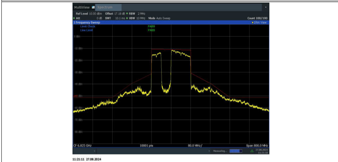
11BE160MIMO_Ant2_6825_996+484_Non-OFDMA_3
