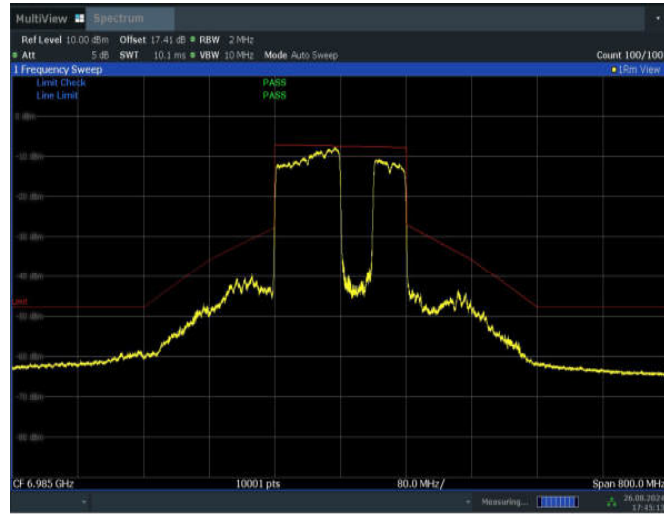
11BE160MIMO_Ant1_6985_996+484_Non-OFDMA_3
