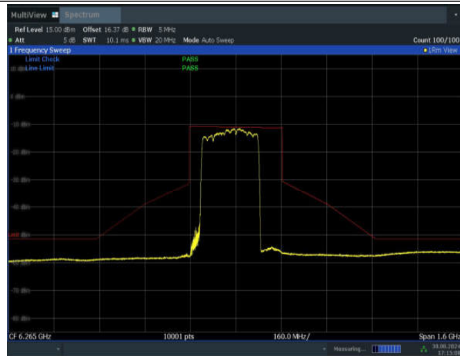
11BE320MIMO_Ant1_6265_2*996+484_Non-OFDMA_1
