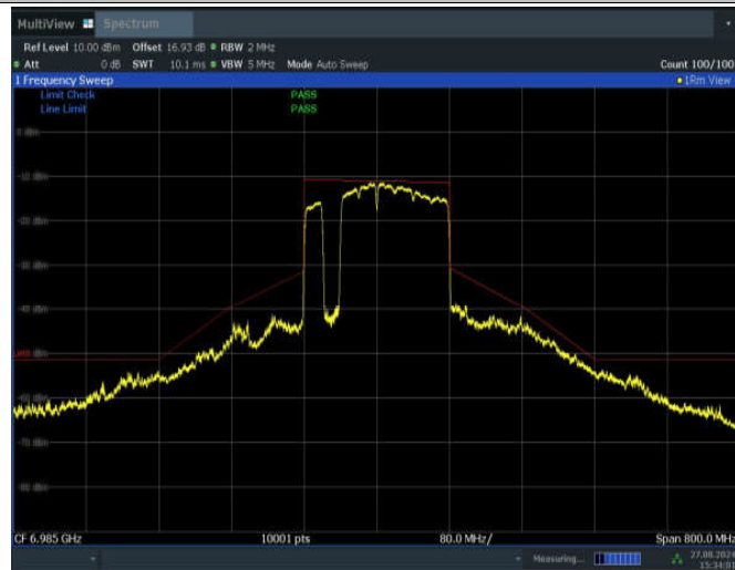
11BE160MIMO_Ant2_6985_996+484+242_Non-OFDMA_2
