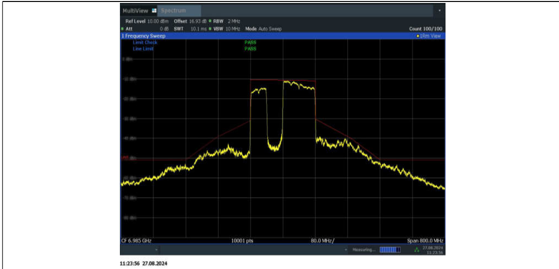
11BE160MIMO_Ant2_6985_996+484_Non-OFDMA_3
