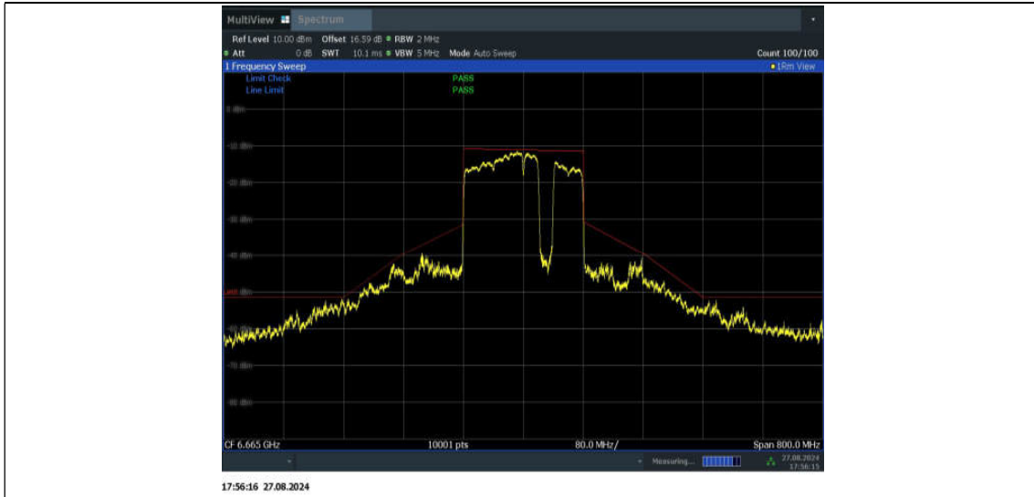
11BE160MIMO_Ant2_6665_996+484+242_Non-OFDMA_7
