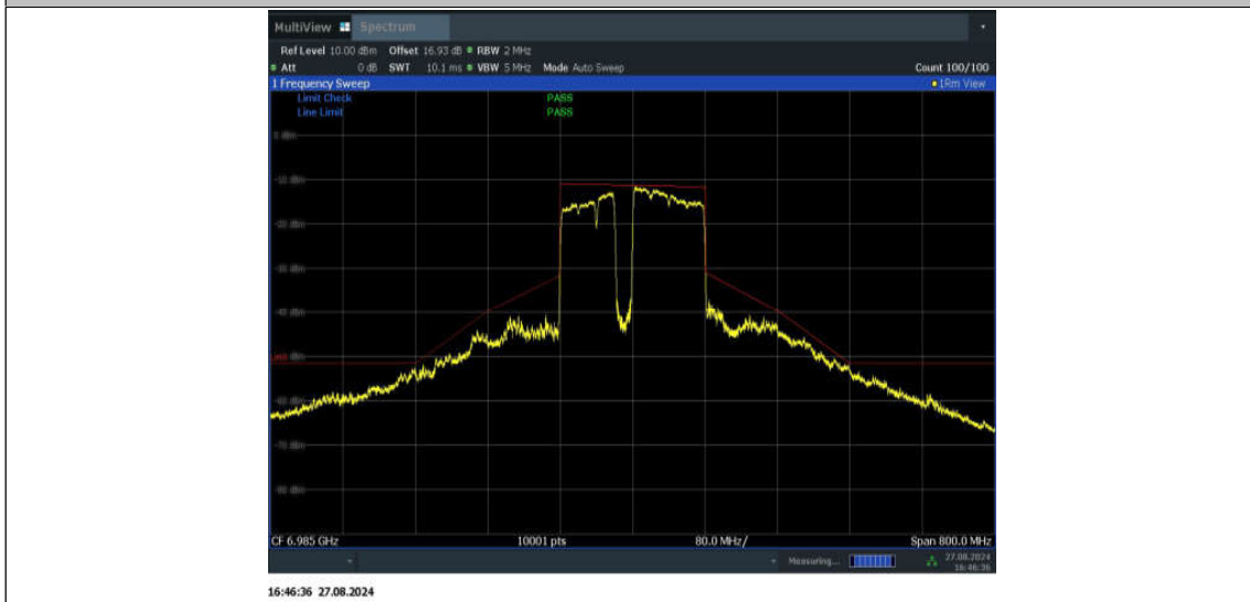
11BE160MIMO_Ant2_6985_996+484+242_Non-OFDMA_5
