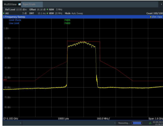
11BE320MIMO_Ant2_6105_3*996+484_Non-OFDMA_8
