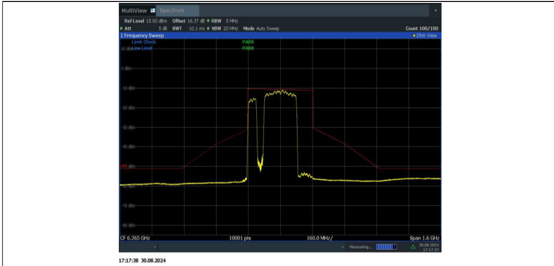
11BE320MIMO_Ant1_6265_2*996+484_Non-OFDMA_3
