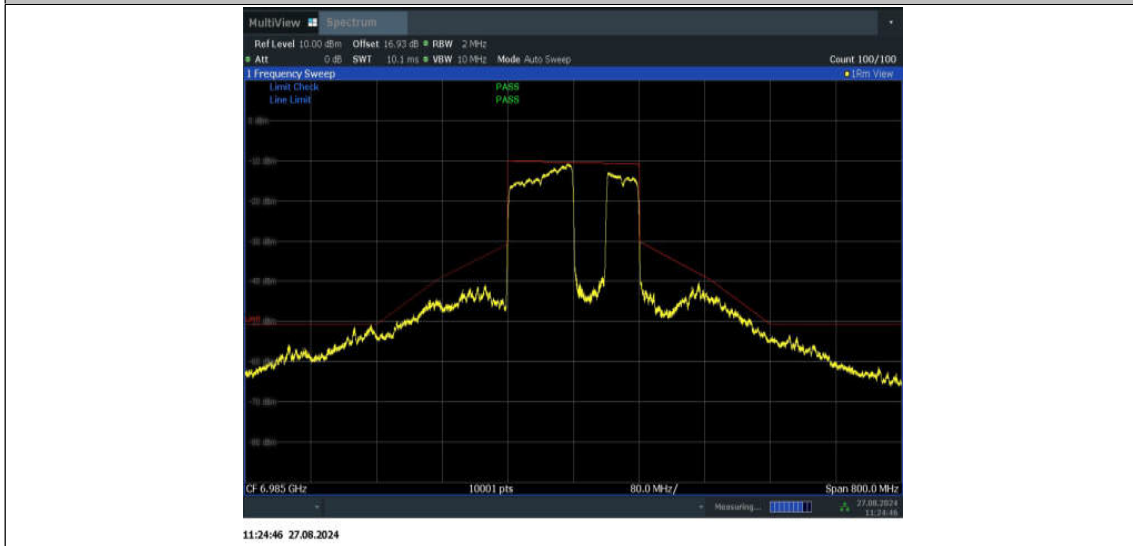
11BE160MIMO_Ant2_6985_996+484_Non-OFDMA_4
