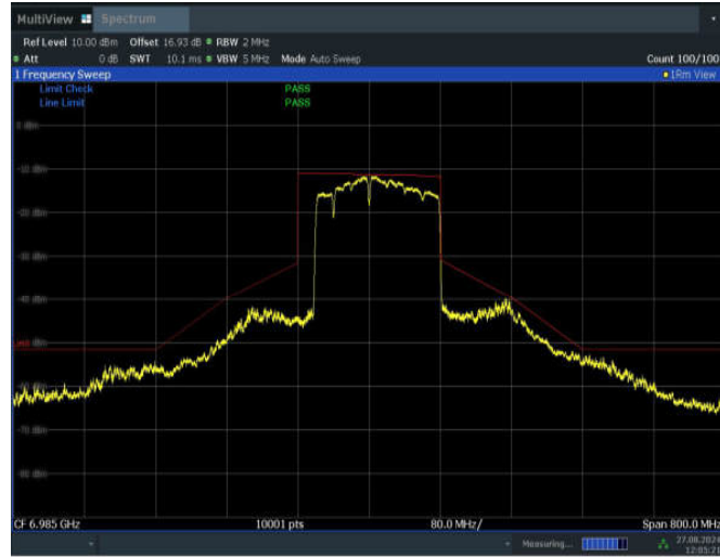
11BE160MIMO_Ant2_6985_996+484+242_Non-OFDMA_1
