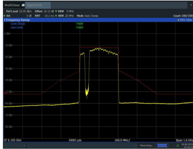
11BE320MIMO_Ant1_6105_3*996+484_Non-OFDMA_2
