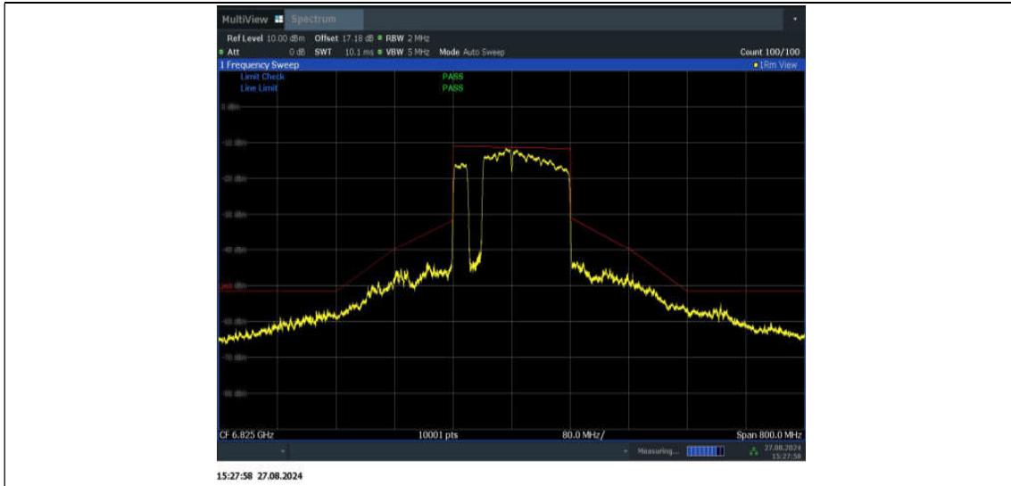
11BE160MIMO_Ant2_6825_996+484+242_Non-OFDMA_3
