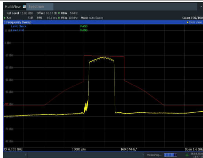
11BE320MIMO_Ant1_6105_2*996+484_Non-OFDMA_4
