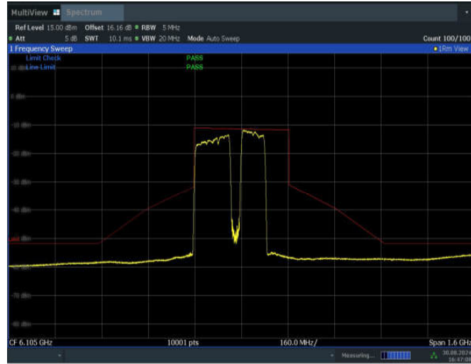
11BE320MIMO_Ant2_6105_2*996+484_Non-OFDMA_4
