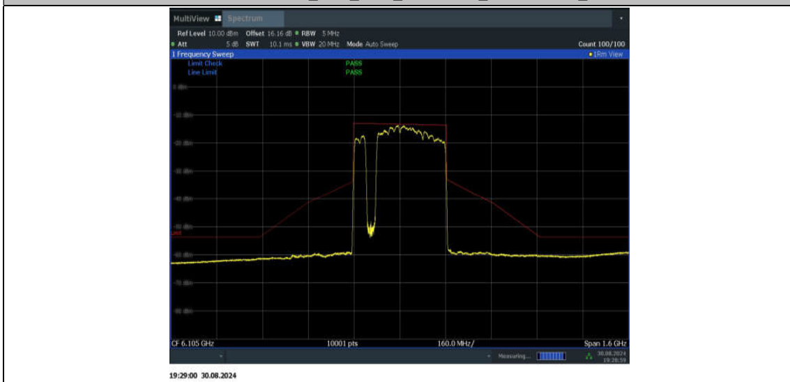
11BE320MIMO_Ant2_6105_3*996+484_Non-OFDMA_2
