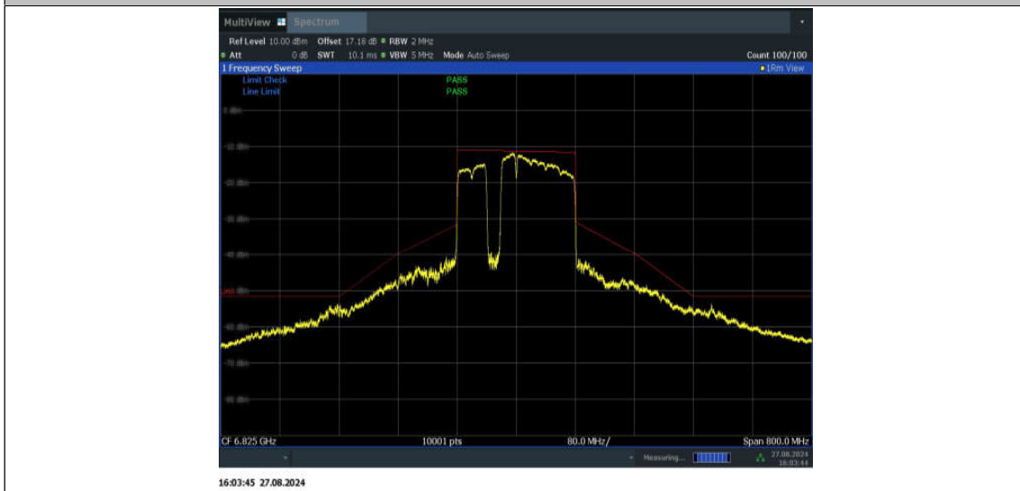
11BE160MIMO_Ant2_6825_996+484+242_Non-OFDMA_4
