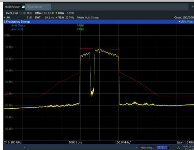
11BE320MIMO_Ant1_6105_3*996+484_Non-OFDMA_3
