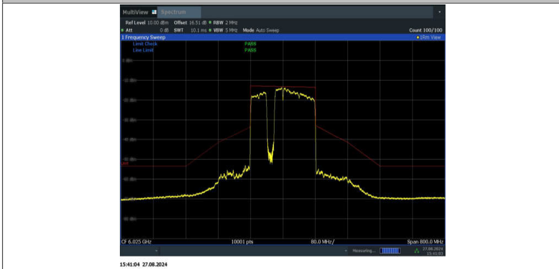
11BE160MIMO_Ant2_6025_996+484+242_Non-OFDMA_4
