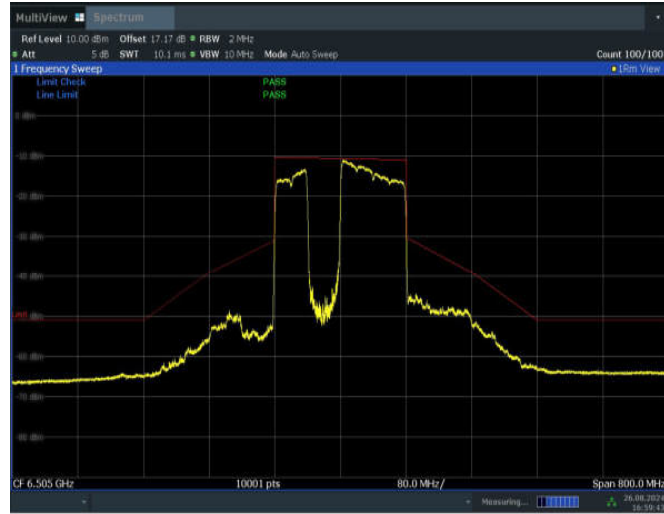
11BE160MIMO_Ant2_6505_996+484_Non-OFDMA_2
