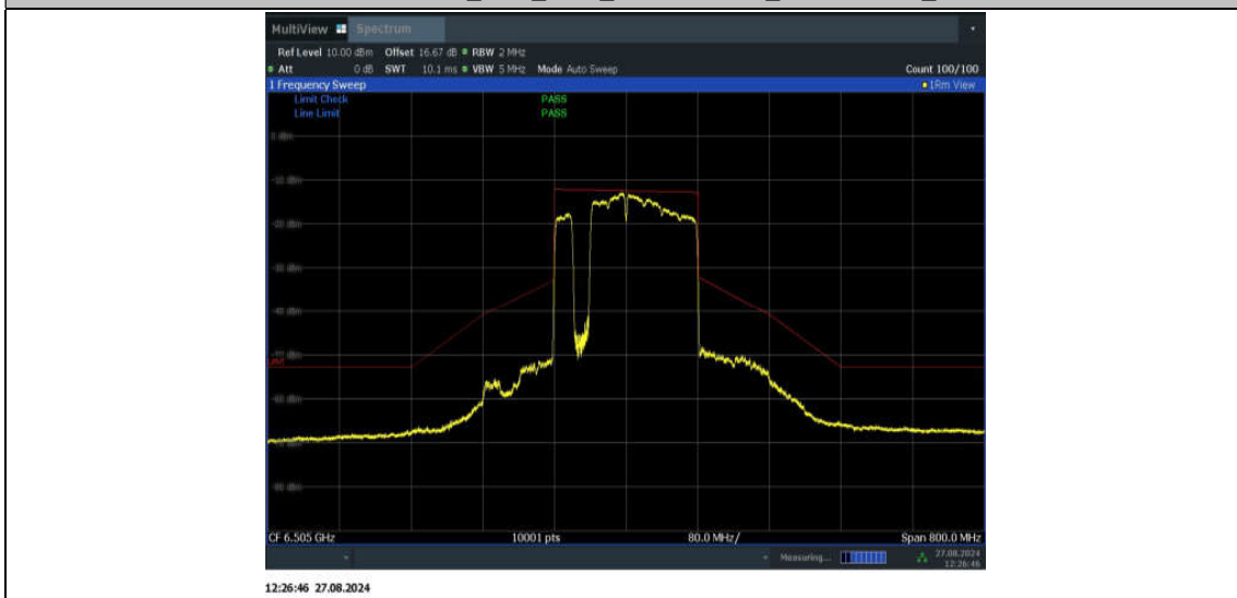
11BE160MIMO_Ant2_6505_996+484+242_Non-OFDMA_2
