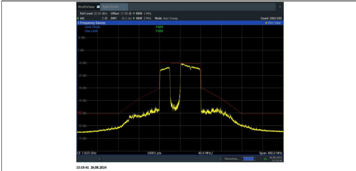
11BE80MIMO_Ant2_7025_484+242_Non-OFDMA_3
