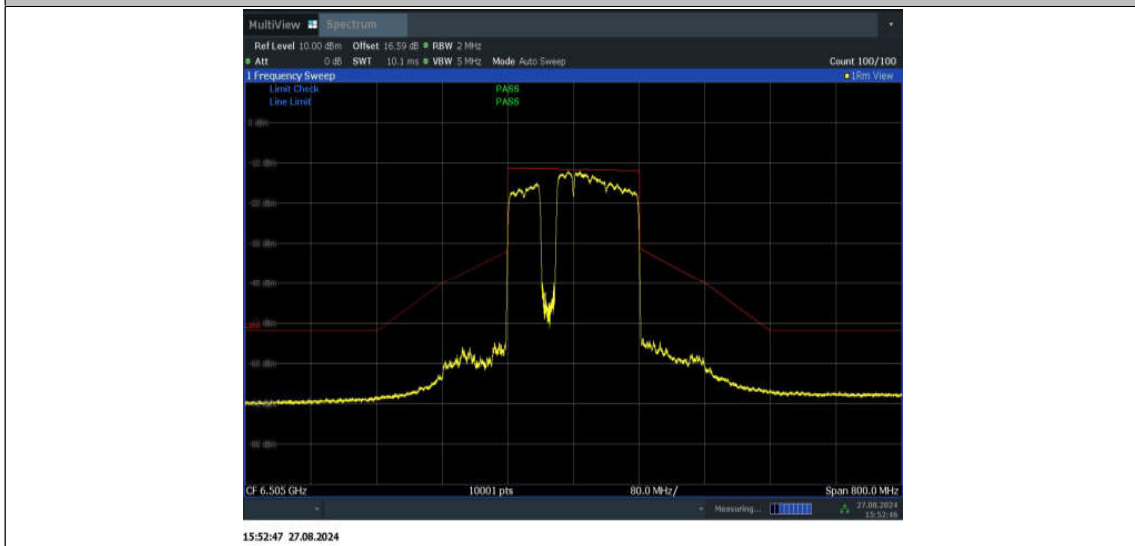
11BE160MIMO_Ant1_6505_996+484+242_Non-OFDMA_4
