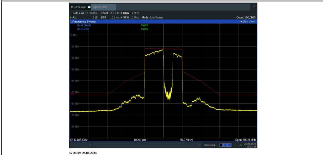
11BE160MIMO_Ant2_6185_996+484_Non-OFDMA_4
