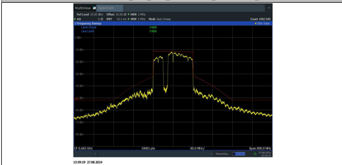
11BE160MIMO_Ant2_6665_996+484+242_Non-OFDMA_3
