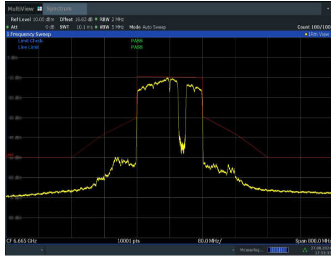
11BE160MIMO_Ant1_6665_996+484+242_Non-OFDMA_6
