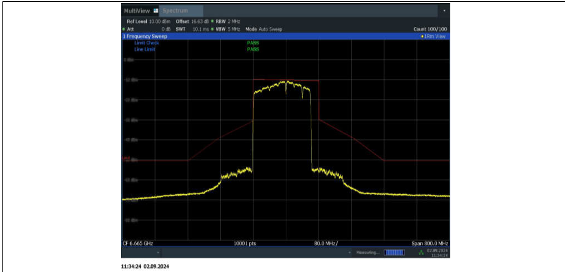
11BE160MIMO_Ant2_6665_996+484_Non-OFDMA_1
