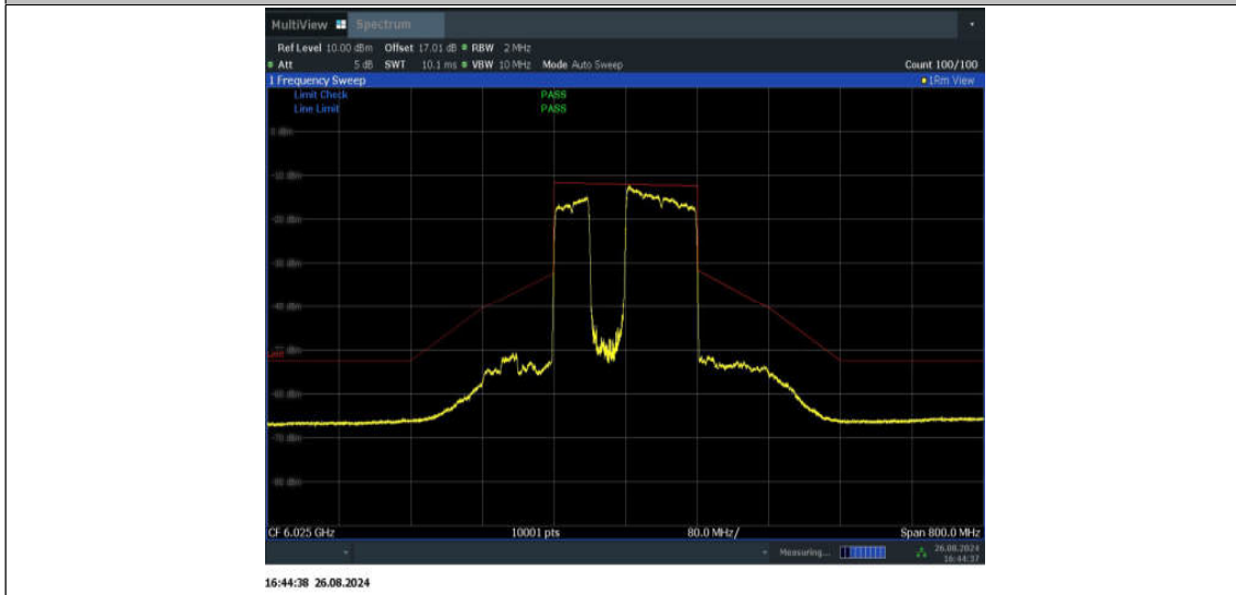
11BE160MIMO_Ant2_6025_996+484_Non-OFDMA_3
