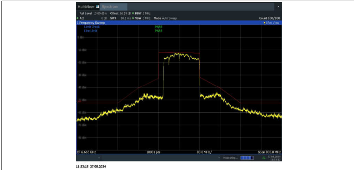
11BE160MIMO_Ant2_6665_996+484+242_Non-OFDMA_2
