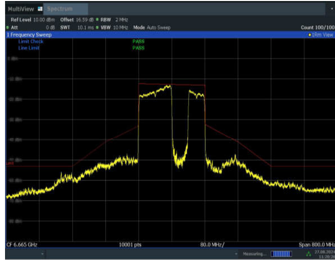
11BE160MIMO_Ant2_6665_996+484_Non-OFDMA_3
