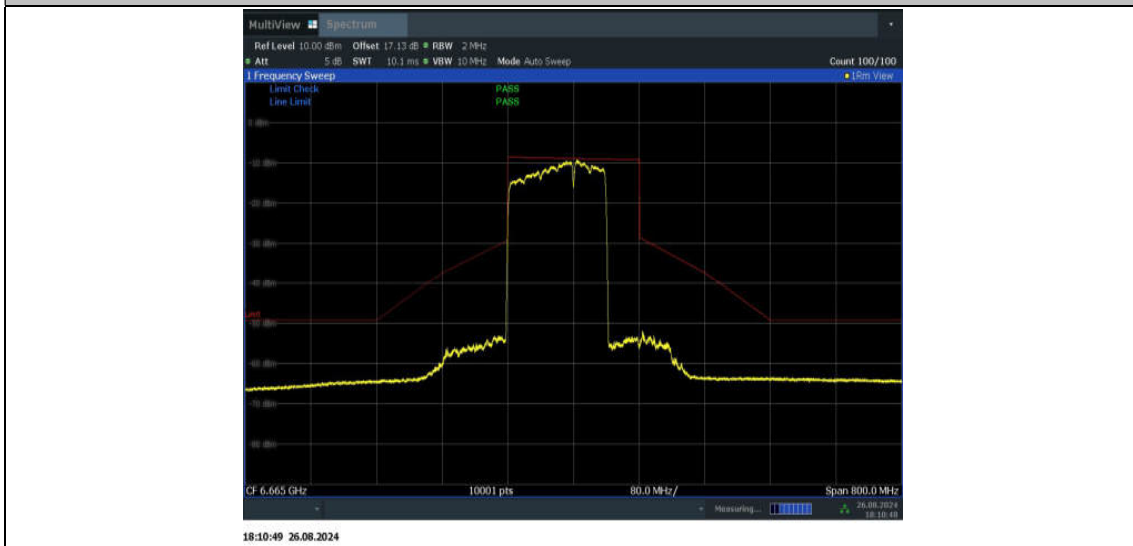
11BE160MIMO_Ant1_6665_996+484_Non-OFDMA_4
