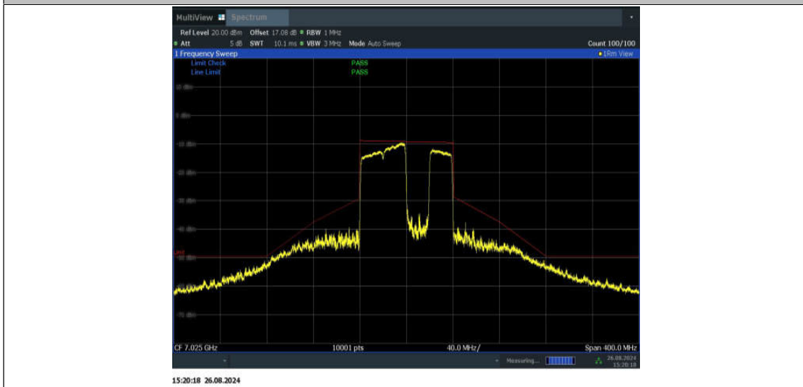
11BE80MIMO_Ant2_7025_484+242_Non-OFDMA_4
