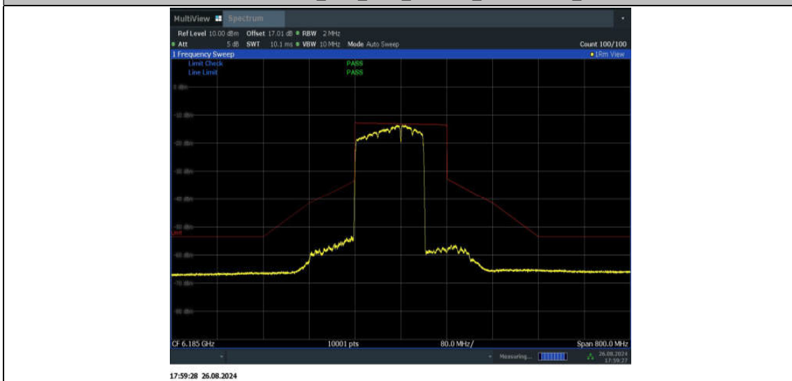
11BE160MIMO_Ant2_6185_996+484_Non-OFDMA_4
