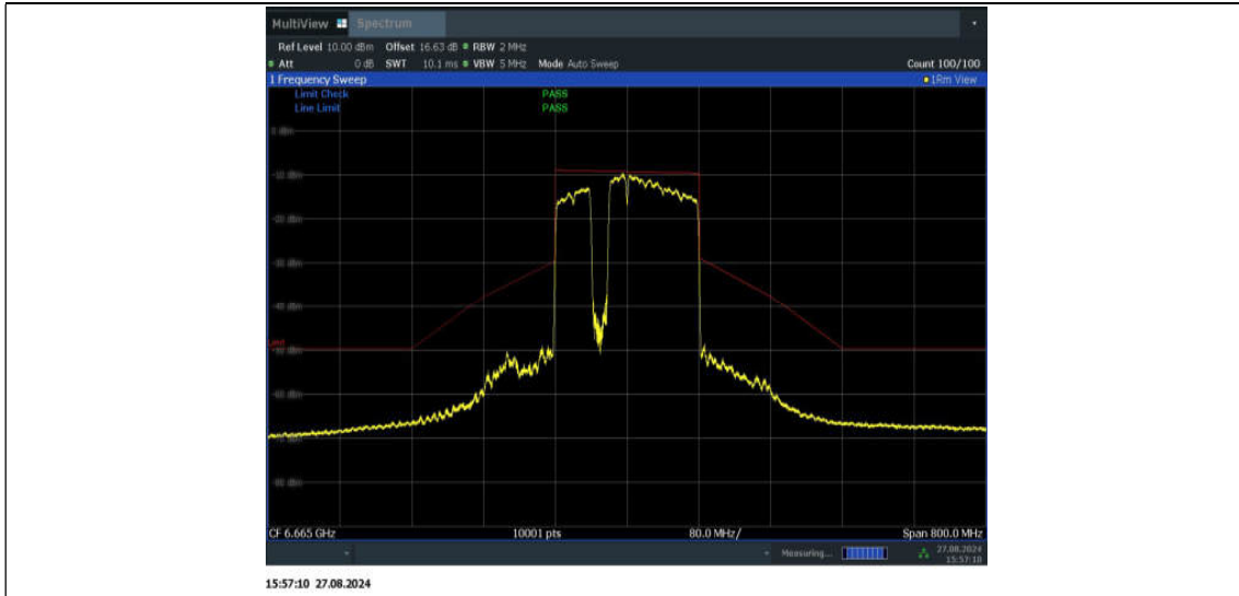
11BE160MIMO_Ant1_6665_996+484+242_Non-OFDMA_4
