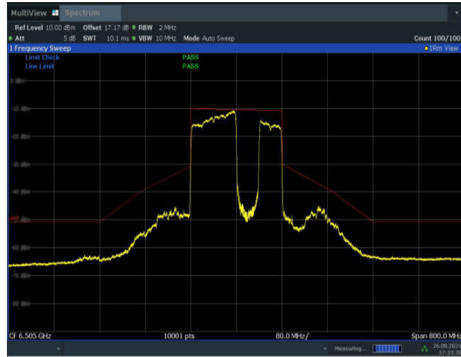
11BE160MIMO_Ant2_6505_996+484_Non-OFDMA_3
