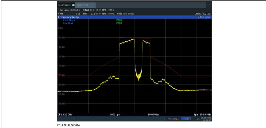
11BE160MIMO_Ant1_6025_996+484_Non-OFDMA_4
