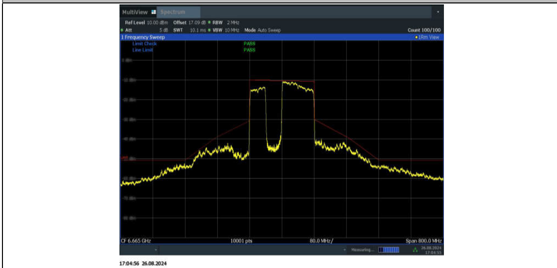
11BE160MIMO_Ant2_6665_996+484_Non-OFDMA_2
