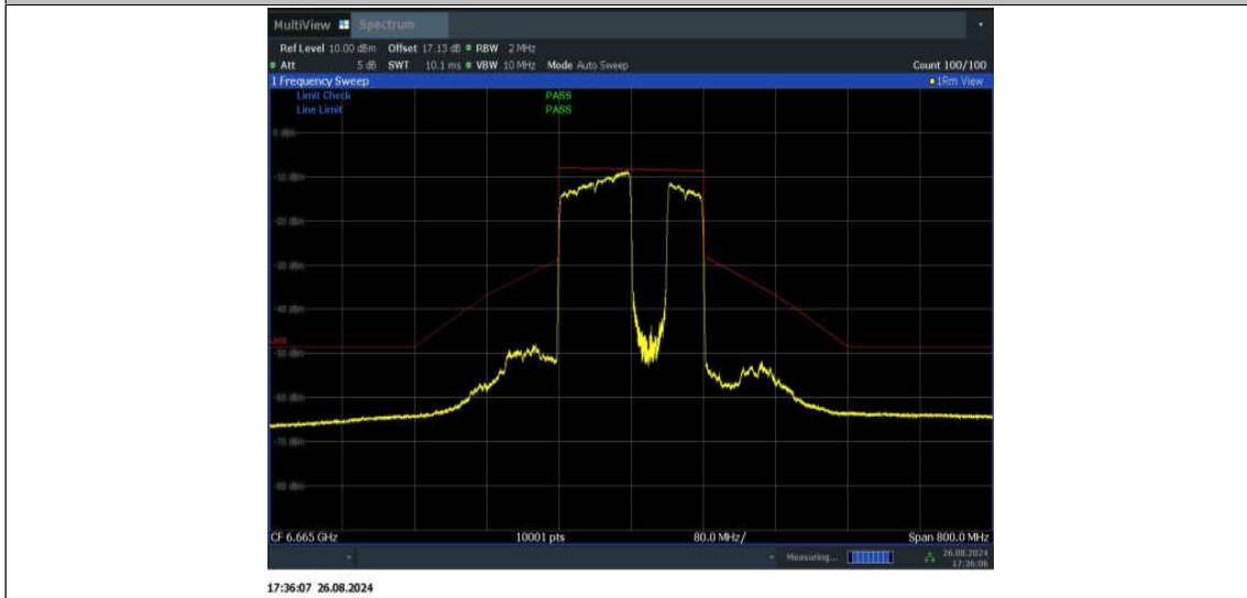
11BE160MIMO_Ant1_6665_996+484_Non-OFDMA_4
