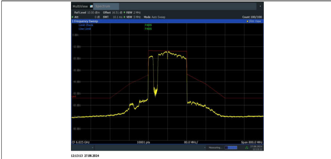
11BE160MIMO_Ant2_6025_996+484+242_Non-OFDMA_3
