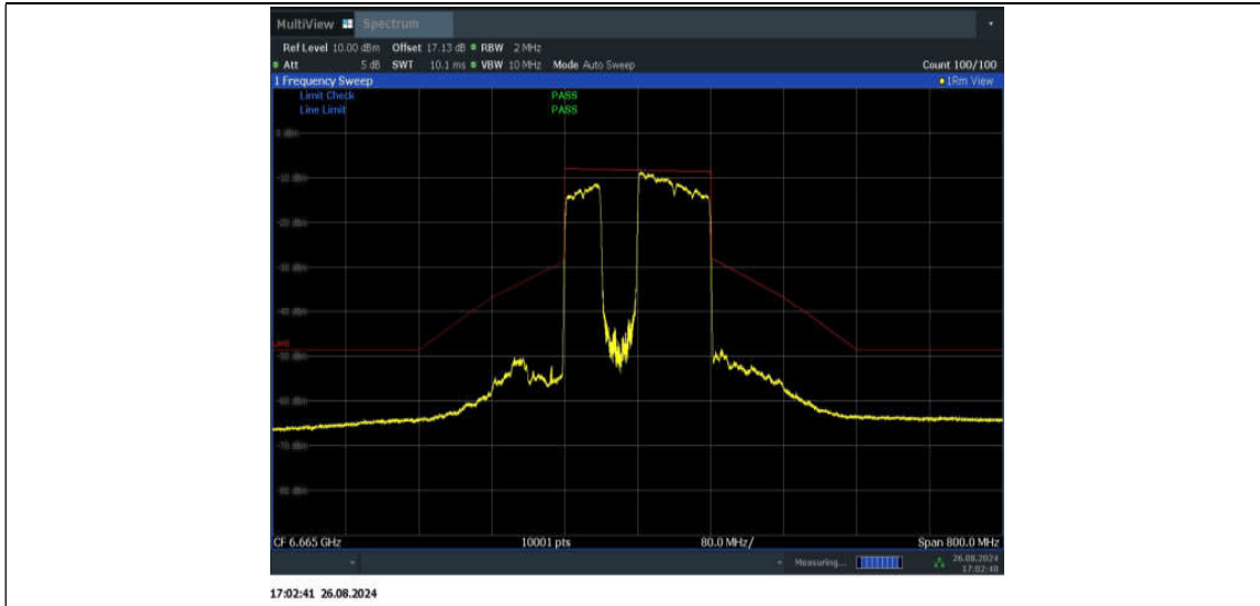
11BE160MIMO_Ant1_6665_996+484_Non-OFDMA_3
