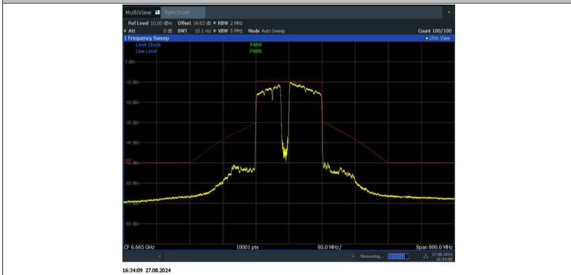
11BE160MIMO_Ant1_6665_996+484+242_Non-OFDMA_5
