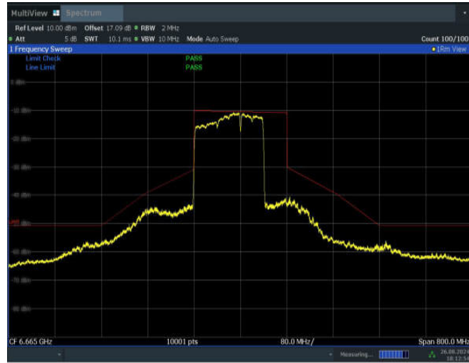
11BE160MIMO_Ant2_6665_996+484_Non-OFDMA_4
