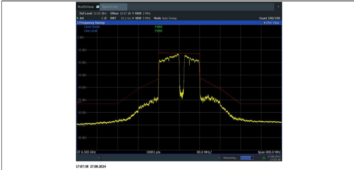
11BE160MIMO_Ant2_6505_996+484+242_Non-OFDMA_6
