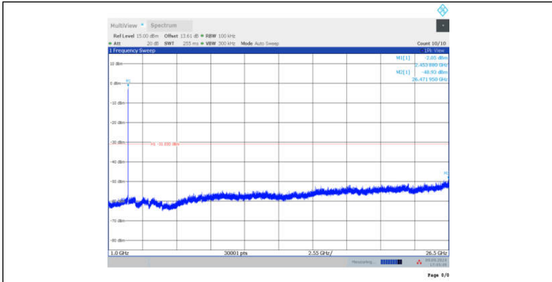
11AX20MIMO_Ant12_2462_106Tone_RU54_0~Reference
