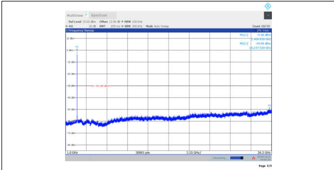
11BE20MIMO_Ant12_2412_106Tone_RU54_0~Reference
