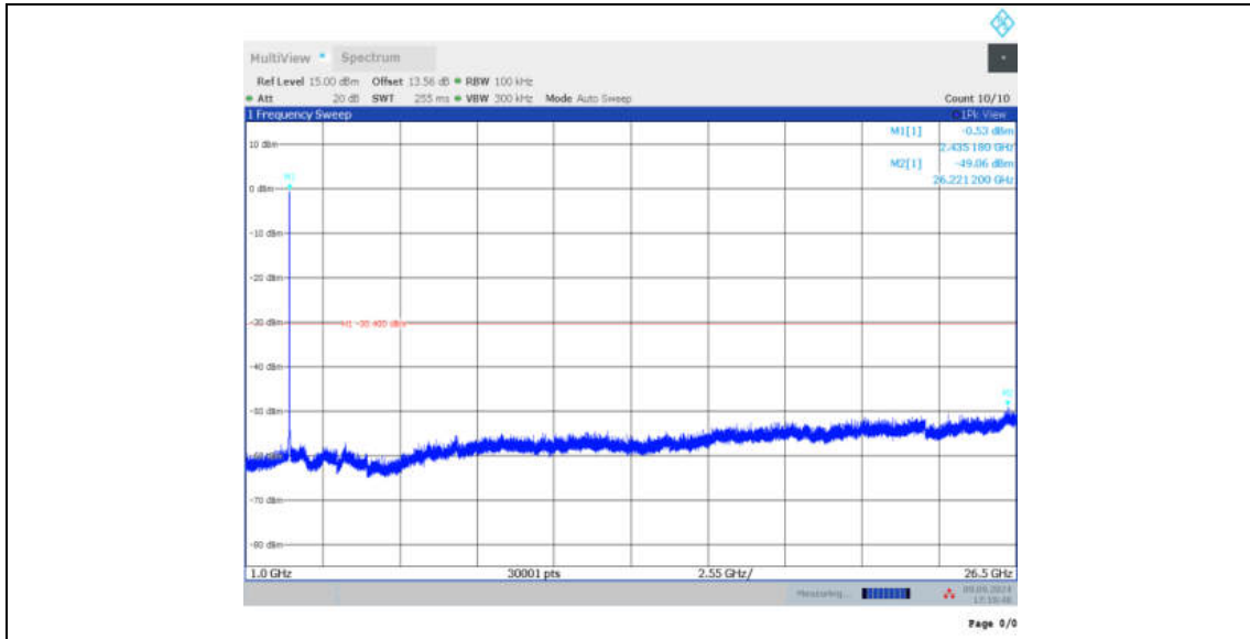
11AX20MIMO_Ant12_2437_106Tone_RU54_0~Reference
