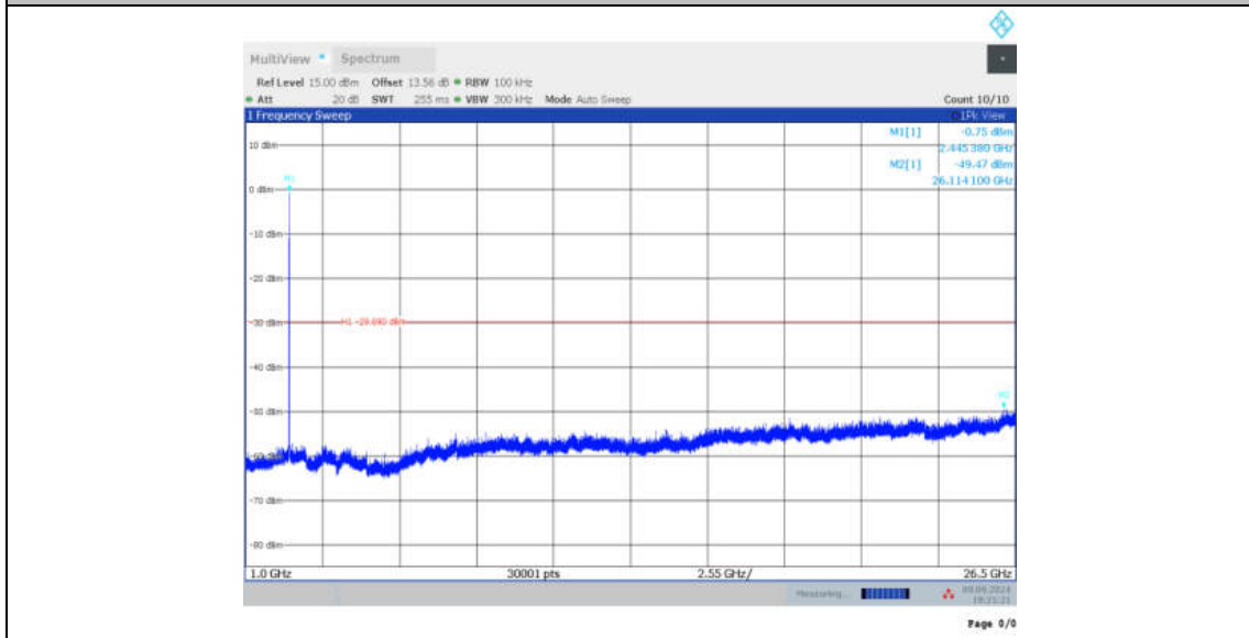
11BE20MIMO_Ant12_2437_52Tone_RU37_0~Reference
