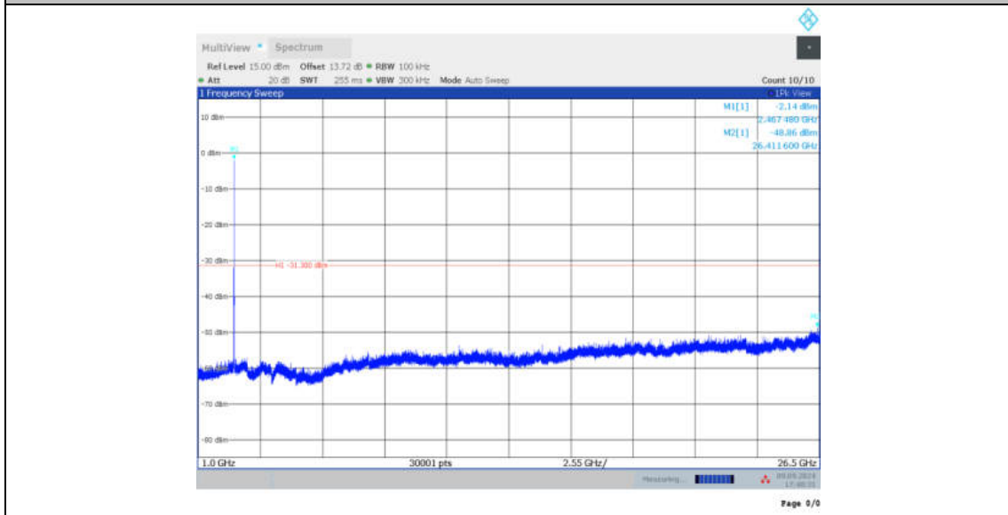
11AX20MIMO_Ant7_2462_106Tone_RU53_0~Reference
