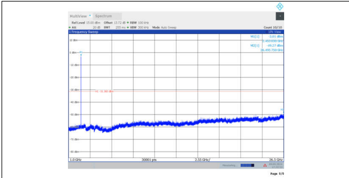
11AX20MIMO_Ant7_2462_26Tone_RU8_0~Reference
