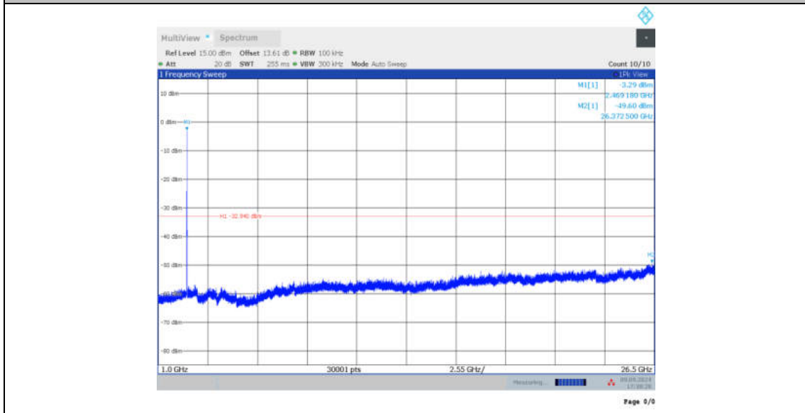
11AX20MIMO_Ant12_2462_106Tone_RU53_0~Reference
