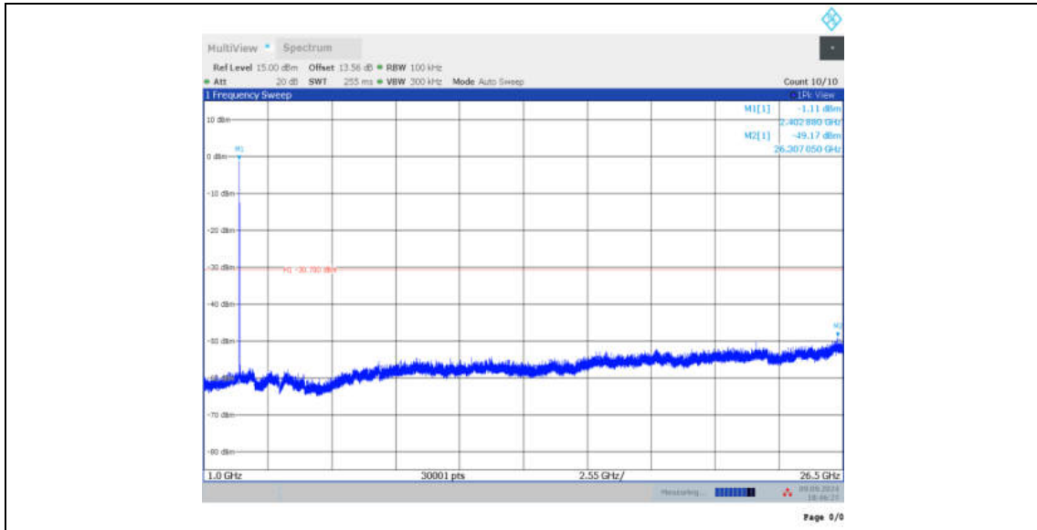
11BE20MIMO_Ant12_2412_26Tone_RU8_0~Reference
