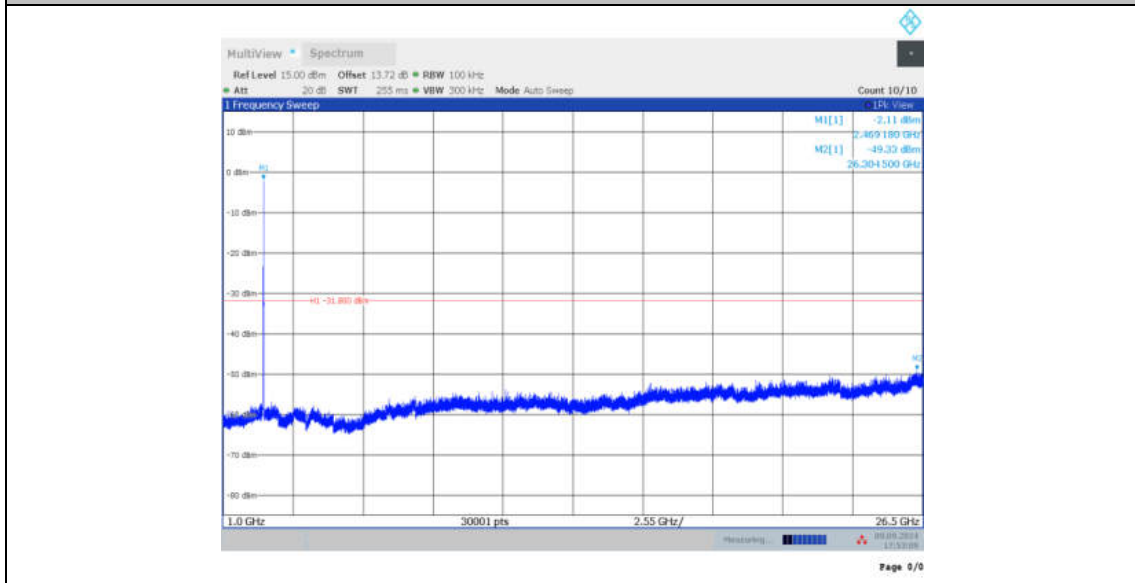
11BE20MIMO_Ant12_2412_26Tone_RU0_0~Reference
