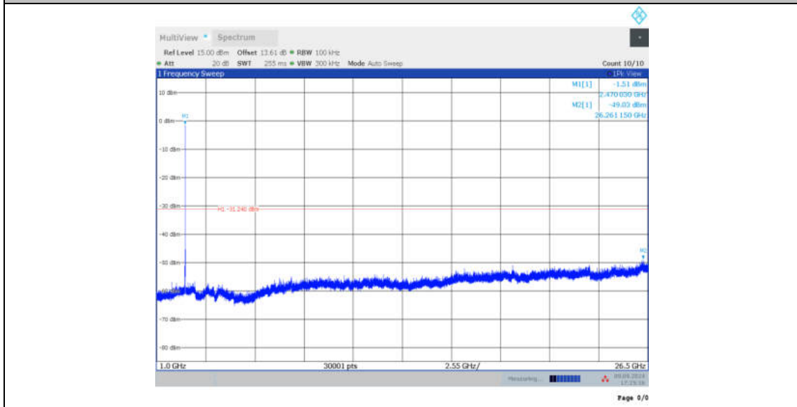
11AX20MIMO_Ant12_2462_52Tone_RU37_0~Reference
