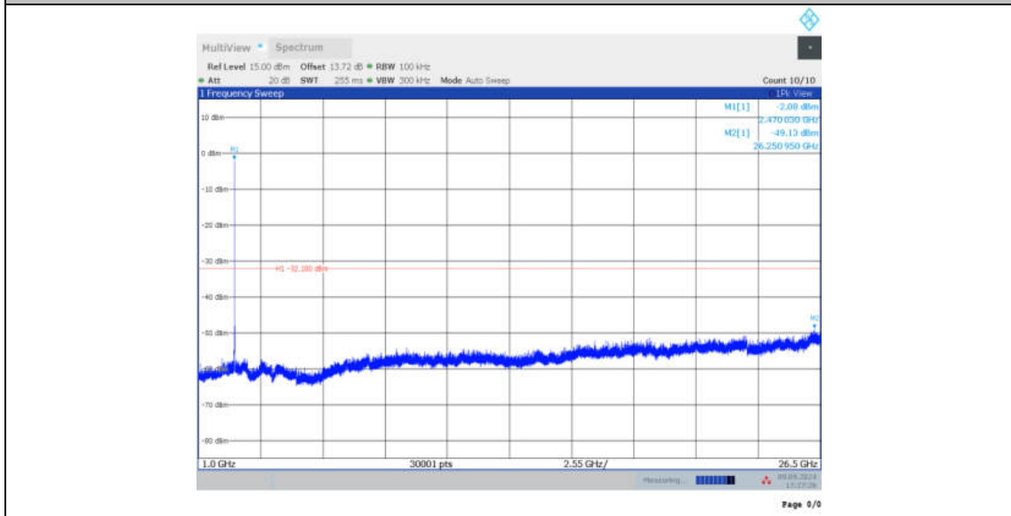
11AX20MIMO_Ant7_2462_52Tone_RU37_0~Reference
