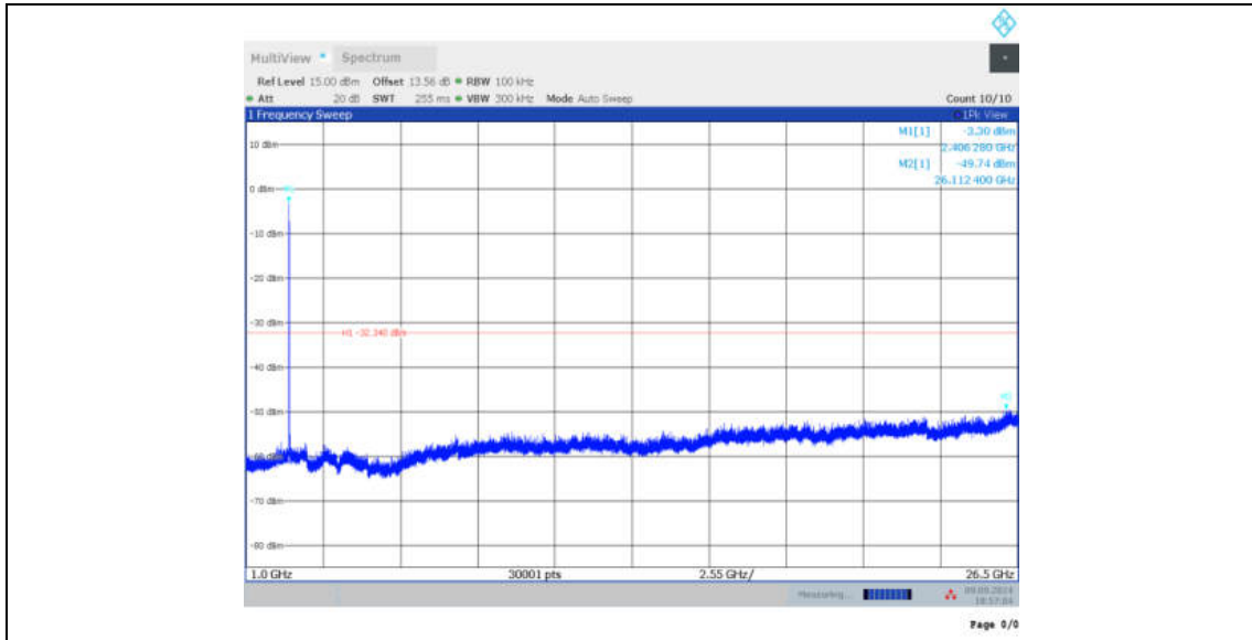
11BE20MIMO_Ant12_2412_52Tone_RU40_0~Reference
