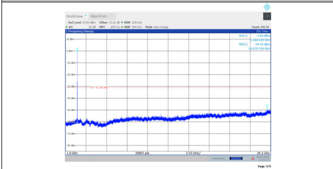
11AX20MIMO_Ant7_2462_26Tone_RU0_0~Reference
