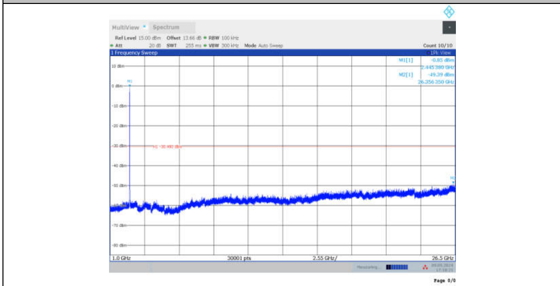
11AX20MIMO_Ant12_2462_26Tone_RU0_0~Reference
