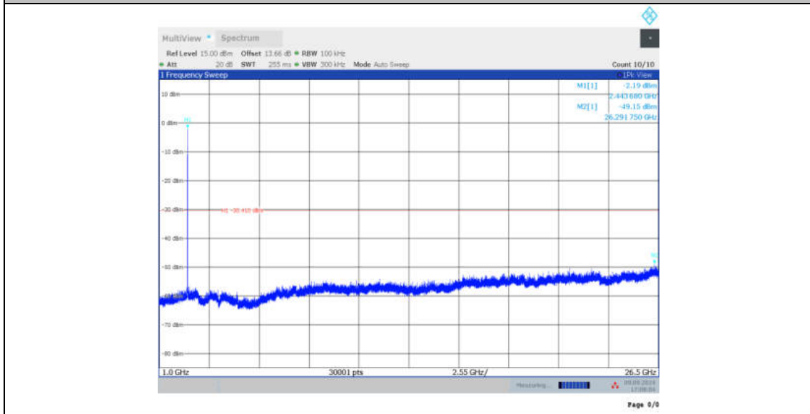
11AX20MIMO_Ant7_2437_106Tone_RU53_0~Reference
