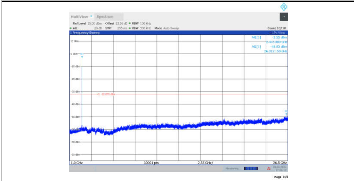
11AX20MIMO_Ant12_2437_106Tone_RU53_0~Reference
