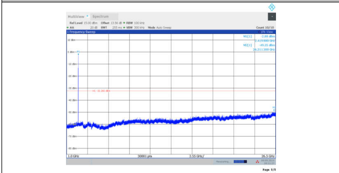
11BE20MIMO_Ant12_2412_52Tone_RU37_0~Reference
