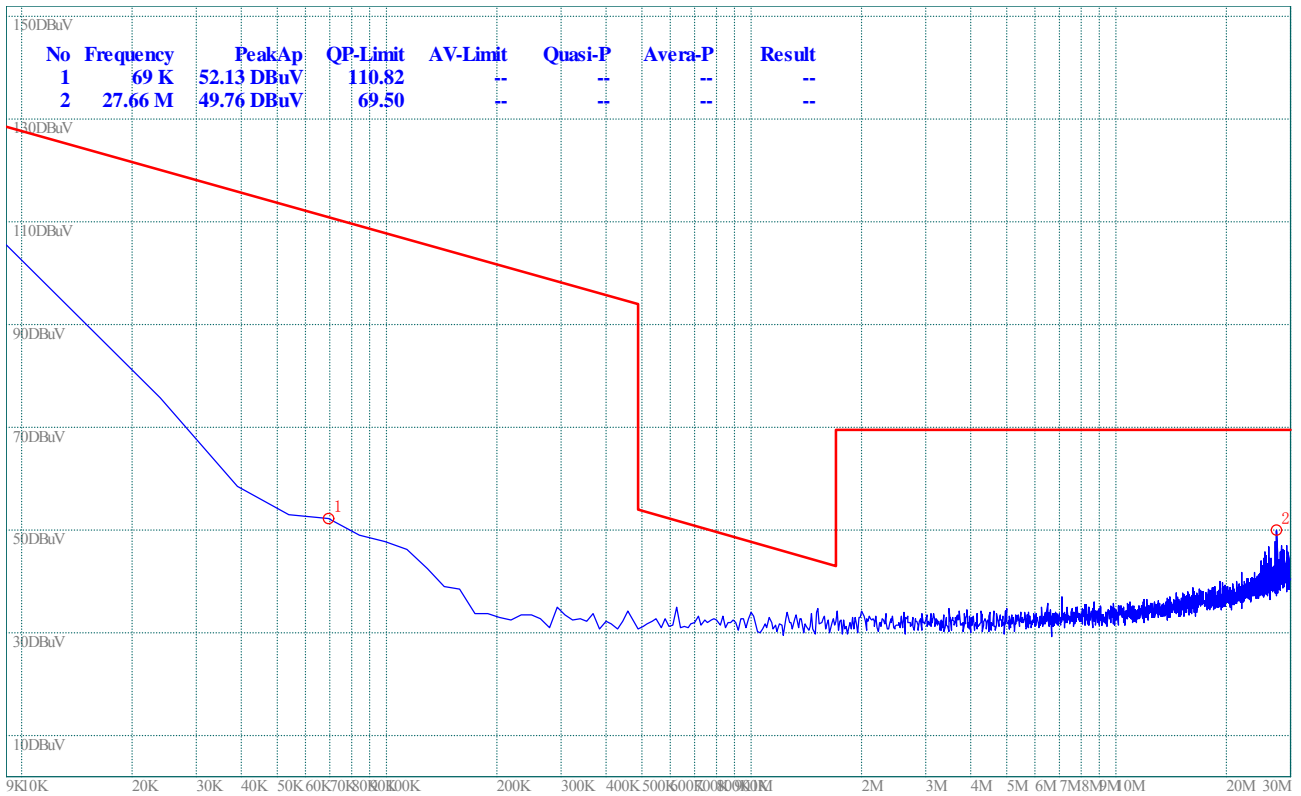
(Plot E.1: 9kHz to 30MHz)
