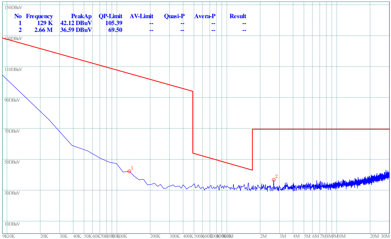
(Plot R.1: 9kHz to 30MHz)
