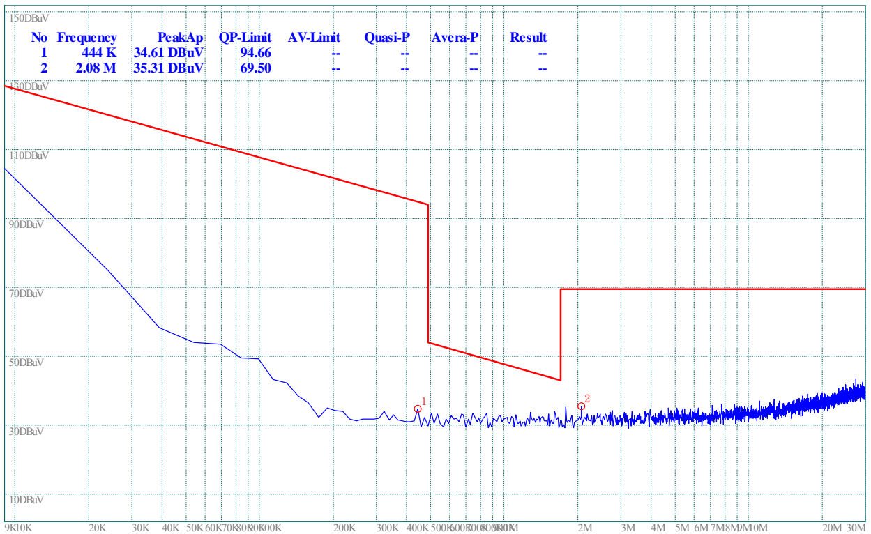
(Plot Q.1: 9kHz to 30MHz)
