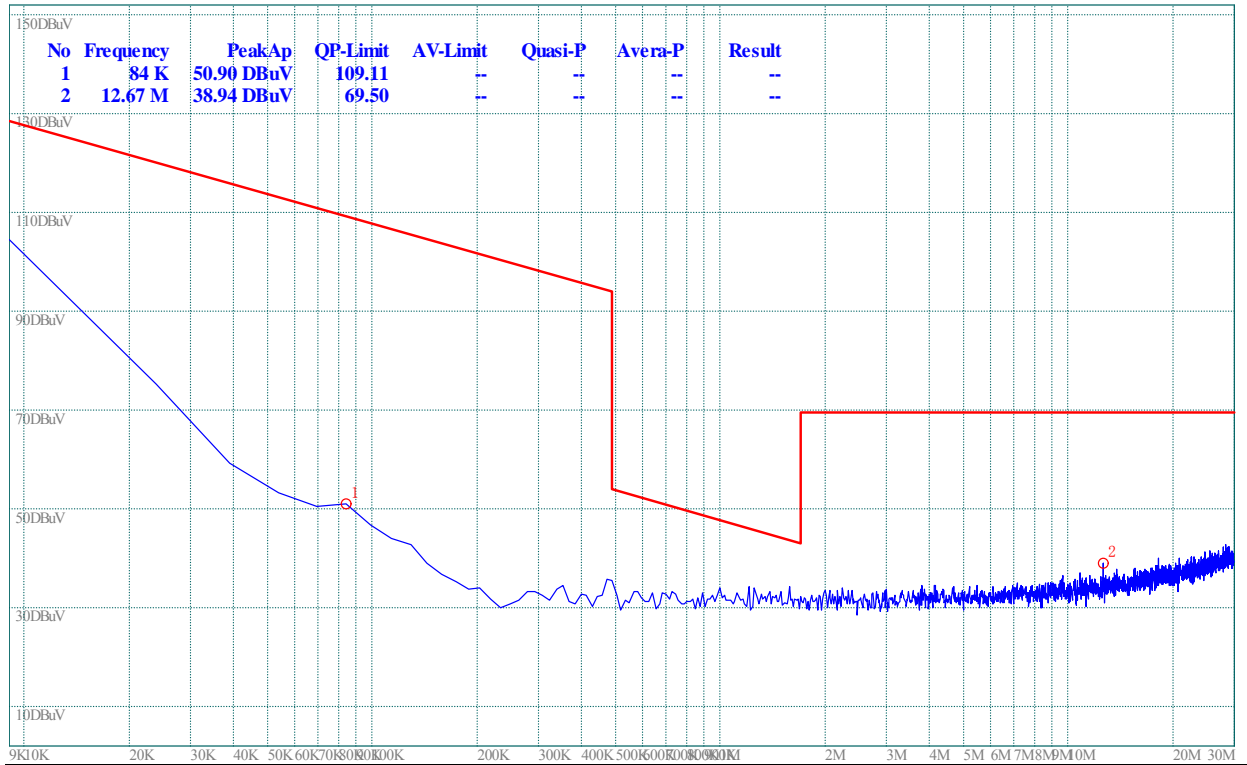
(Plot P.1: 9kHz to 30MHz)
