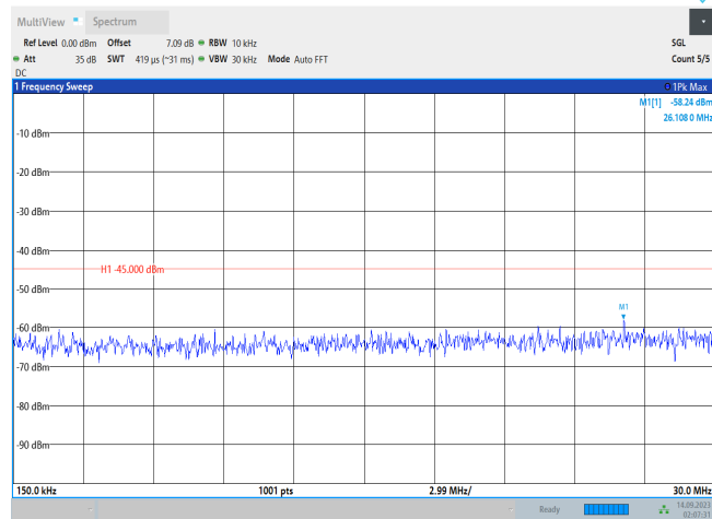
Band38-20MHz-QPSK-37850-1RB#0-Range2:0.15~30MHz
