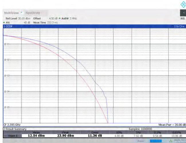
Band41-20MHz-QPSK-40640-100RB#0
