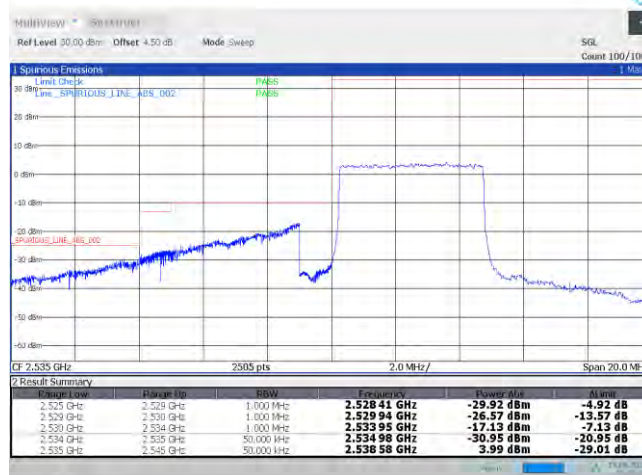
Band41-5MHz-QPSK-40065-25RB#0
