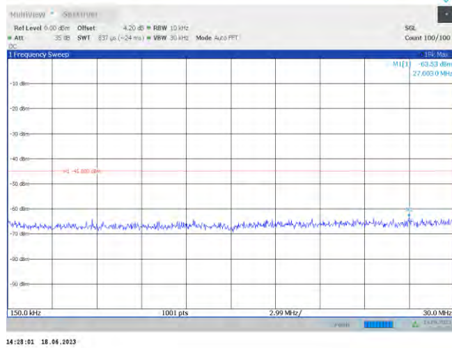
Band41-20MHz-QPSK-40140-1RB#0-Range2:0.15~30MHz
