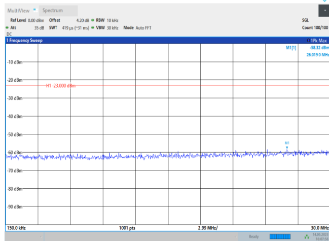
Band13-10MHz-QPSK-23230-1RB#0-Range2:0.15~30MHz
