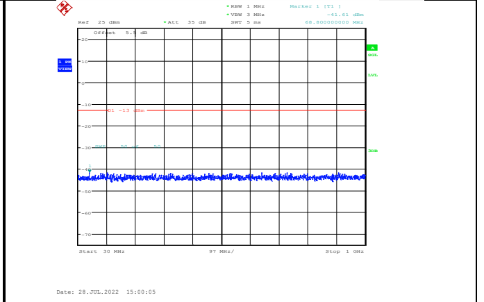
Band66-20MHz-QPSK-132572-1RB#0-Range1:30~1000MHz
