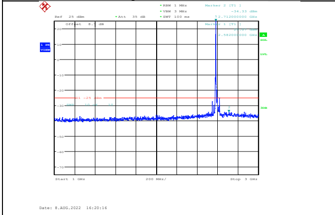
Band41-20MHz-QPSK-40590-1RB#0-Range2:1000~3000MHz
