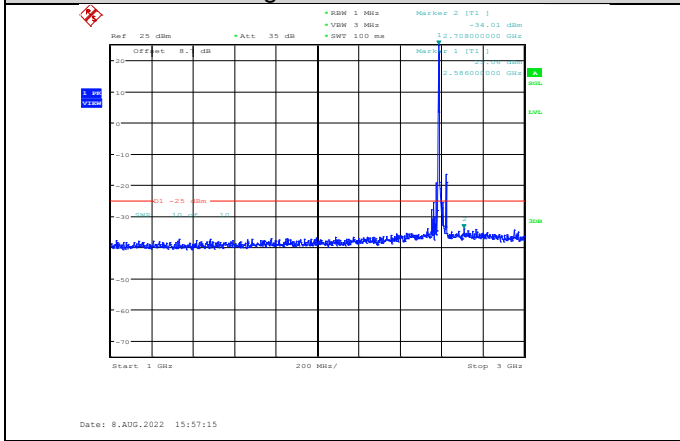
Band38-20MHz-QPSK-38000-1RB#0-Range2:1000~3000MHz
