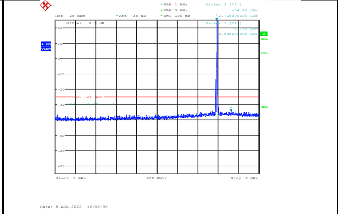
Band41-5MHz-QPSK-40590-1RB#0-Range2:1000~3000MHz
