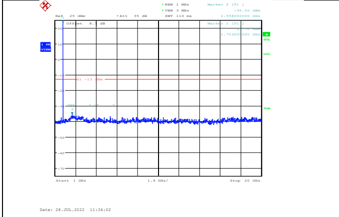
Band66-3MHz-QPSK-131987-1RB#0-Range2:1000~20000MHz
