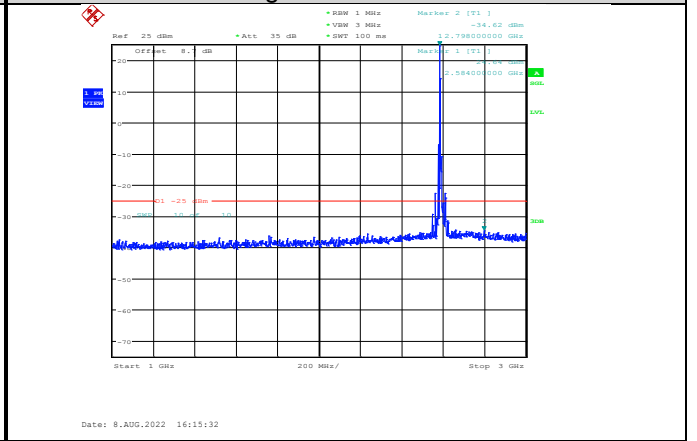
Band41-15MHz-QPSK-40590-1RB#0- Range2:1000~3000MHz
