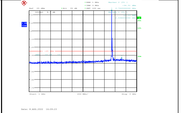
Band41-10MHz-QPSK-40090-1RB#0-Range2:1000~3000MHz
