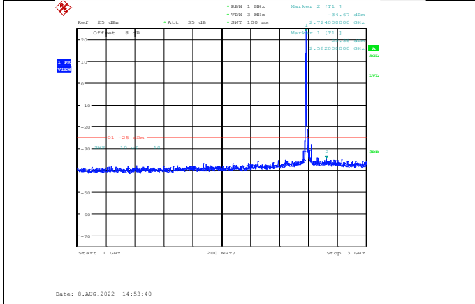
Band41-20MHz-64QAM-40590-1RB#0-Range2:1000~3000MHz
