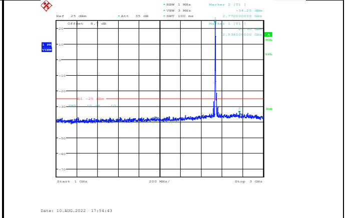
Band41-5MHz-16QAM-40065-1RB#0-Range2:1000~3000MHz
