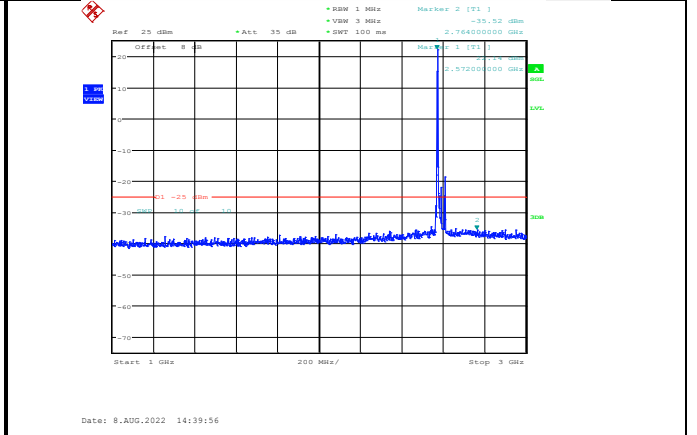
Band38-20MHz-64QAM-37850-1RB#0-Range2:1000~3000MHz
