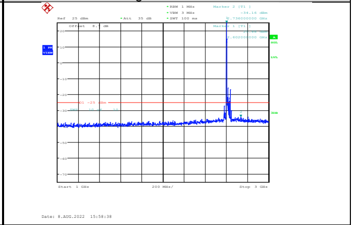
Band38-20MHz-QPSK-38150-1RB#0-Range2:1000~3000MHz
