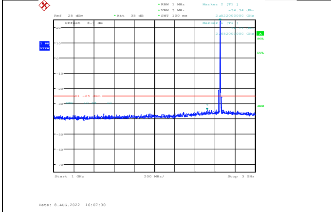
Band41-5MHz-QPSK-41215-1RB#0-Range2:1000~3000MHz
