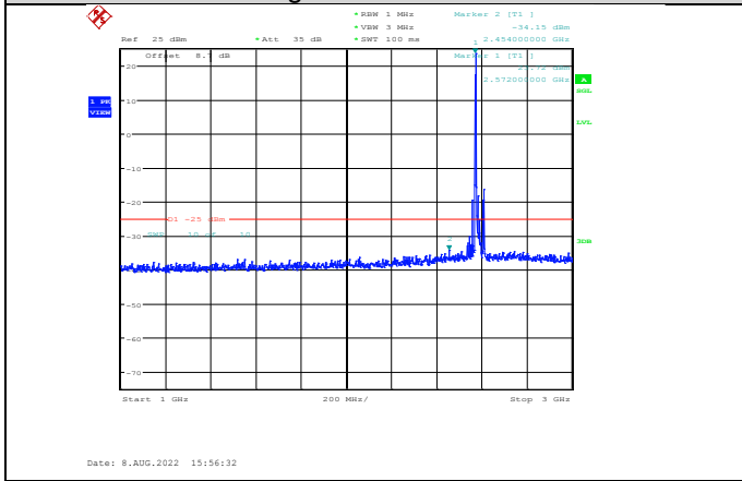
Band38-20MHz-16QAM-37850-1RB#0- Range2:1000~3000MHz
