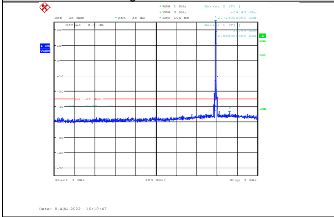
Band41-10MHz-QPSK-40590-1RB#0-Range2:1000~3000MHz
