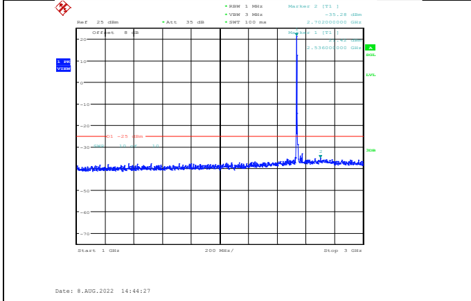
Band41-5MHz-64QAM-40065-1RB#0-Range2:1000~3000MHz
