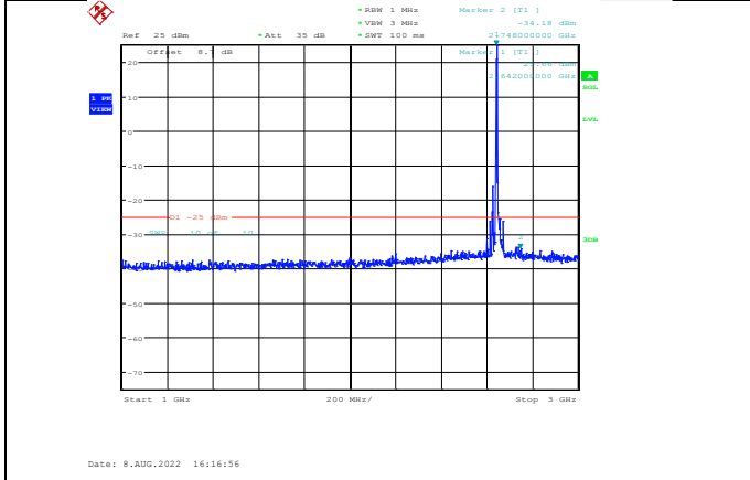
Band41-15MHz-QPSK-41165-1RB#0-Range2:1000~3000MHz
