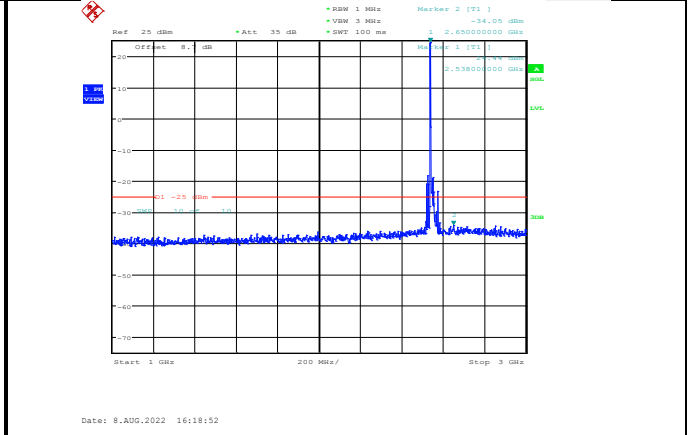
Band41-20MHz-QPSK-40140-1RB#0-Range2:1000~3000MHz
