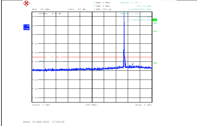
Band41-5MHz-QPSK-40065-1RB#0-Range2:1000~3000MHz
