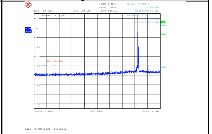
Band41-10MHz-QPSK-41190-1RB#0-Range2:1000~3000MHz
