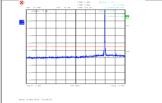
Band41-10MHz-64QAM-40590-1RB#0-Range2:1000~3000MHz
