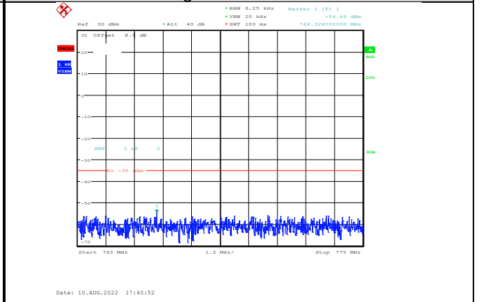
Band13-5MHz-QPSK-23255-1RB#0-Range3:763~775MHz
