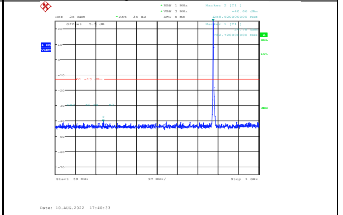
Band13-5MHz-QPSK-23255-1RB#0-Range1:30~1000MHz
