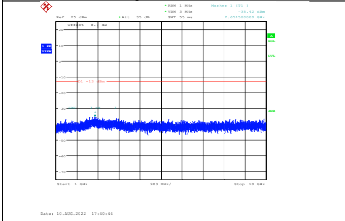
Band13-5MHz-QPSK-23255-1RB#0-Range2:1000~10000MHz
