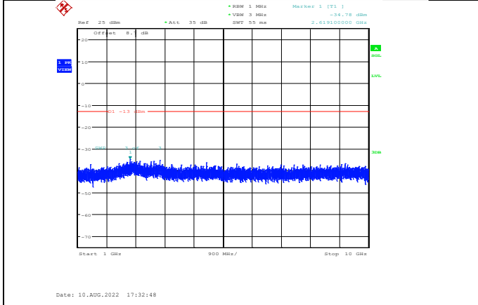
Band12-1.4MHz-QPSK-23017-1RB#0-Range2:1000~10000MHz
