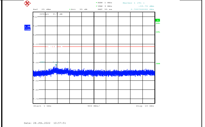
Band12-5MHz-QPSK-23155-1RB#0-Range2:1000~10000MHz
