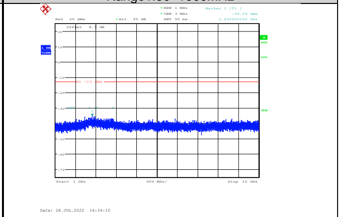
Band12-10MHz-QPSK-23130-1RB#0- Range2:1000~10000MHz
