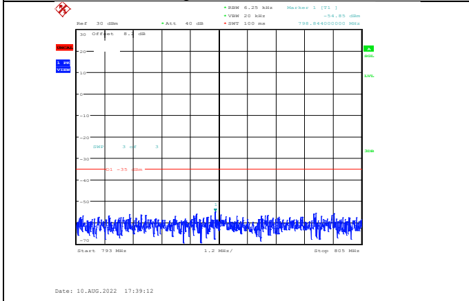
Band13-5MHz-QPSK-23230-1RB#0-Range4:793~805MHz
