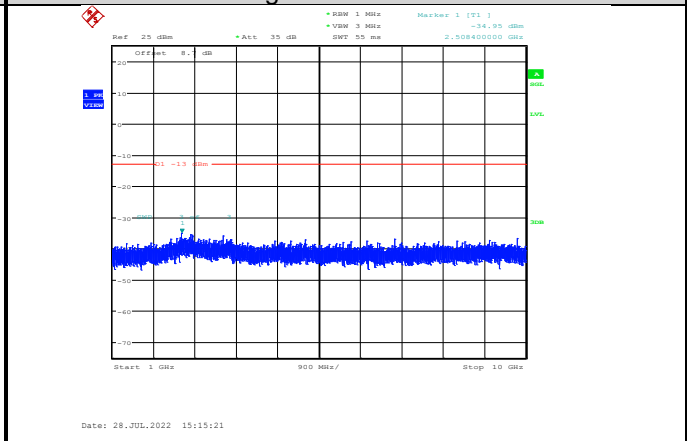
Band26-5MHz-QPSK-26765-1RB#0- Range2:1000~10000MHz
