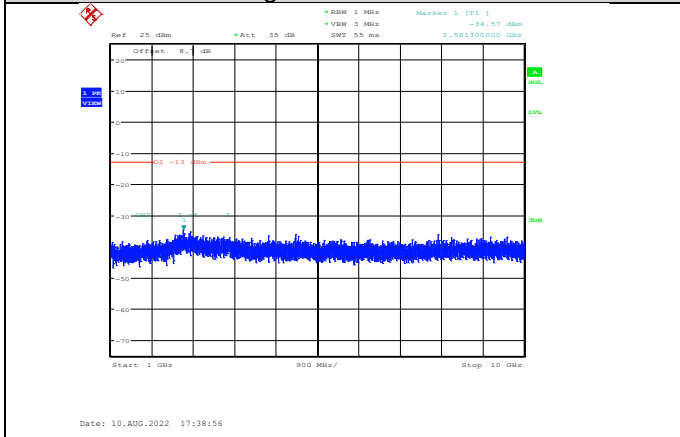
Band13-5MHz-QPSK-23230-1RB#0-Range2:1000~10000MHz
