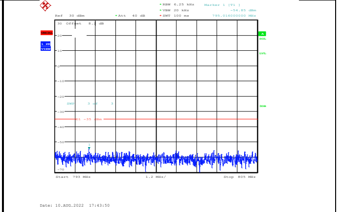
Band13-10MHz-QPSK-23230-1RB#0-Range4:793~805MHz
