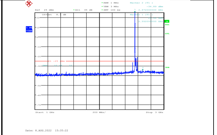
Band7-20MHz-QPSK-21350-1RB#0-Range2:1000~3000MHz
