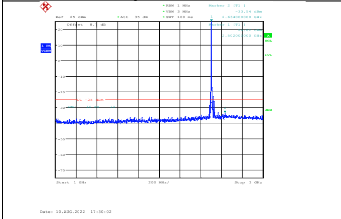
Band7-5MHz-QPSK-20775-1RB#0-Range2:1000~3000MHz
