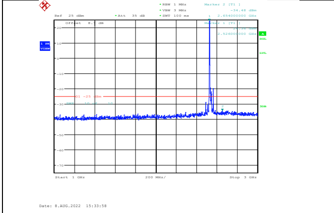
Band7-20MHz-QPSK-21100-1RB#0-Range2:1000~3000MHz
