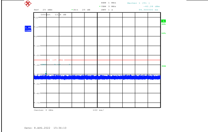
Band7-20MHz-QPSK-21100-1RB#0-Range3:3000~27000MHz
