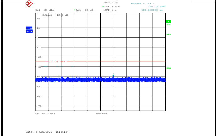
Band7-20MHz-QPSK-21350-1RB#0-Range3:3000~27000MHz
