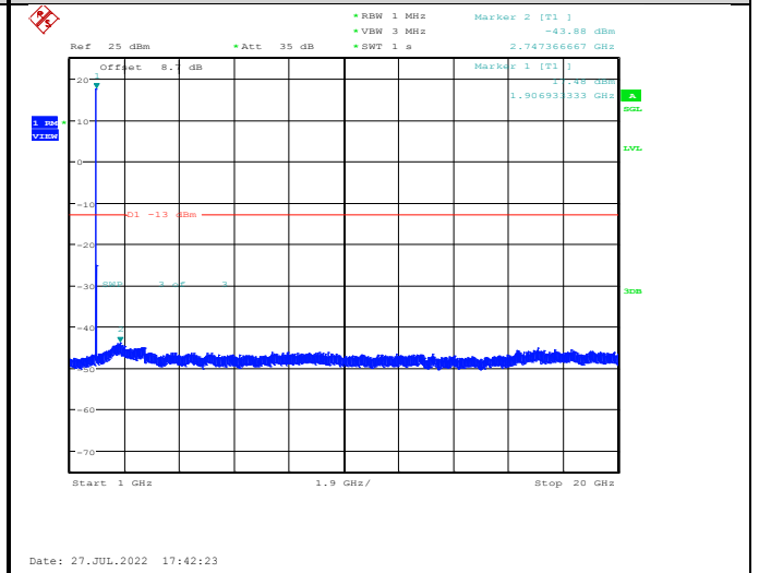
Band II-9538-1000~20000MHz
