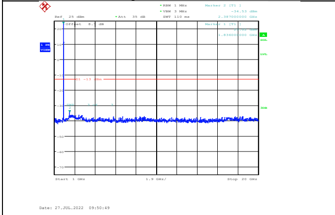
Band2-20MHz-16QAM-18700-1RB#0-Range2:1000~20000MHz
