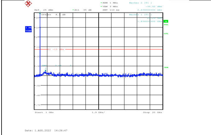
Band2-20MHz-64QAM-18700-1RB#0-Range2:1000~20000MHz
