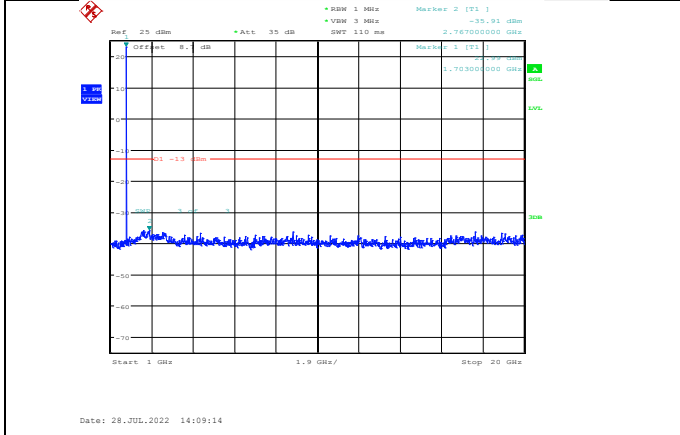
Band4-1.4MHz-QPSK-19957-1RB#0- Range2:1000~20000MHz
