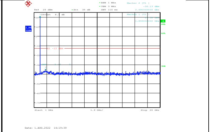
Band2-3MHz-64QAM-19185-1RB#0-Range2:1000~20000MHz
