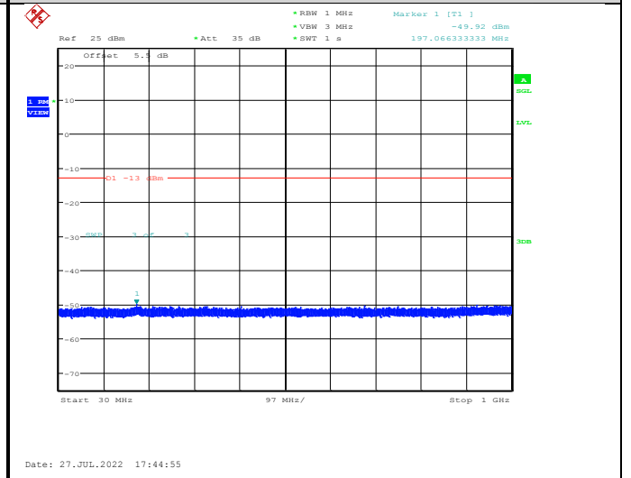
Band IV-1513-30~1000MHz
