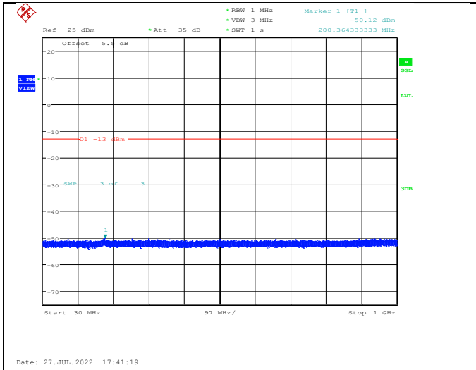
Band II-9262-30~1000MHz
