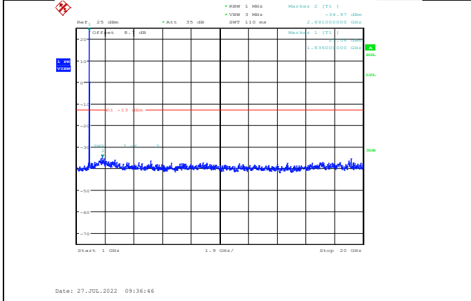
Band2-3MHz-16QAM-18615-1RB#0-Range2:1000~20000MHz
