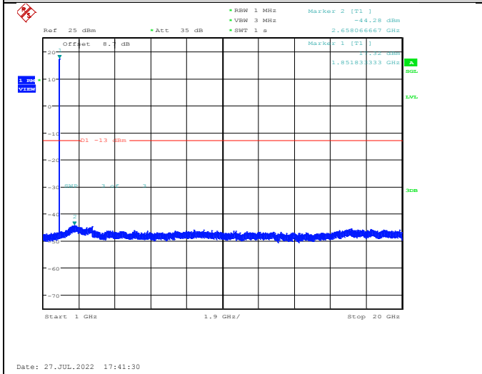
Band II-9262-1000~20000MHz
