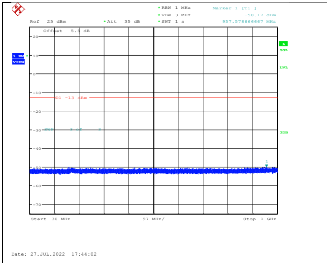
Band IV-1312-30~1000MHz
