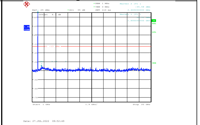
Band2-20MHz-16QAM-19100-1RB#0-Range2:1000~20000MHz
