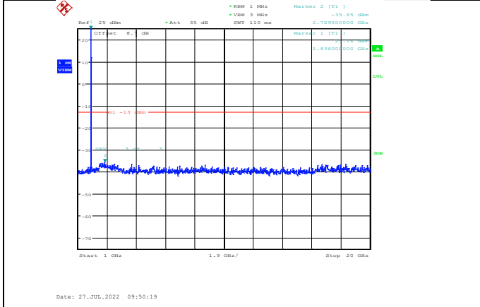
Band2-20MHz-QPSK-18700-1RB#0- Range2:1000~20000MHz
