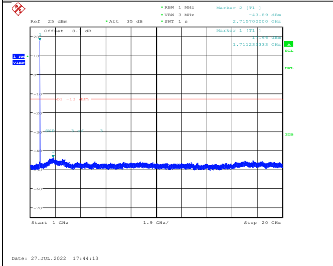
Band IV-1312-1000~20000MHz
