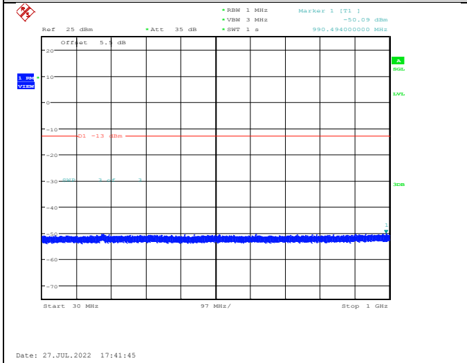
Band II-9400-30~1000MHz
