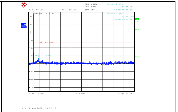
Band2-20MHz-64QAM-18900-1RB#0-Range2:1000~20000MHz
