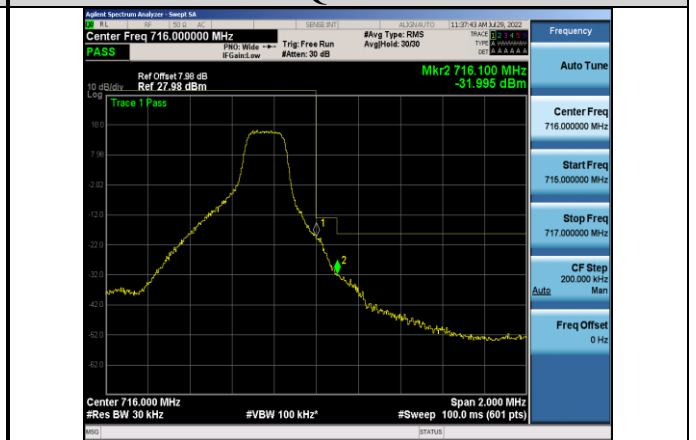
Band12-3MHz-QPSK-23165-1RB#14
