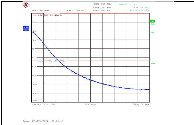
Band2-20MHz-16QAM-19100-1RB#99
