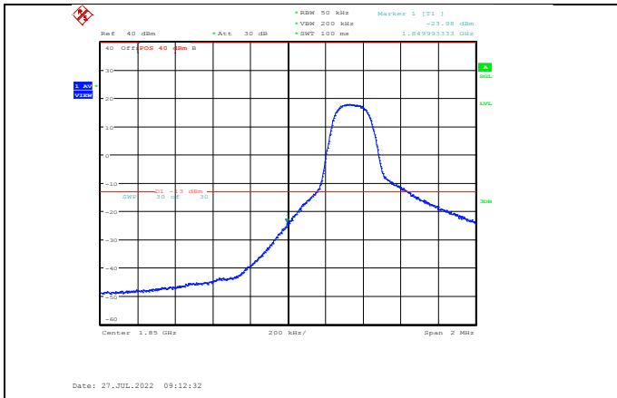
Band2-5MHz-QPSK-18625-1RB#0
