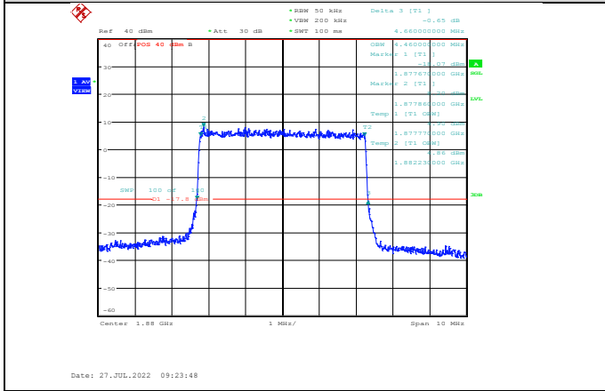
Band2-5MHz-QPSK-18900-25RB#0
