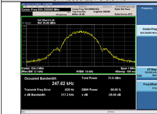
EGPRS850-128-8-0.3172
