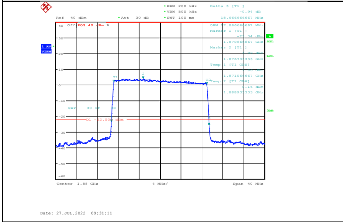
Band2-20MHz-16QAM-18900-100RB#0
