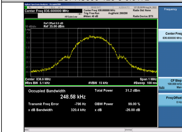
EGPRS850-190-8-0.3204
