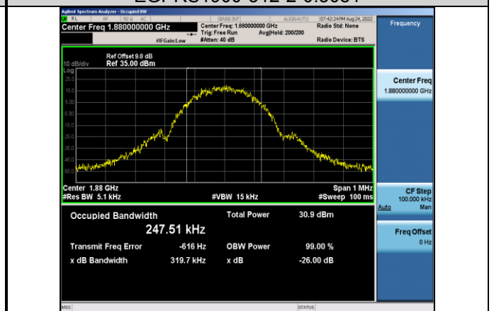
EGPRS1900-512-2-0.3081
