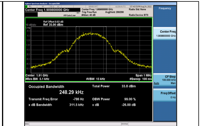
GPRS1900-810-0-0.3115
