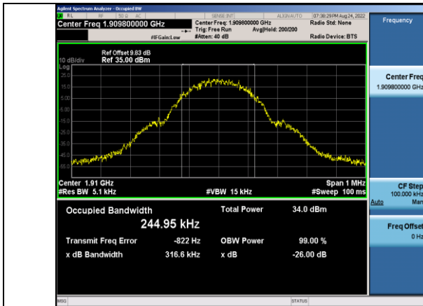
GSM1900-810-0-0.3166
