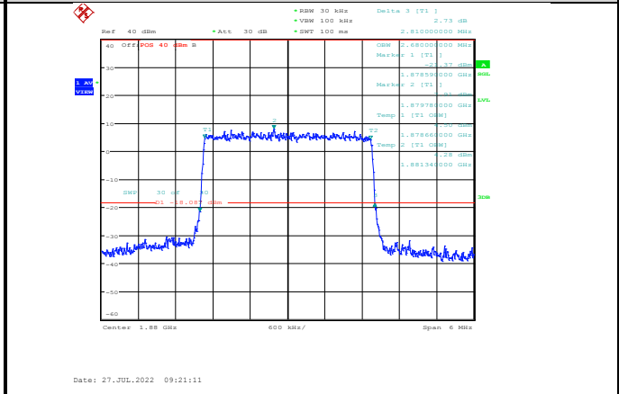
Band2-3MHz-QPSK-18915-15RB#0
