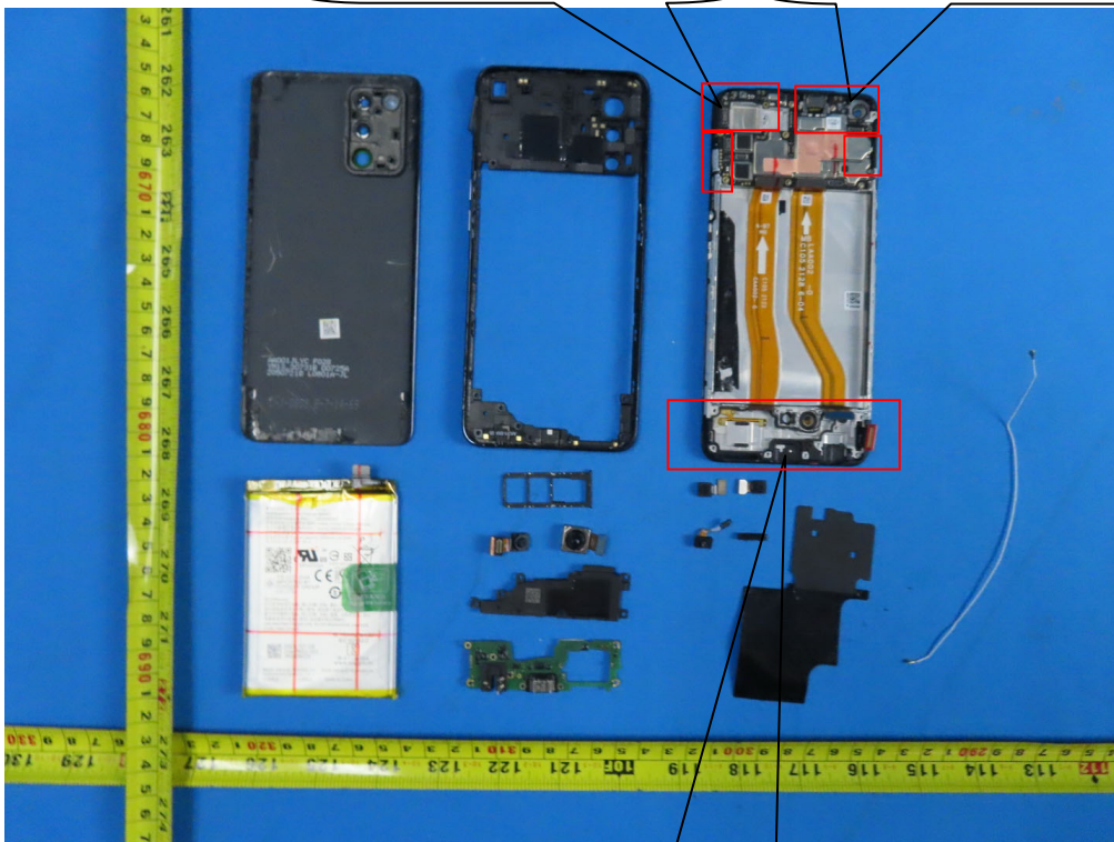
BT/WIFI/GPS Antenna 2/3/4G Second Antenna
