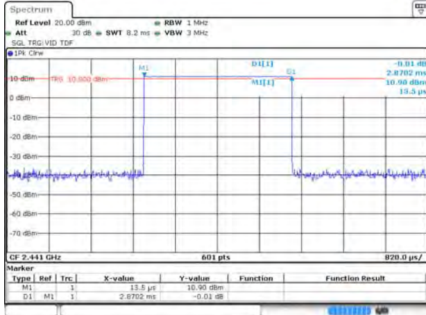
GFSK DH5
