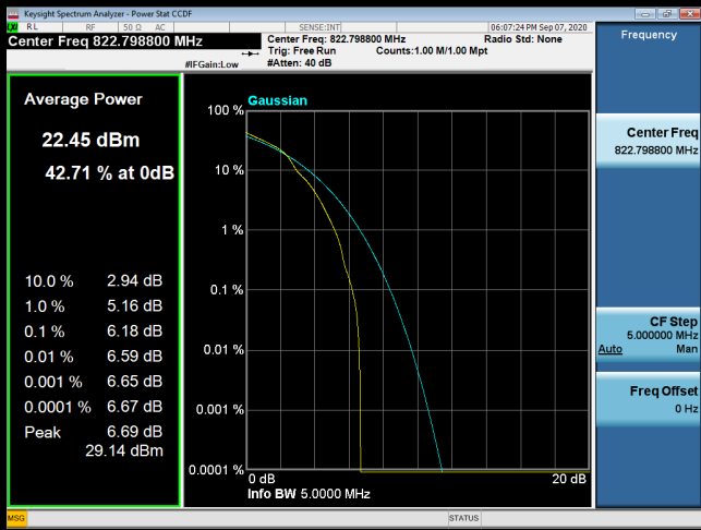
64QAM-26783
