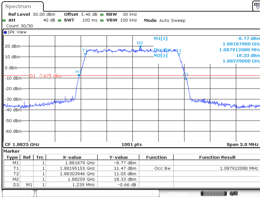
Band25-1.4MHz-QPSK-26365-6RB#0-1.088
