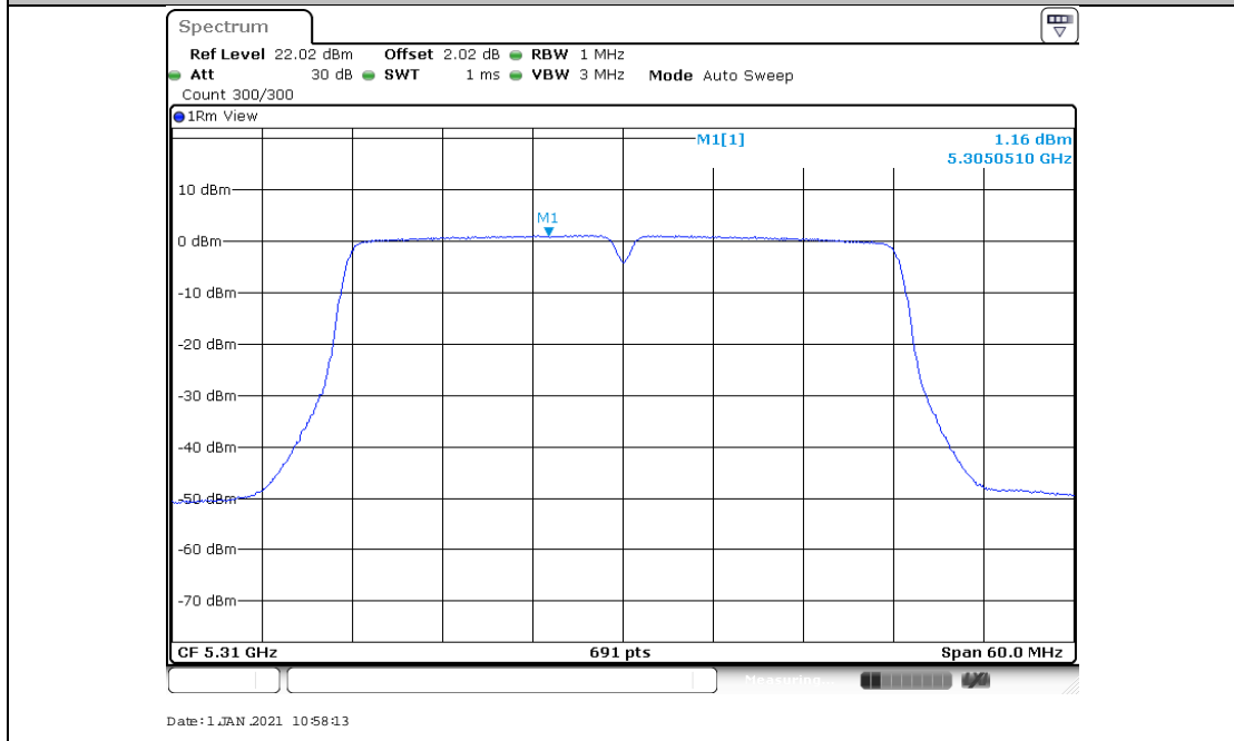
11AC40MIMO_Ant2_5310
