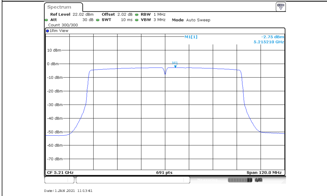
11AC80MIMO_Ant2_5210
