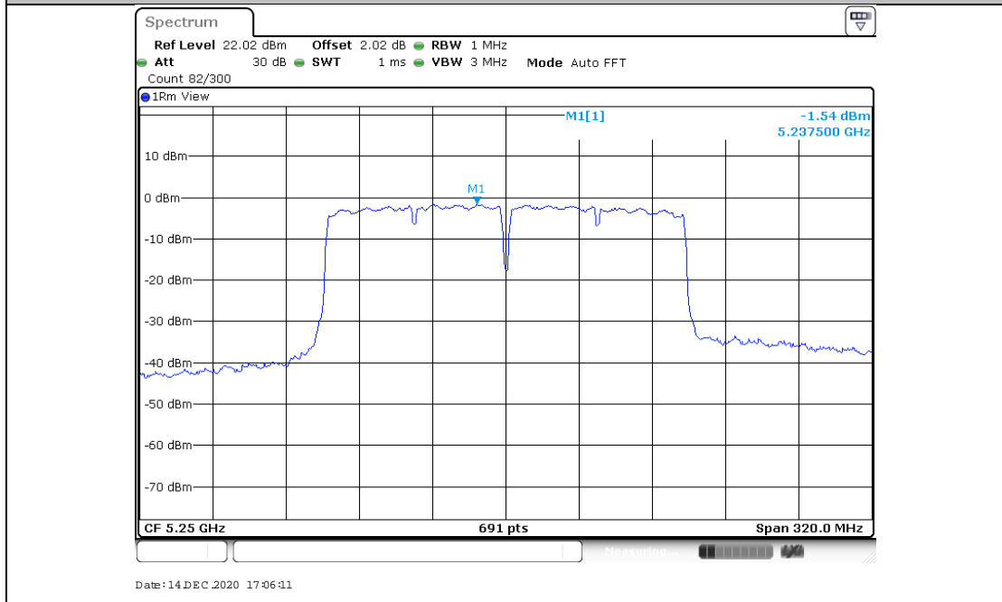
11AC160MIMO_Ant2_5250
