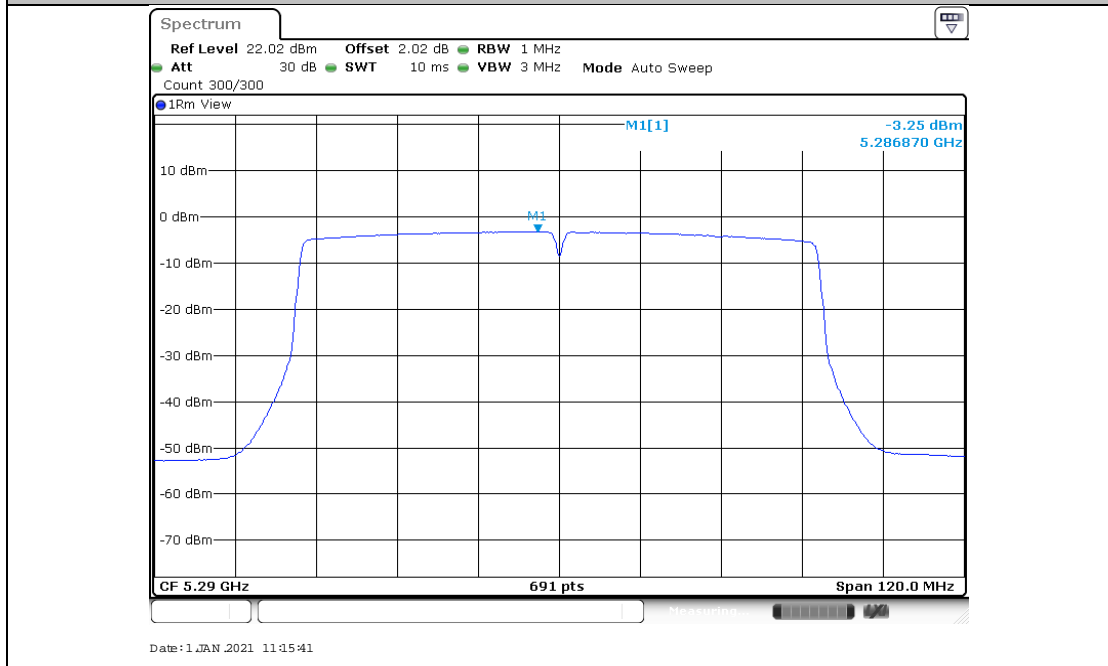
11AC80MIMO_Ant2_5290
