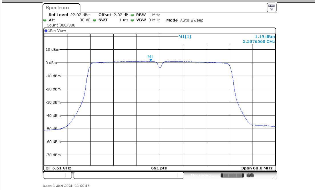
11AC40MIMO_Ant2_5510
