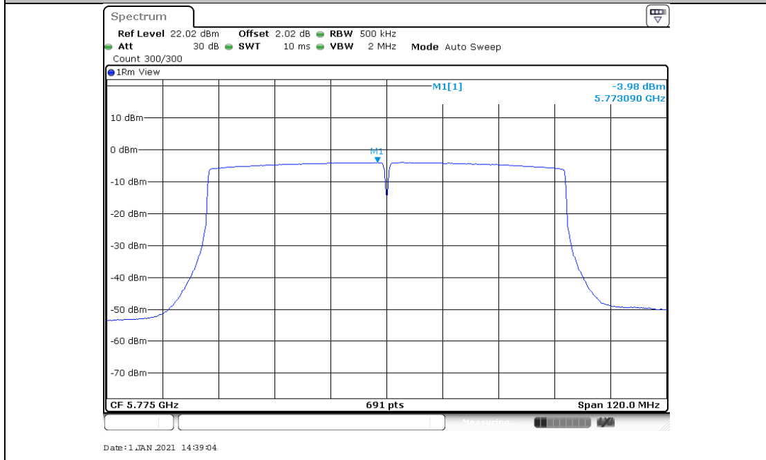
11AC80MIMO_Ant2_5775
