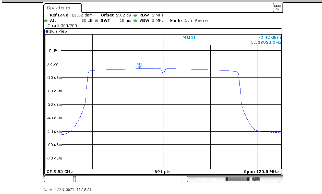
11AC80MIMO_Ant2_5530
