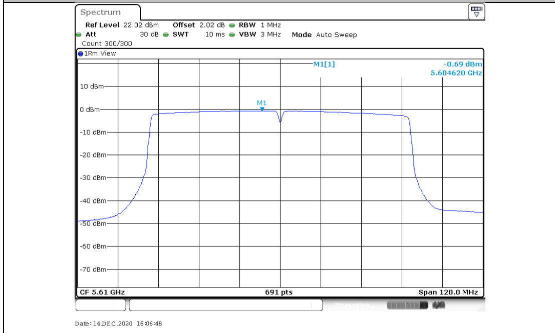
11AC80MIMO_Ant2_5610
