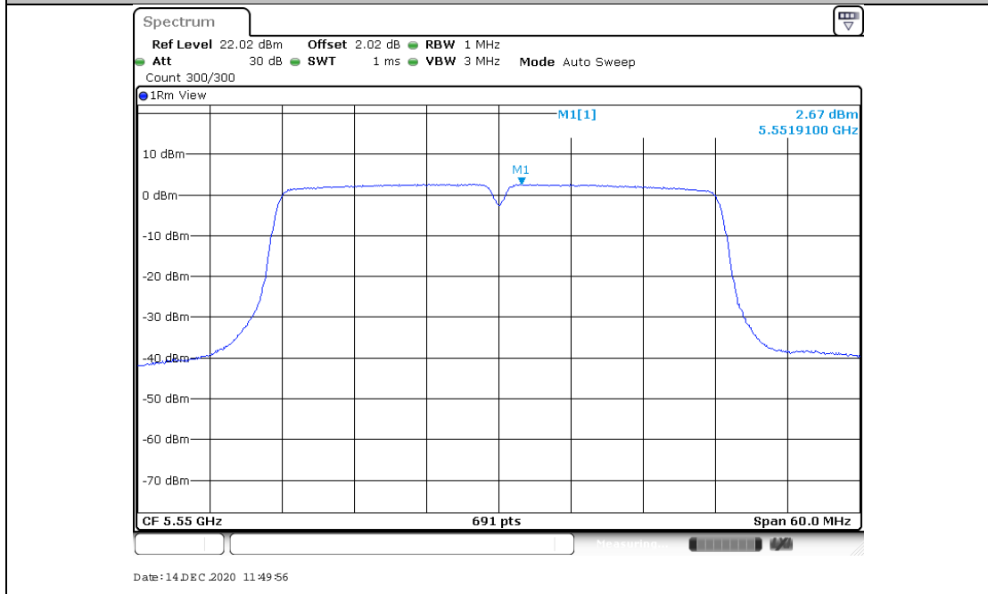
11AC40MIMO_Ant2_5550
