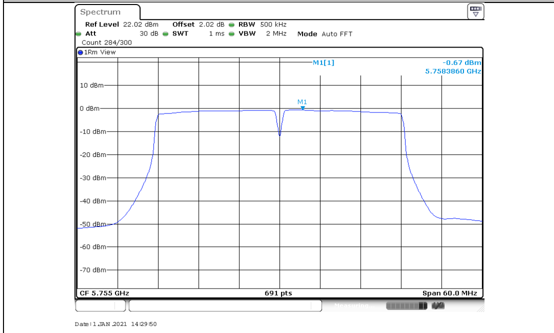
11AC40MIMO_Ant2_5755
