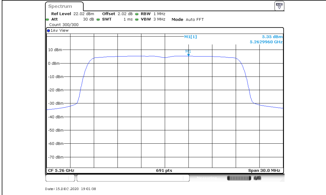
11AX20SISO_Ant2_5260
