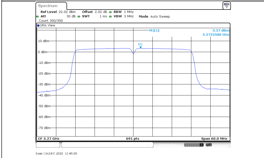
11AC40MIMO_Ant2_5270
