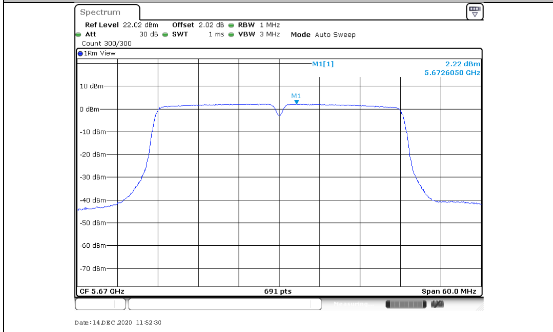
11AC40MIMO_Ant2_5670
