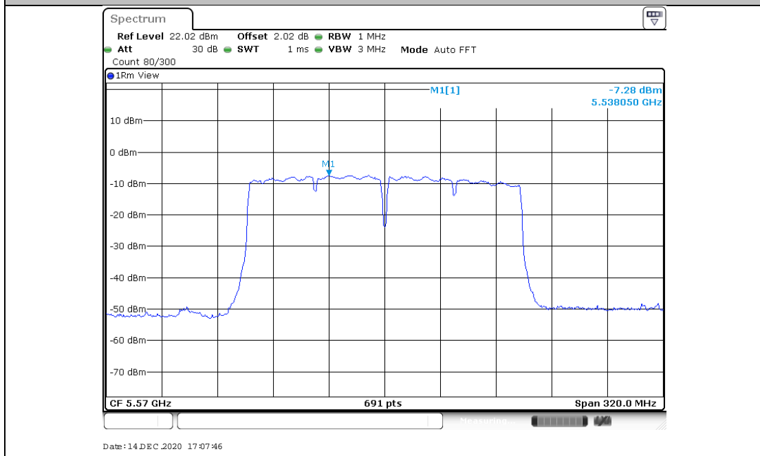
11AC160MIMO_Ant2_5570
