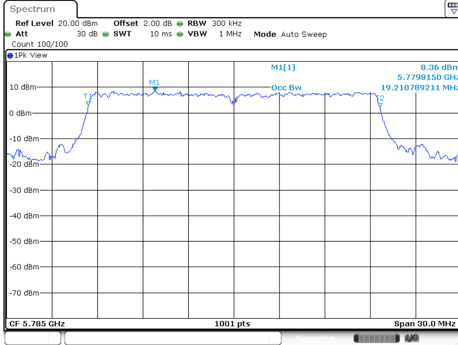
11AX20-242TSISO_Ant2_5785
