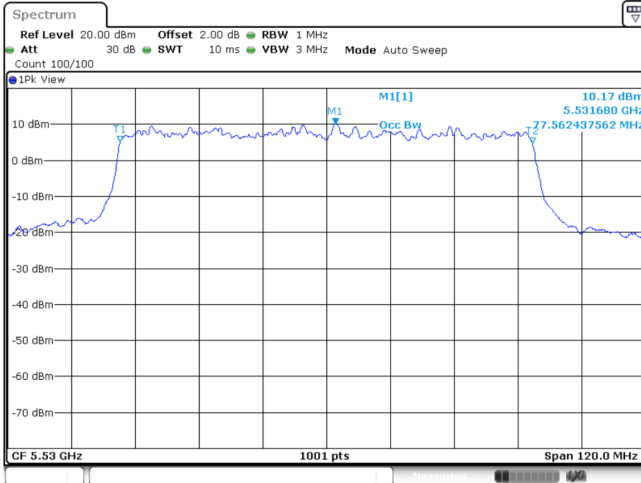
11AX80-996TMIMO_Ant1_5530
