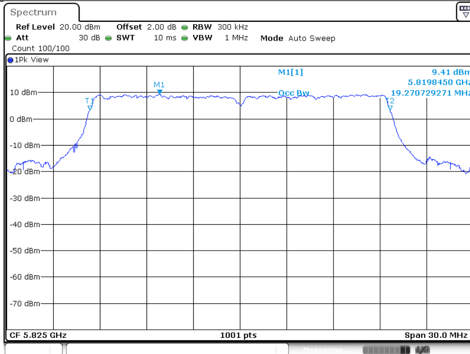
11AX20-242TSISO_Ant1_5825
