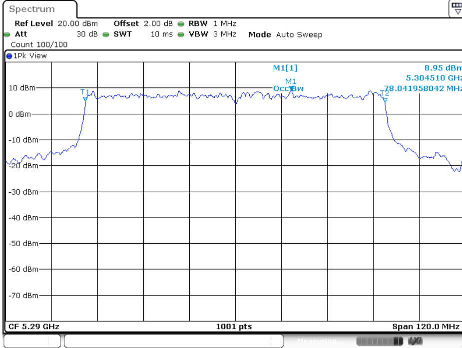
11AX80-996TMIMO_Ant2_5290
