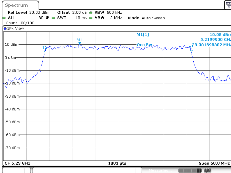
11AX40-484TMIMO_Ant1_5230
