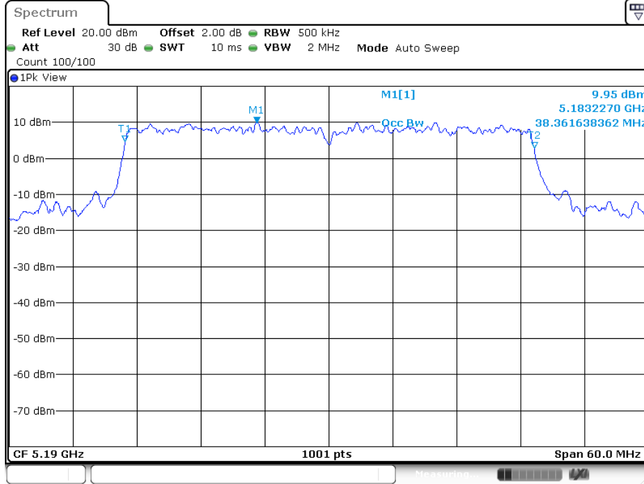
11AX40-484TMIMO_Ant2_5190
