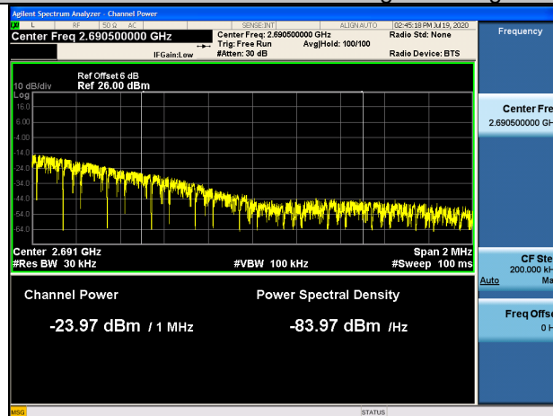
N41 TM5 100MHz 528000 Edge 1RB Right
