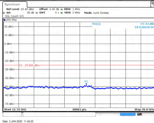
LTE Band CA_41C_100RB+100RB_64QAM_40719+40521_1RB#0+0RB#0_30_1000
