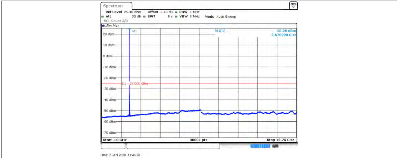
LTE Band CA_41C_100RB+100RB_QPSK_41490+41292_1RB#0+0RB#0_12750_26000
