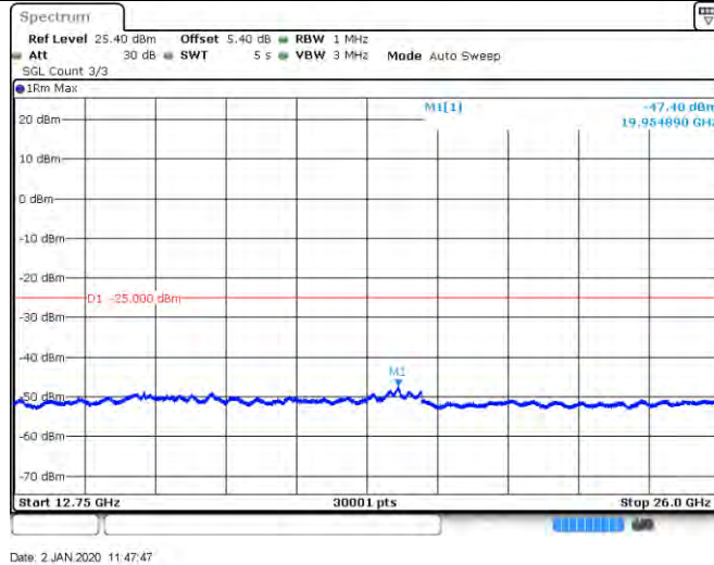
LTE Band CA_41C_100RB+100RB_QPSK_40719+40521_1RB#0+0RB#0_30_100
