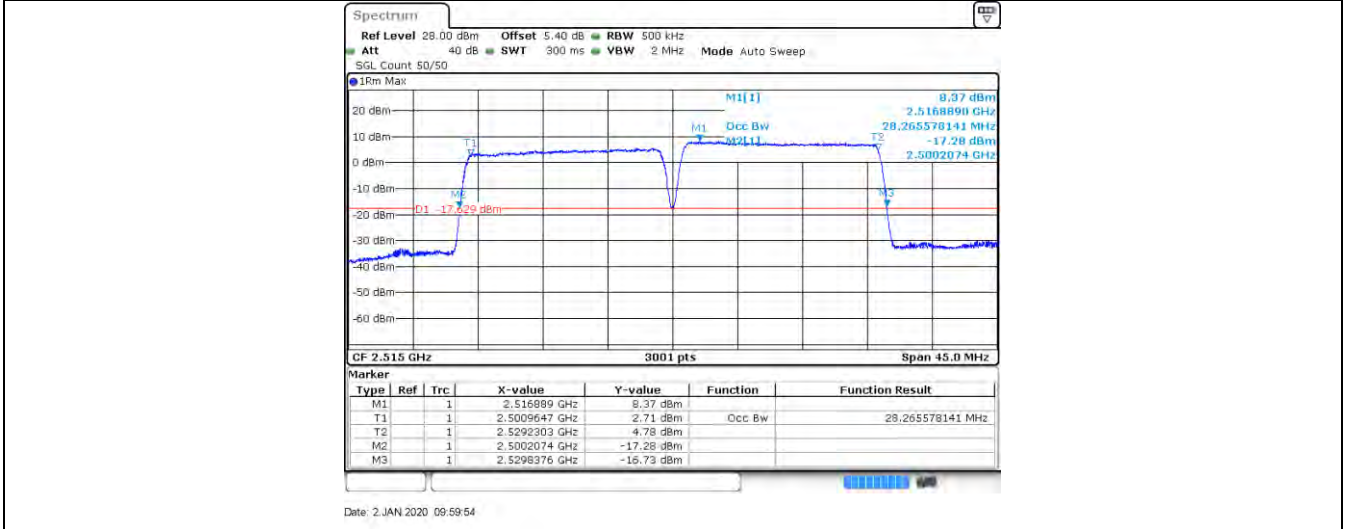
LTE Band CA_7C_75RB+75RB_QPSK_21175+21025_75RB#0+75RB#0
