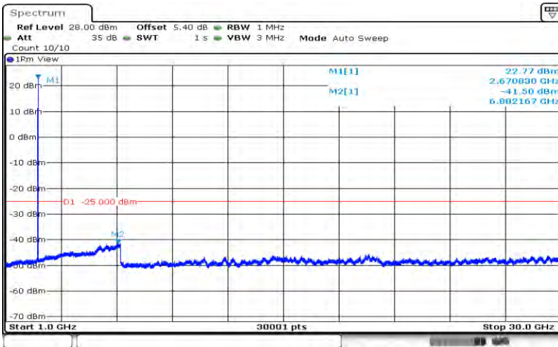
Band41-20MHz-QPSK-41490-1RB#0-Range2:1000~30000MHz
