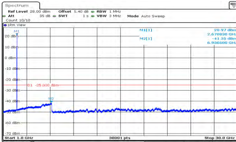
Band41-20MHz-64QAM-41490-1RB#0-Range2:1000~30000MHz
