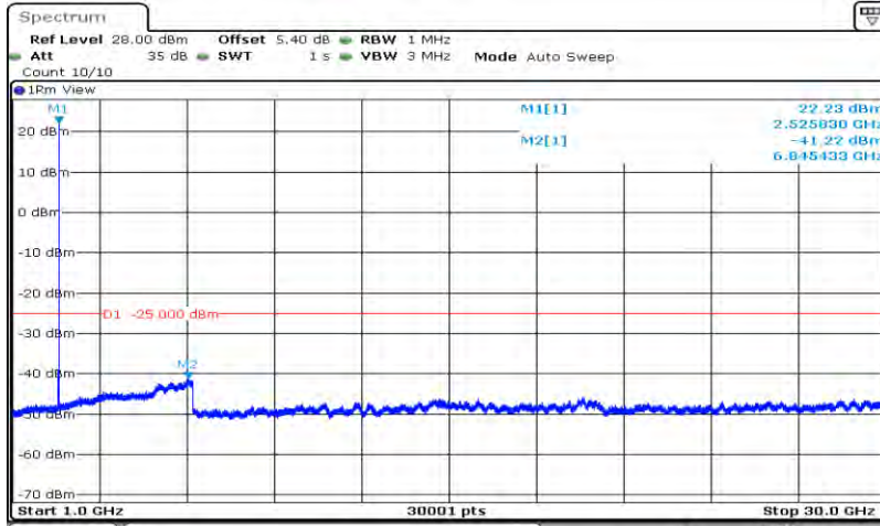
Band7-20MHz-QPSK-21100-1RB#0-Range2:1000~30000MHz
