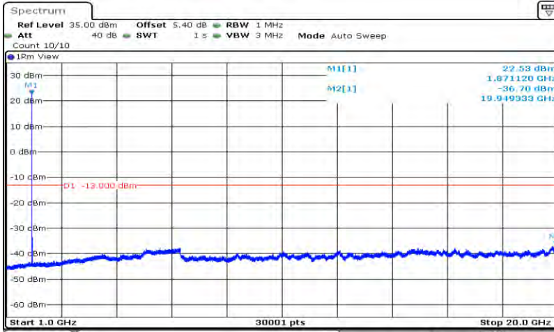
Band2-20MHz-QPSK-18900-1RB#0-Range2:1000~20000MHz
