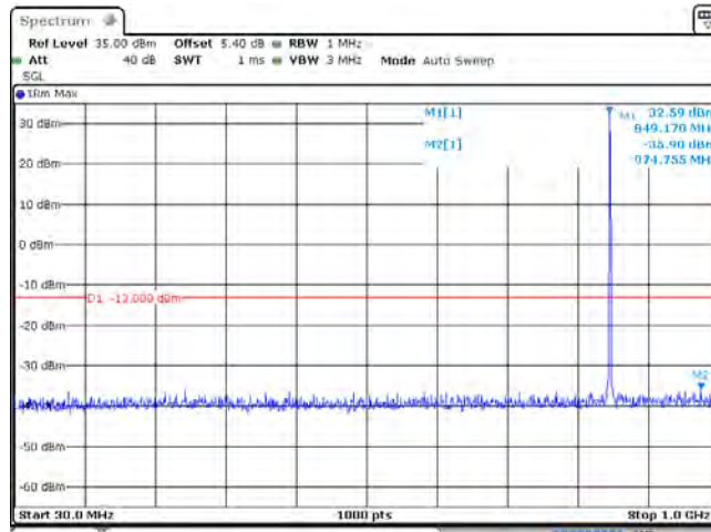
GSM850_251
