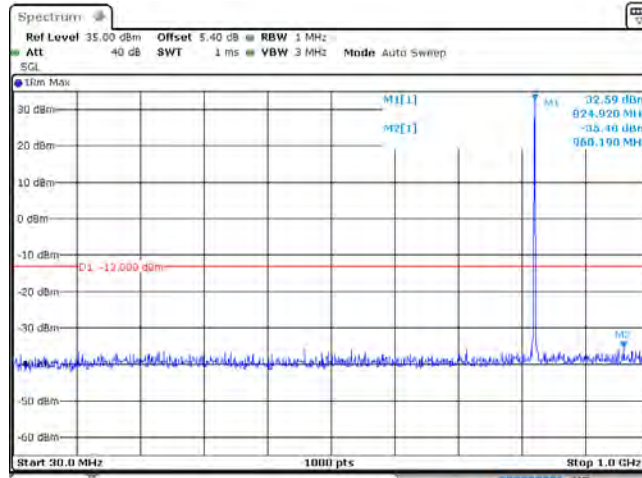
GSM850_128
