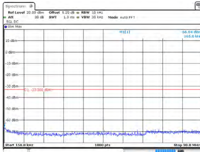
GSM850_251
