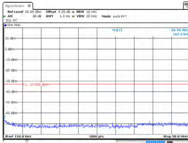
GSM1900_810
