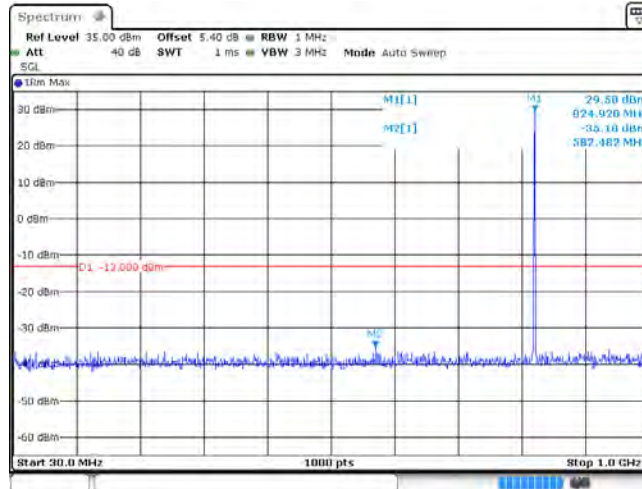
EGPRS850_128
