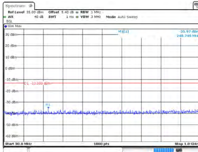
GSM1900_810
