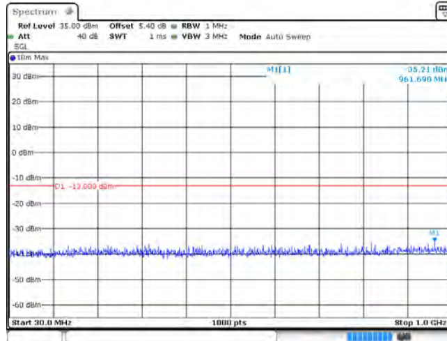
GSM1900_661
