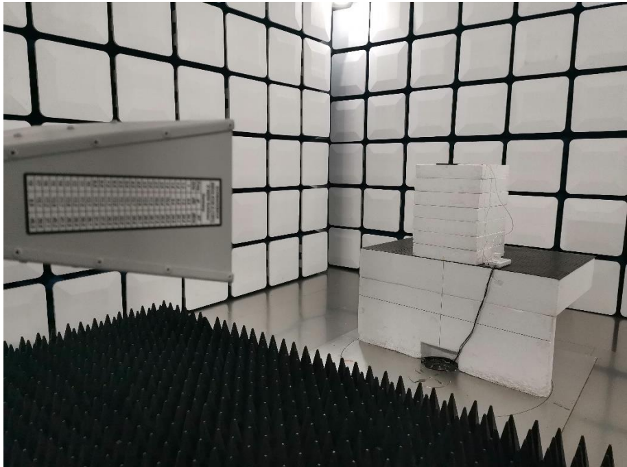
Above 1GHz-BT/WIFI
