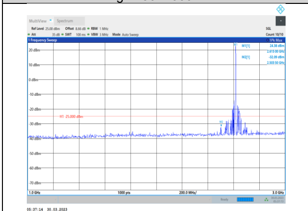
Band38-5MHz-QPSK-38225-1RB#0-Range2:1000~3000MHz
