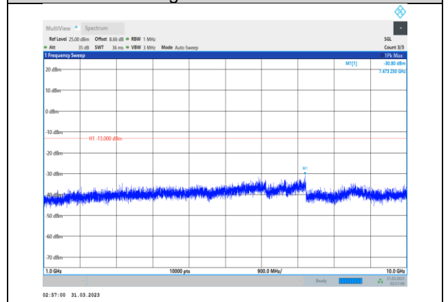
Band26-5MHz-QPSK-26765-1RB#0-Range2:1000~10000MHz
