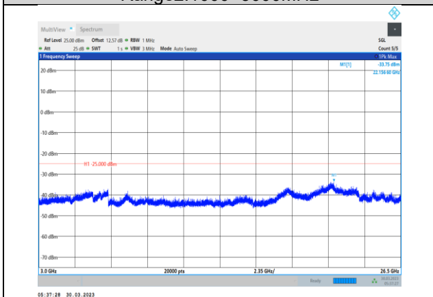
Band38-5MHz-QPSK-38225-1RB#0-Range3:3000~26500MHz
