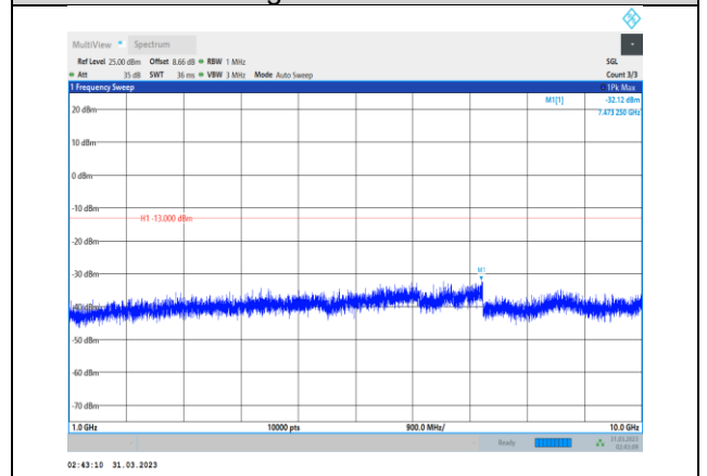
Band12-5MHz-QPSK-23155-1RB#0- Range2:1000~10000MHz
