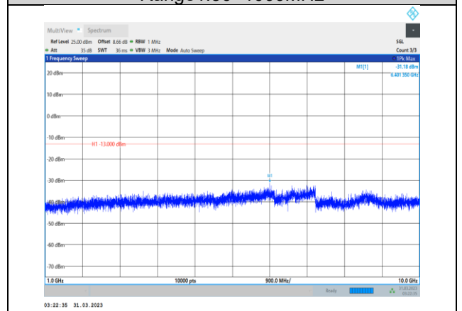
Band12-10MHz-QPSK-23130-1RB#0- Range2:1000~10000MHz
