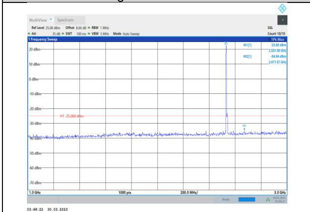
Band7-10MHz-QPSK-21100-1RB#0- Range2:1000~3000MHz
