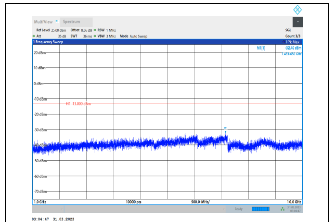
Band5-10MHz-QPSK-20525-1RB#0- Range2:1000~10000MHz
