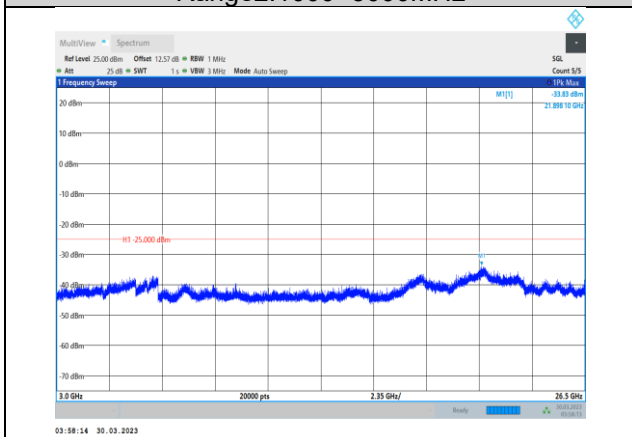
Band7-15MHz-QPSK-20825-1RB#0- Range3:3000~26500MHz
