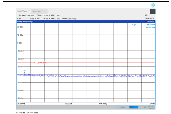
Band7-20MHz-QPSK-21350-1RB#0- Range1:30~1000MHz
