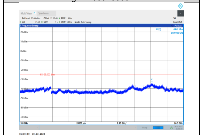
Band7-20MHz-QPSK-20850-1RB#0- Range3:3000~26500MHz
