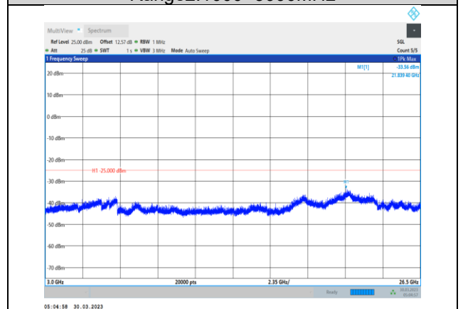
Band7-20MHz-QPSK-21350-1RB#0- Range3:3000~26500MHz
