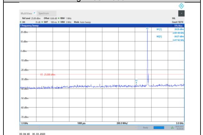
Band7-20MHz-QPSK-21350-1RB#0- Range2:1000~3000MHz
