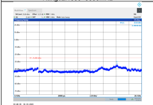
Band7-10MHz-QPSK-21100-1RB#0- Range3:3000~26500MHz
