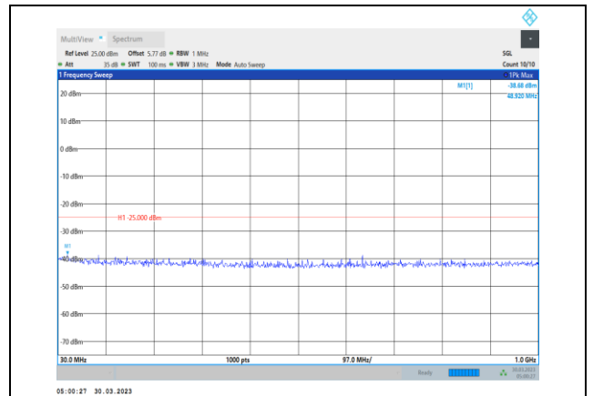
Band7-20MHz-QPSK-20850-1RB#0- Range1:30~1000MHz
