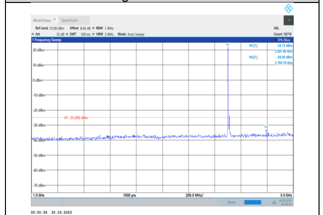
Band7-20MHz-QPSK-20850-1RB#0- Range2:1000~3000MHz
