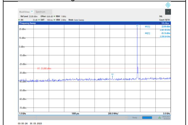
Band7-10MHz-QPSK-21400-1RB#0- Range2:1000~3000MHz
