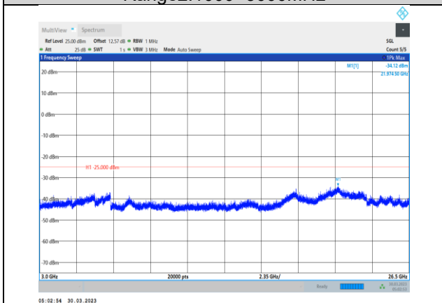
Band7-20MHz-QPSK-21100-1RB#0- Range3:3000~26500MHz
