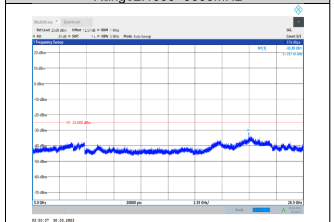
Band7-10MHz-QPSK-21400-1RB#0- Range3:3000~26500MHz
