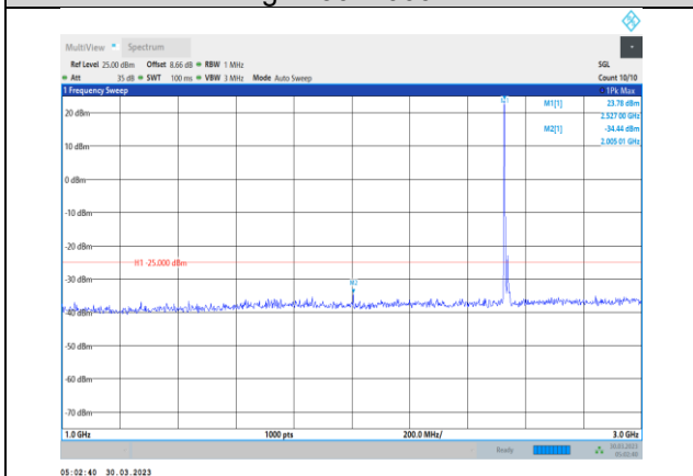
Band7-20MHz-QPSK-21100-1RB#0- Range2:1000~3000MHz
