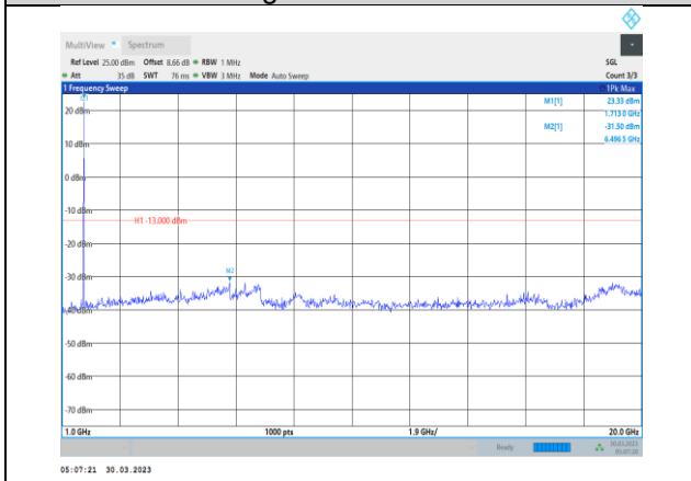
Band4-1.4MHz-QPSK-19957-1RB#0- Range2:1000~20000MHz
