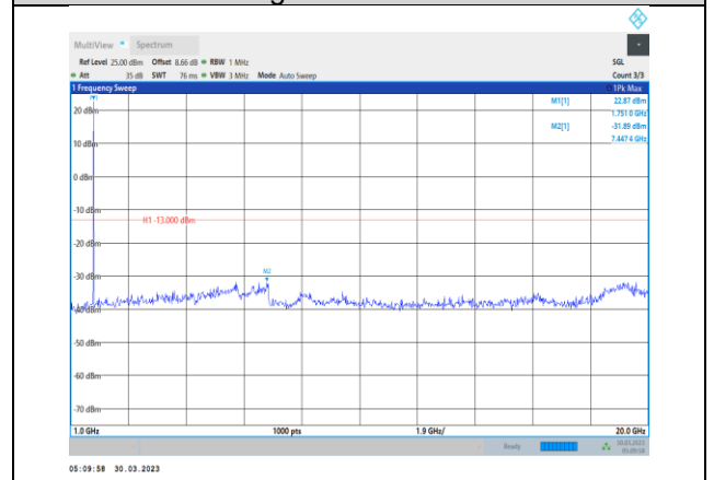
Band4-1.4MHz-QPSK-20393-1RB#0- Range2:1000~20000MHz
