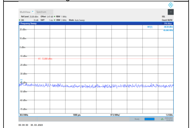
Band4-1.4MHz-QPSK-20393-1RB#0- Range1:30~1000MHz
