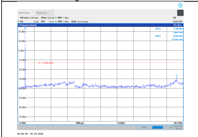
Band2-20MHz-16QAM-18700-1RB#0- Range2:1000~20000MHz
