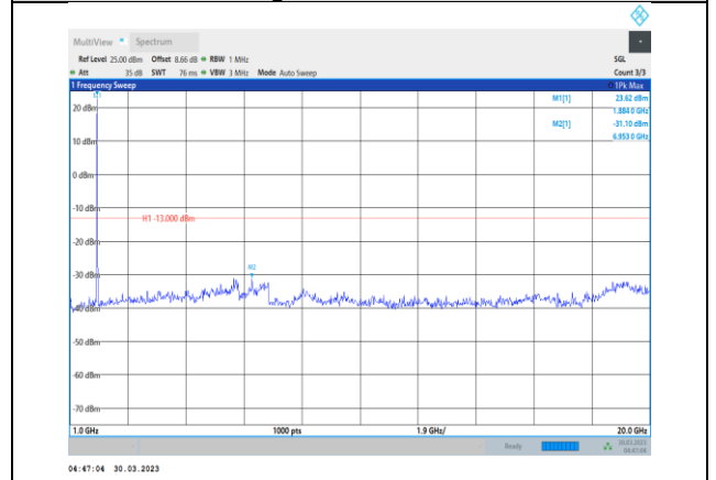
Band2-20MHz-QPSK-19100-1RB#0-Range2:1000~20000MHz
