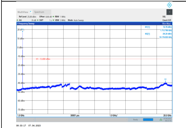
Band4-1312-1000~20000MHz
