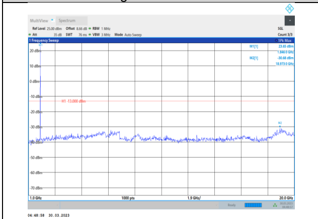
Band2-5MHz-QPSK-18625-1RB#0- Range2:1000~20000MHz
