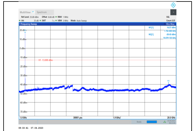
Band4-1413-1000~20000MHz
