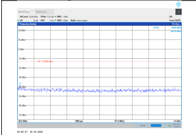
Band2-20MHz-QPSK-18900-1RB#0-Range1:30~1000MHz
