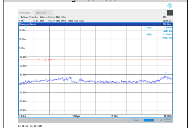
Band2-5MHz-QPSK-19175-1RB#0- Range2:1000~20000MHz
