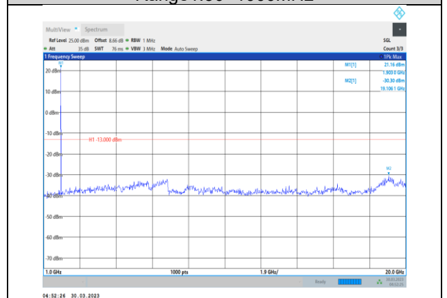
Band2-5MHz-64QAM-19175-1RB#0- Range2:1000~20000MHz
