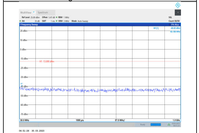
Band2-5MHz-QPSK-19175-1RB#0- Range1:30~1000MHz
