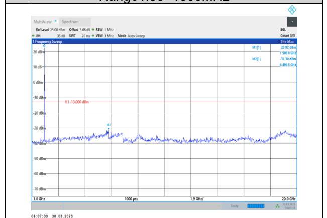
Band2-15MHz-QPSK-19125-1RB#0- Range2:1000~20000MHz
