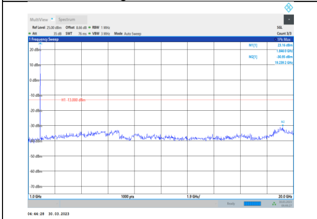
Band2-20MHz-QPSK-18700-1RB#0-Range2:1000~20000MHz
