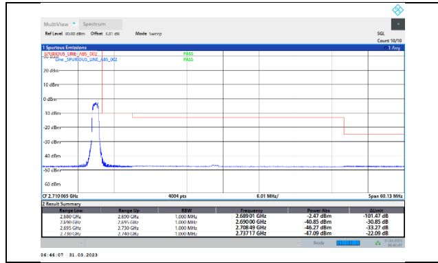
41-41-20MHz-20MHz-QPSK-QPSK-41292-41490-1RB#99-1RB#99
