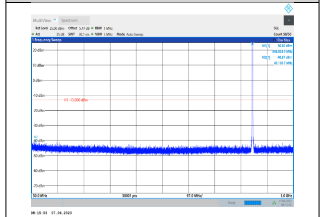
GPRS850-251-30~1000MHz
