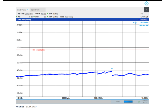
GSM850-190-1000~10000MHz
