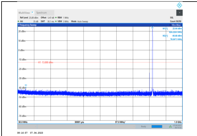
EGPRS850-128-30~1000MHz
