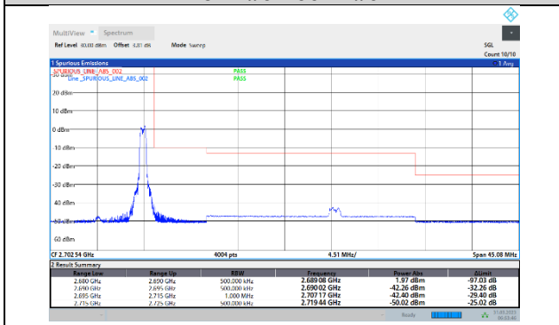
41-41-5MHz-20MHz-QPSK-QPSK-41373-41490-1RB#24-1RB#99
