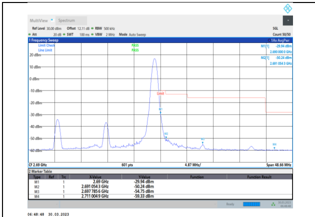
Band41-20MHz-16QAM-41490-1RB#99
