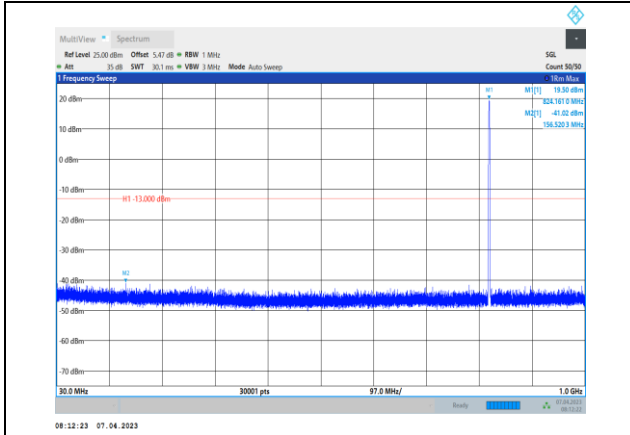
GSM850-128-30~1000MHz
