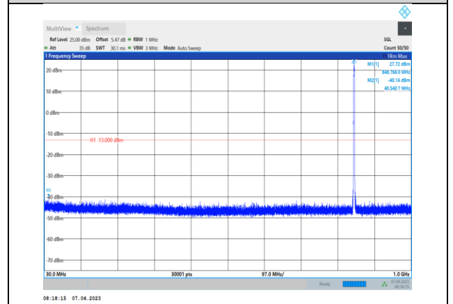
EGPRS850-251-30~1000MHz
