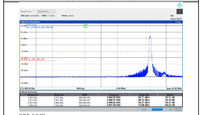
41-41-5MHz-20MHz-QPSK-QPSK-39683-39800-1RB#0-0RB#0
