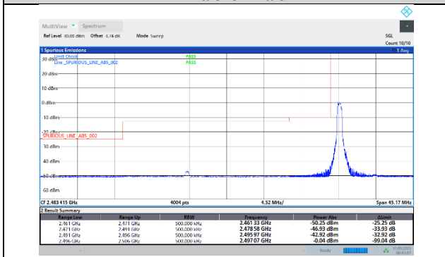
41-41-20MHz-5MHz-QPSK-QPSK-39750-39867-1RB#0-1RB#0
