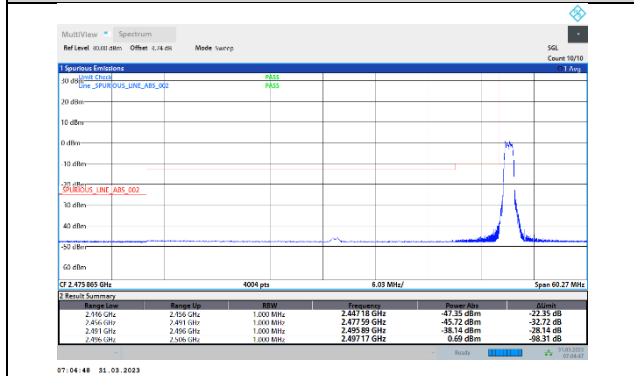
41-41-20MHz-20MHz-QPSK-QPSK-39750-39948-1RB#0-1RB#0
