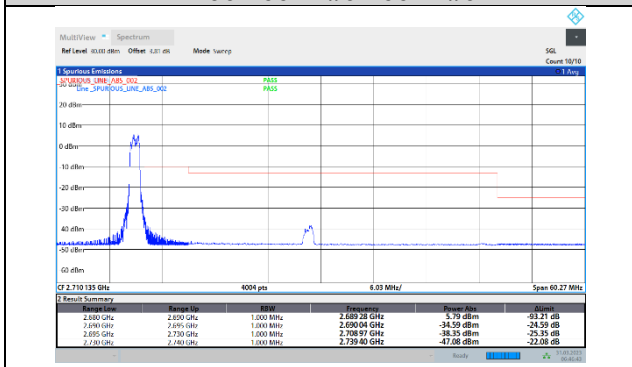
41-41-20MHz-20MHz-16QAM-16QAM-41292-41490-1RB#99-1RB#99
