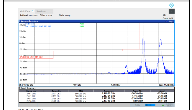
41-41-5MHz-20MHz-QPSK-QPSK-39683-39800-1RB#0-1RB#0
