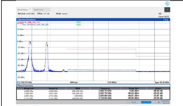
41-41-20MHz-5MHz-QPSK-QPSK-41440-41557-1RB#99-1RB#24
