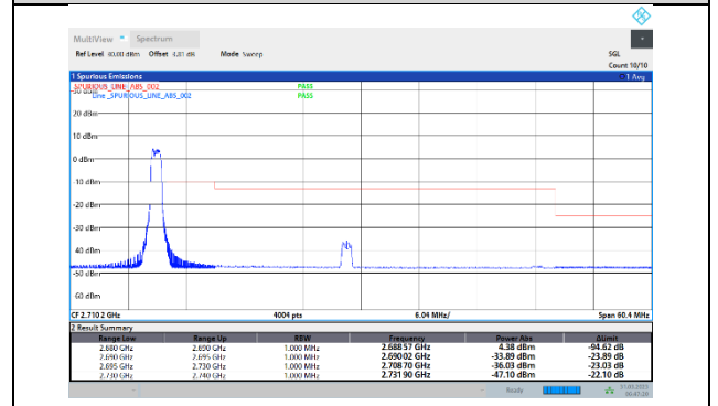
41-41-20MHz-20MHz-64QAM-64QAM-41292-41490-1RB#99-1RB#99
