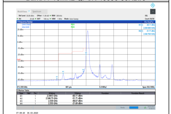
Band41-10MHz-QPSK-40290-1RB#0
