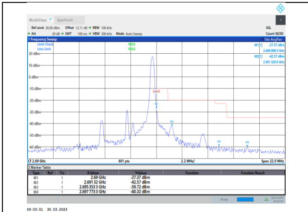
Band41-5MHz-16QAM-41565-1RB#24
