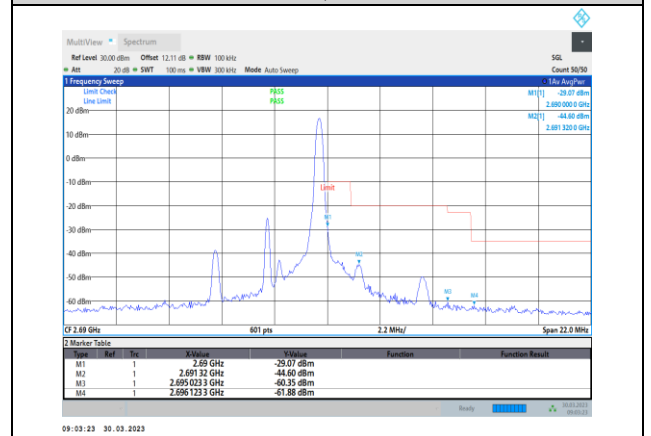
Band41-5MHz-64QAM-41565-1RB#24
