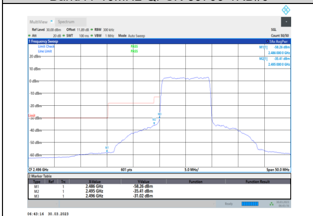
Band41-10MHz-QPSK-39700-50RB#0
