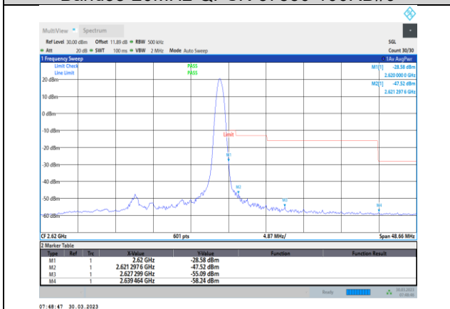
Band38-20MHz-QPSK-38150-1RB#99
