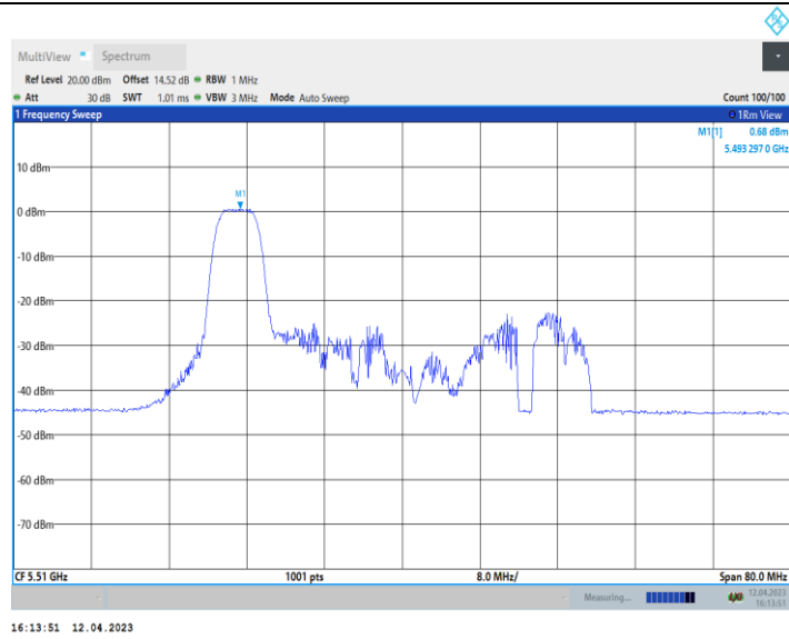
11AX40_Ant10_5510_242Tone_RU61
