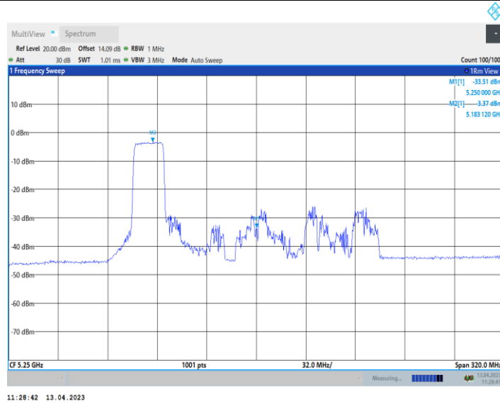
11AX160_Ant9_5250_UNII-1_484Tone_RU65
