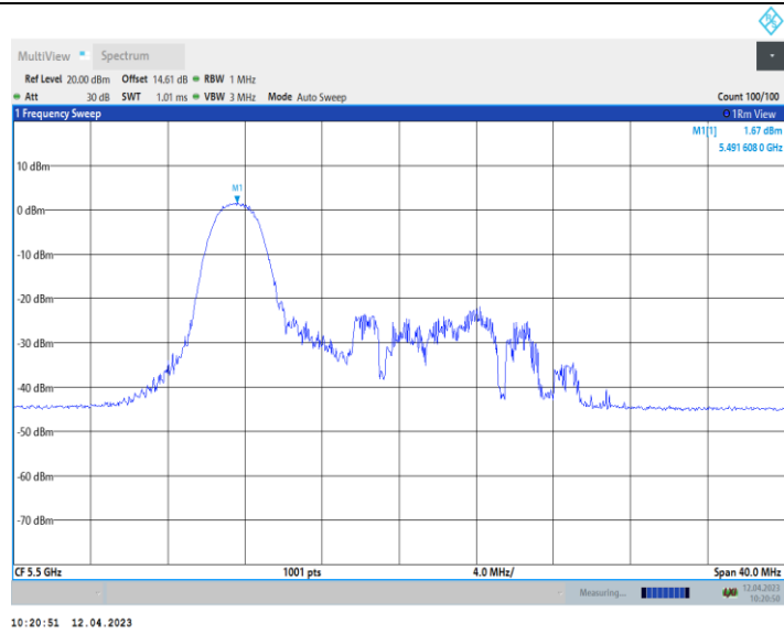
11AX20_Ant10_5500_52Tone_RU37
