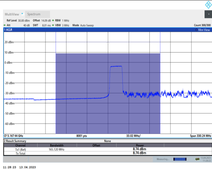
11AX160_Ant9_5250_UNII-1_484Tone_RU65
