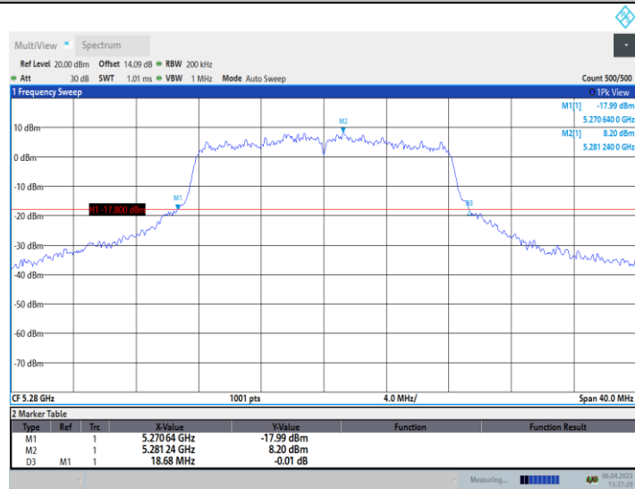
11A_Ant10_5280
