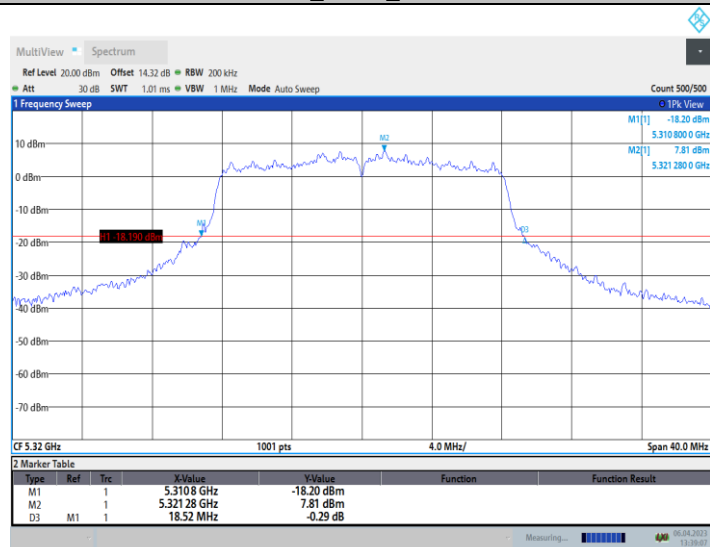
11A_Ant10_5320
