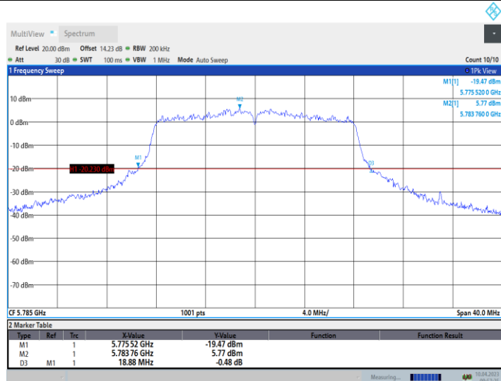
11A_Ant10_5785
